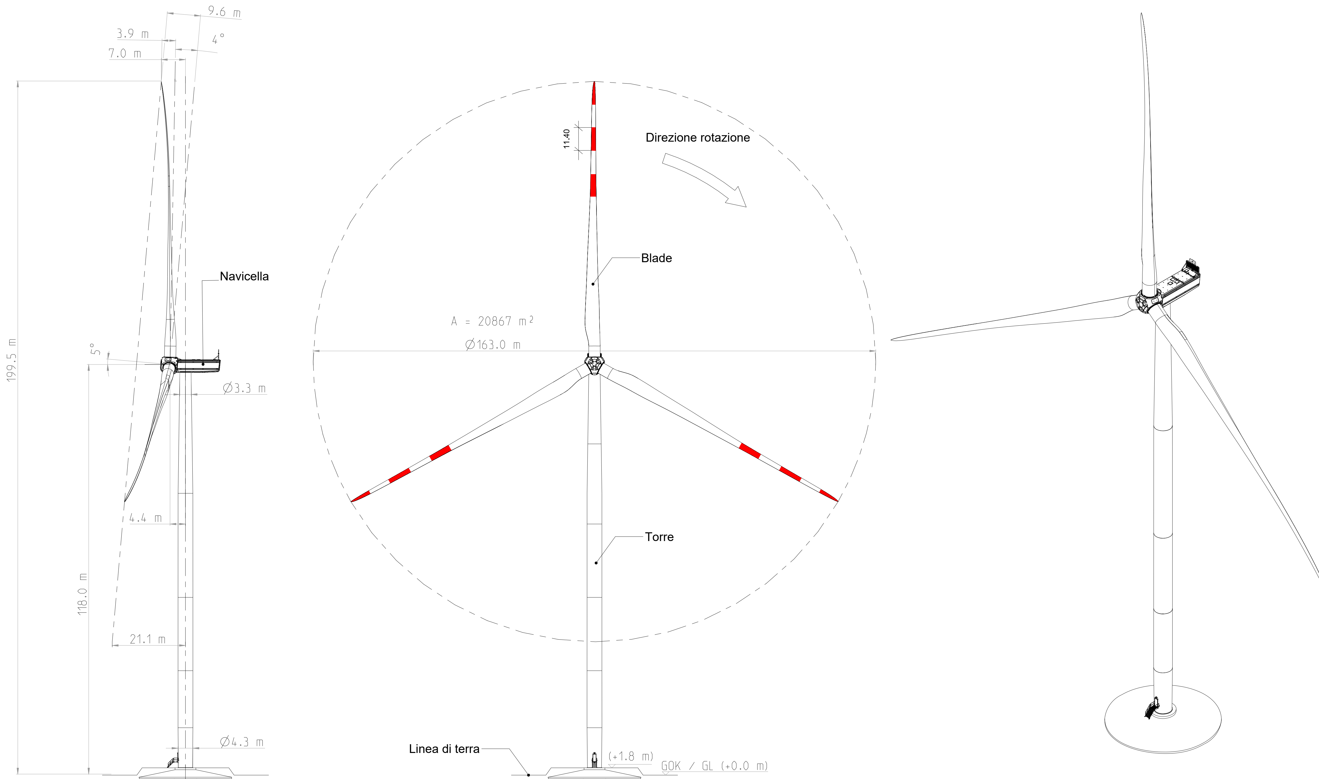
AEROGENERATORE TIPO DI PROGETTO - NORDEX 163
