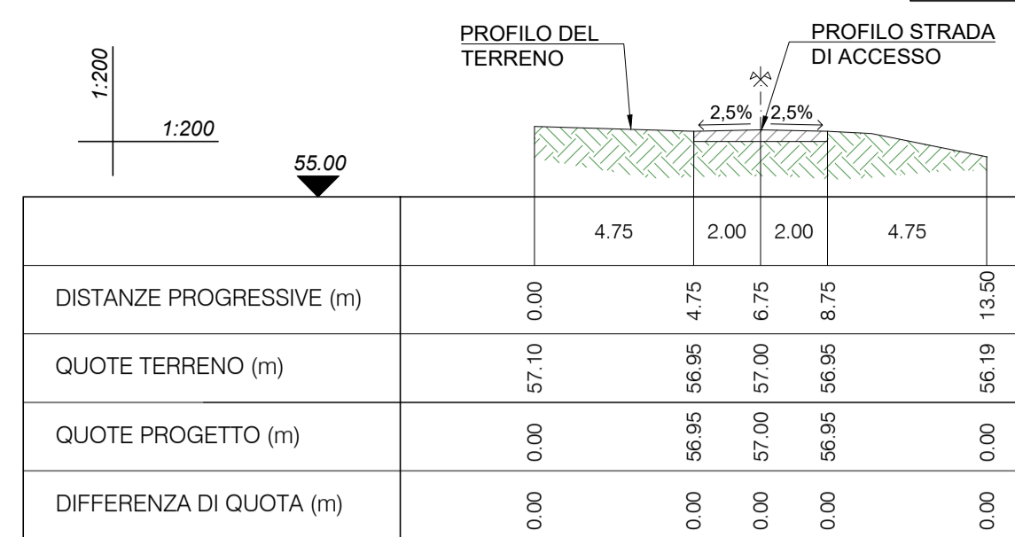
SEZIONE 3-3 PROGR. 151.98
