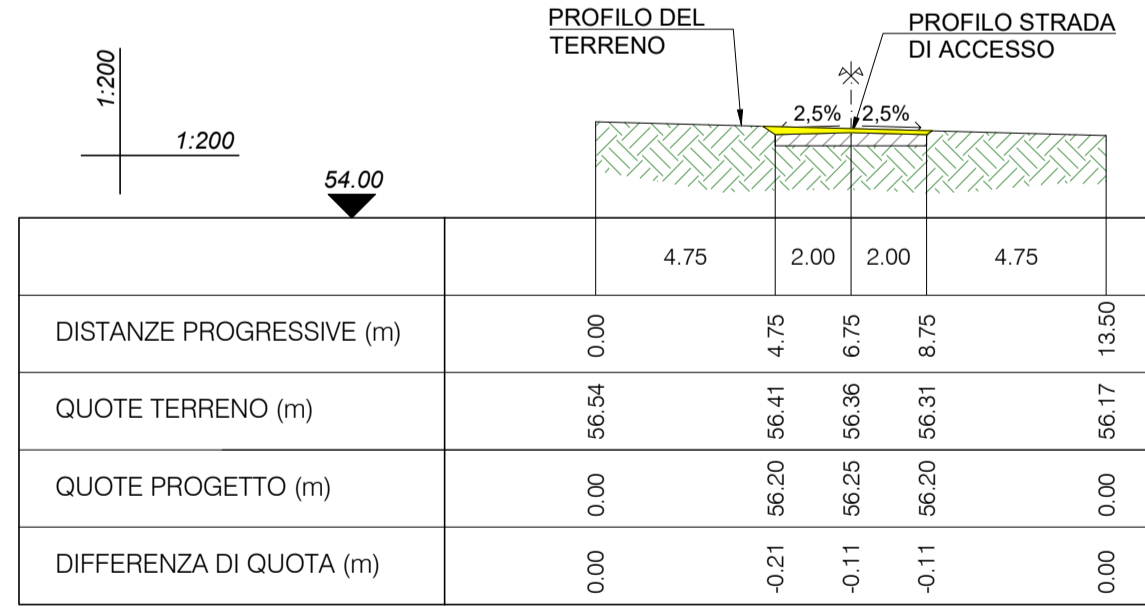
SEZIONE 12-12 PROGR. 488.31
