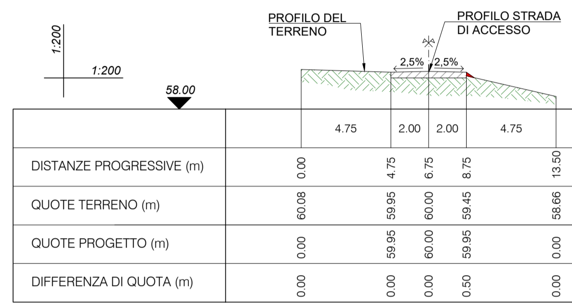
SEZIONE 7-7 PROGR. 300.00
