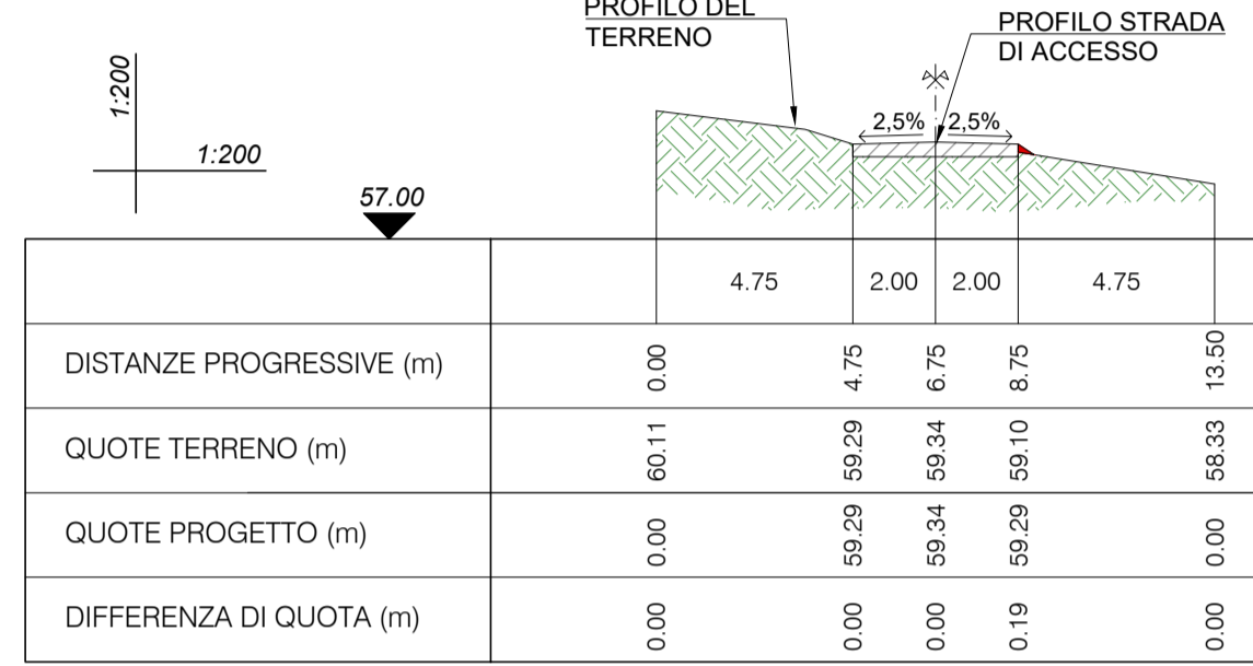
SEZIONE 6-6 PROGR. 248.76
