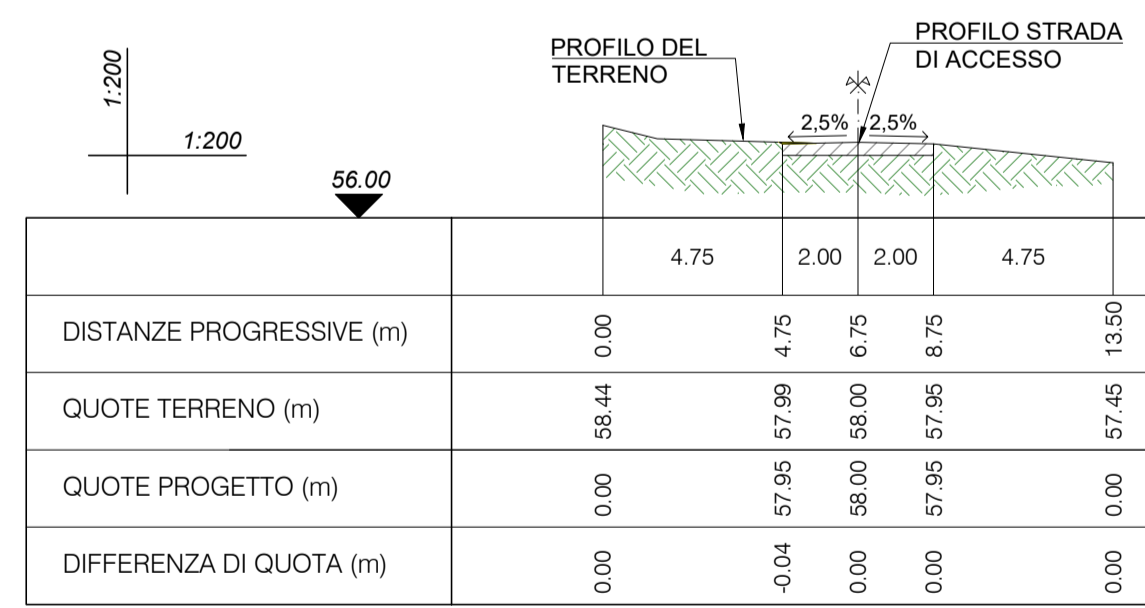
SEZIONE 14-14 PROGR. 550.00
