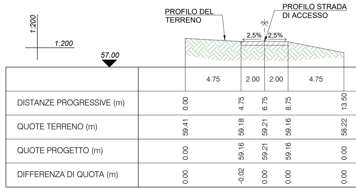
SEZIONE 15-15 PROGR. 600.00
