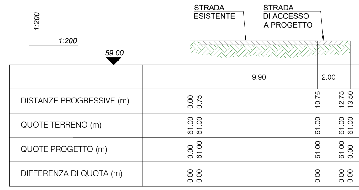
SEZIONE 17-17 PROGR. 675.00
