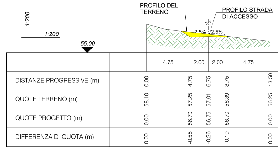
SEZIONE 11-11 PROGR. 450.00
