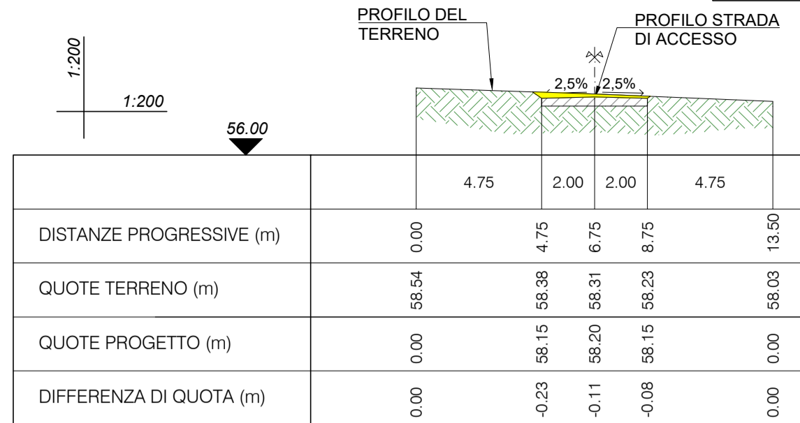
SEZIONE 1-1 PROGR. 50.00
