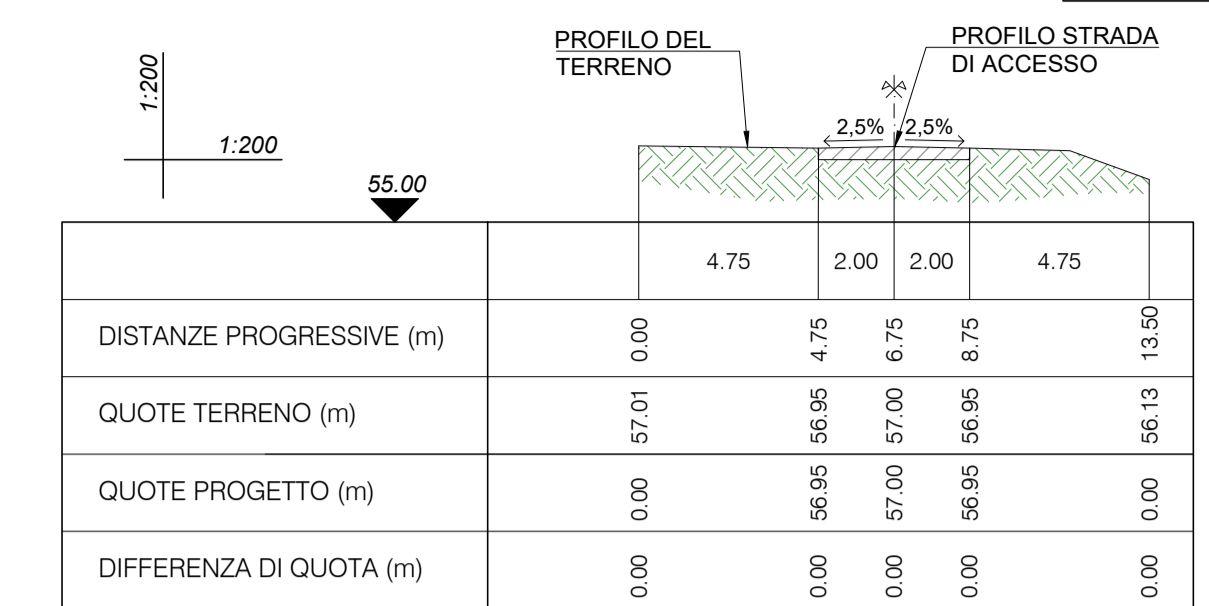
SEZIONE 4-4 PROGR. 164.22
