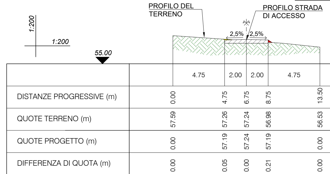
SEZIONE 2-2 PROGR. 100.00
