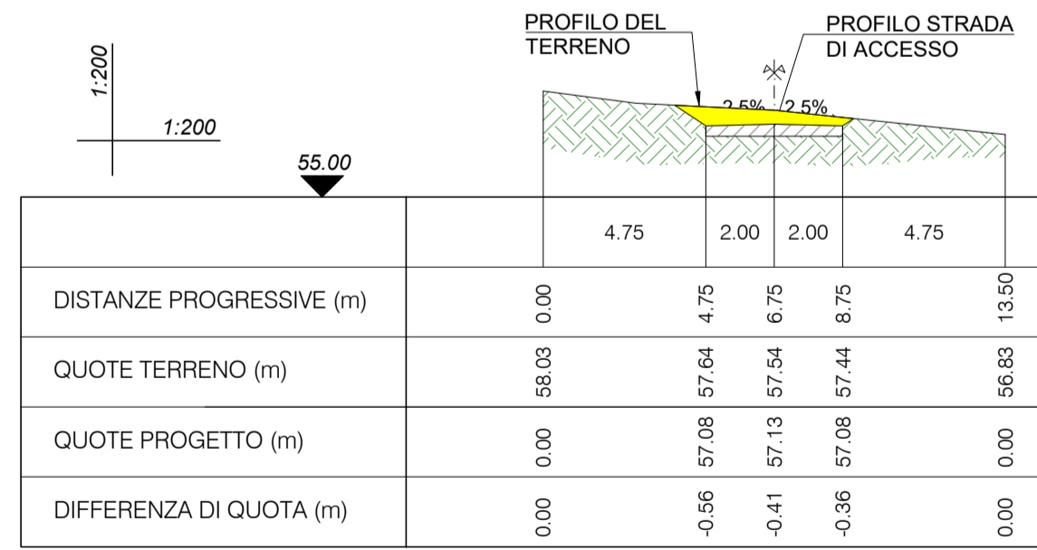
SEZIONE 13-13 PROGR. 500.00
