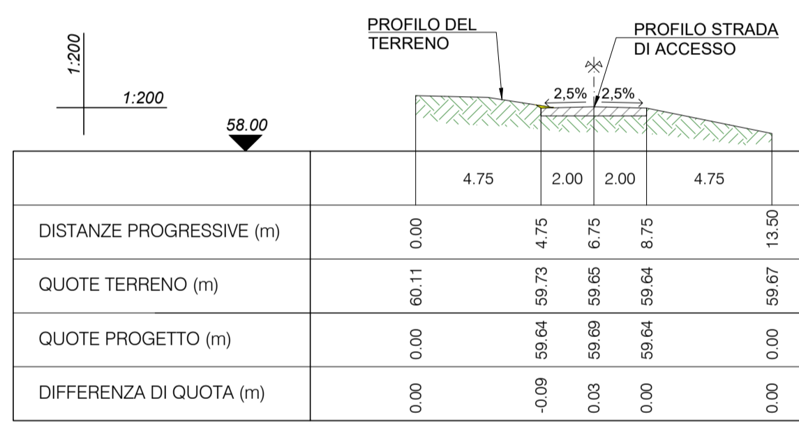
SEZIONE 9-9 PROGR. 400.00
