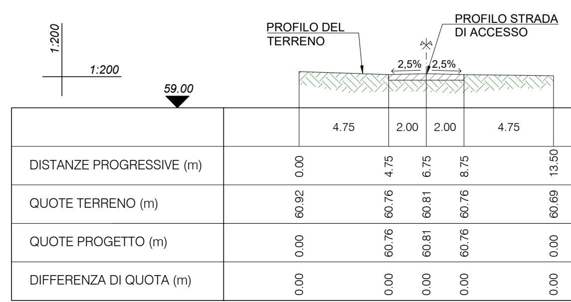
SEZIONE 16-16 PROGR. 650.00
