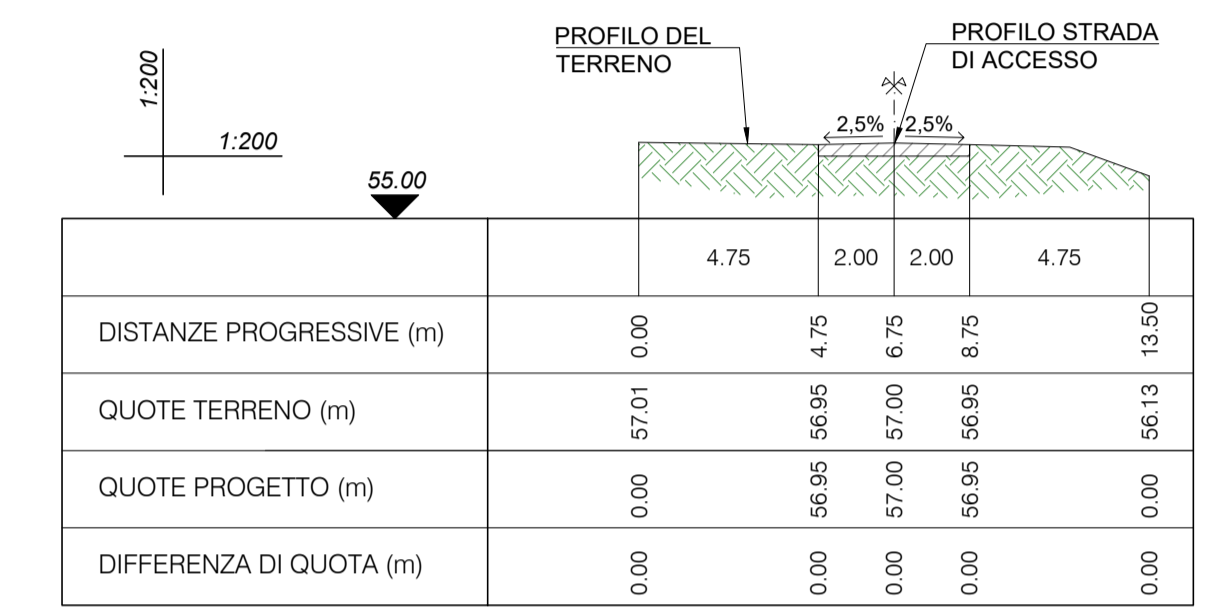
SEZIONE 8-8 PROGR. 339.42
