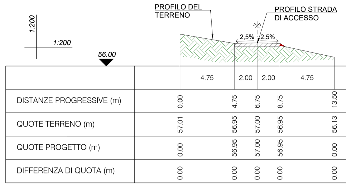
SEZIONE 5-5 PROGR. 200.00
