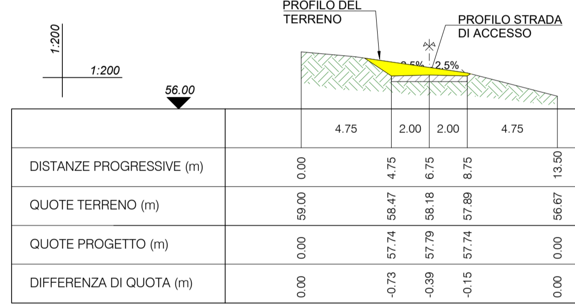
SEZIONE 10-10 PROGR. 435.22
