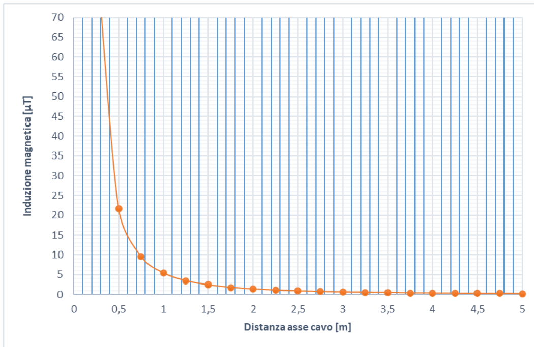
Figura 4. Andamento dell'induzione magnetica con la distanza dal cavo AT
