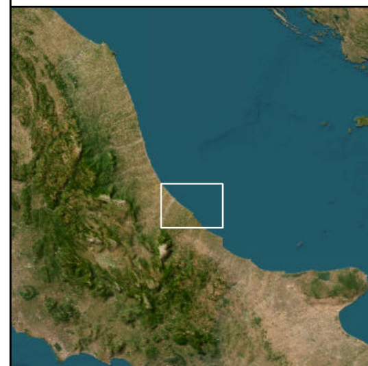
INTENSITA' TRAFFICO MARITTIMO - ALTRE IMBARCAZIONI
