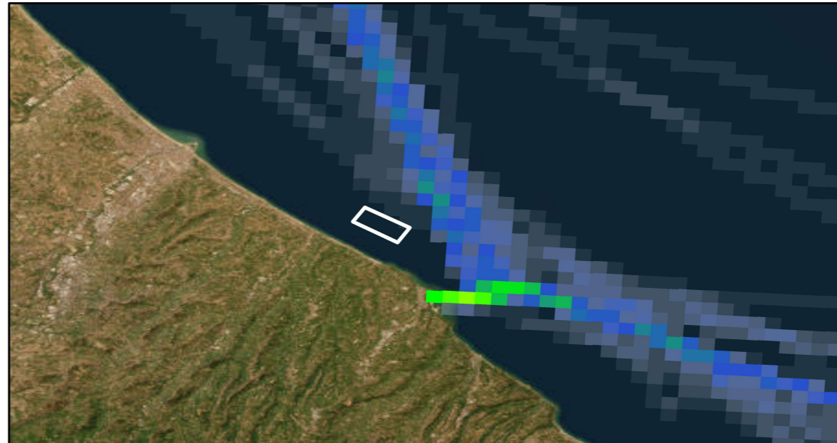
INTENSITA' TRAFFICO MARITTIMO - PASSEGGERI
