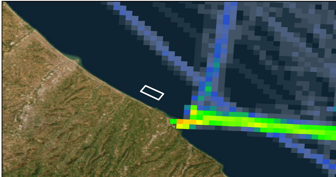
INTENSITA' TRAFFICO MARITTIMO - PETROLIERE
