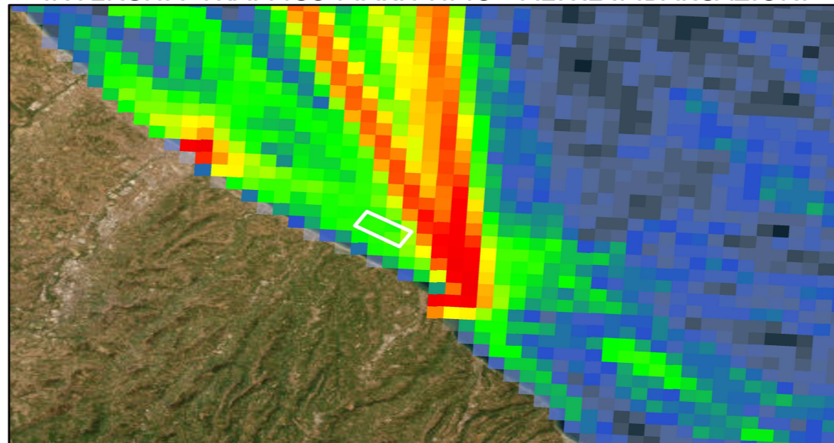
INTENSITA' TRAFFICO MARITTIMO - ALTRE IMBARCAZIONI
