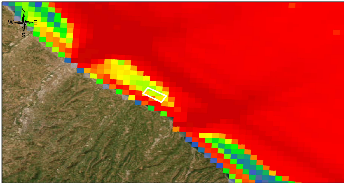
INTENSITA' TRAFFICO MARITTIMO - TOTALE
