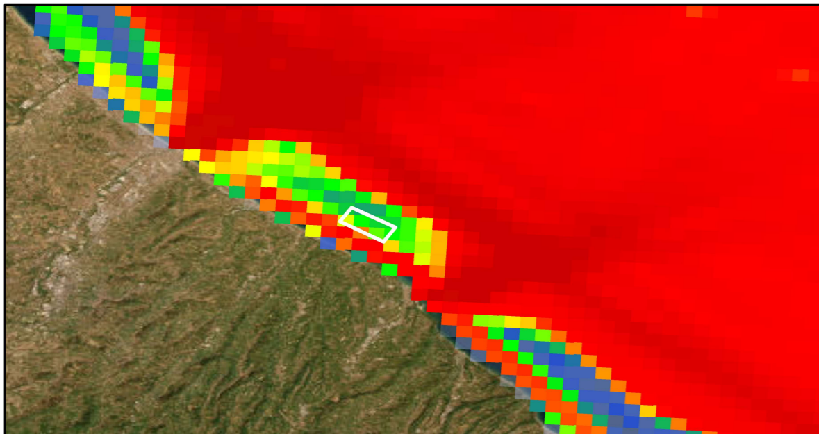
INTENSITA' TRAFFICO MARITTIMO - PESCA
