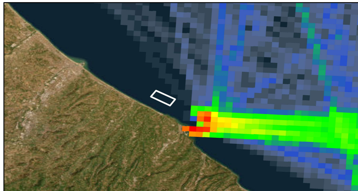
INTENSITA' TRAFFICO MARITTIMO - MERCANTILE
