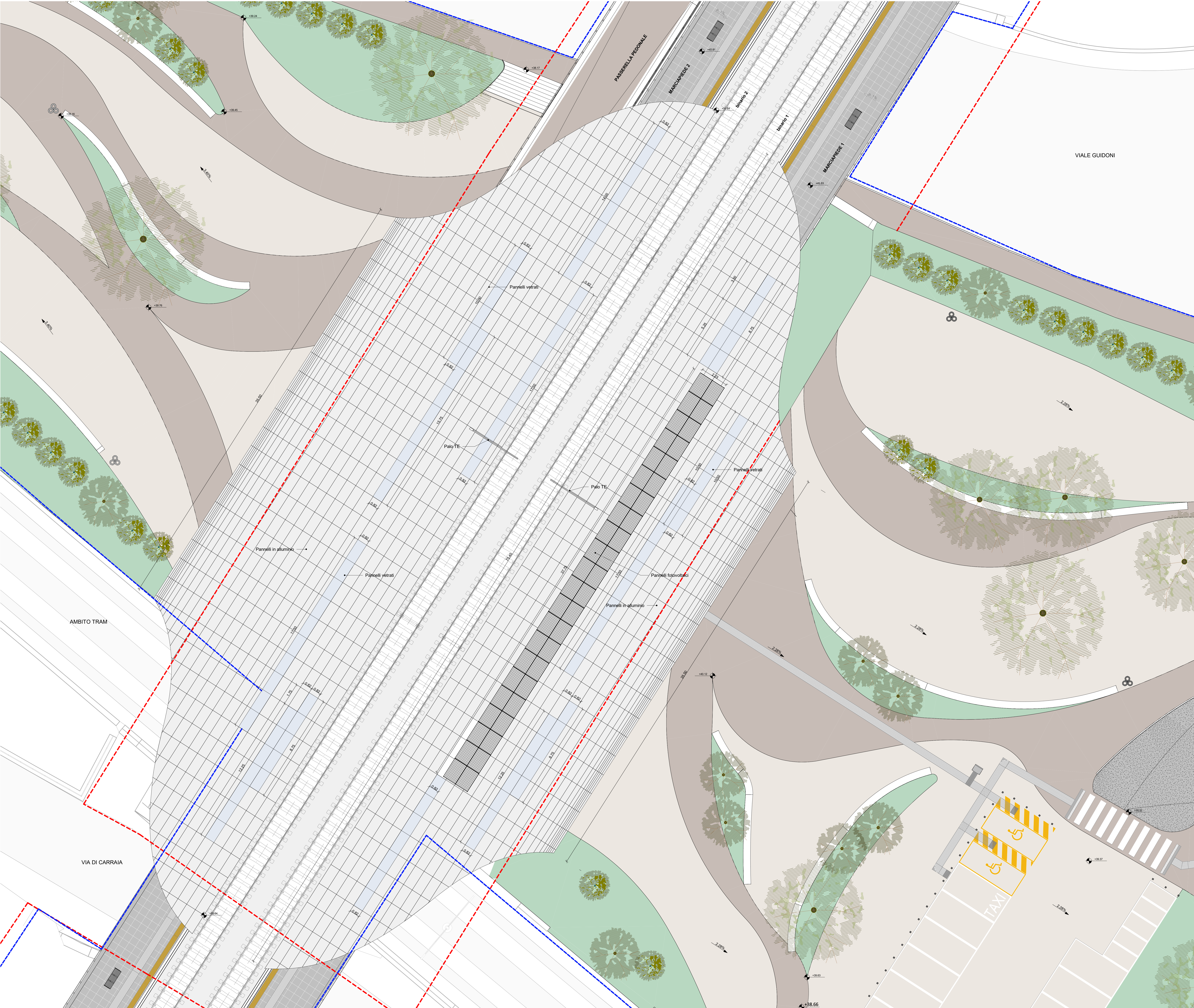
MARCIAPIEDI - PIANTE DELLE PENSILINE 1:100
