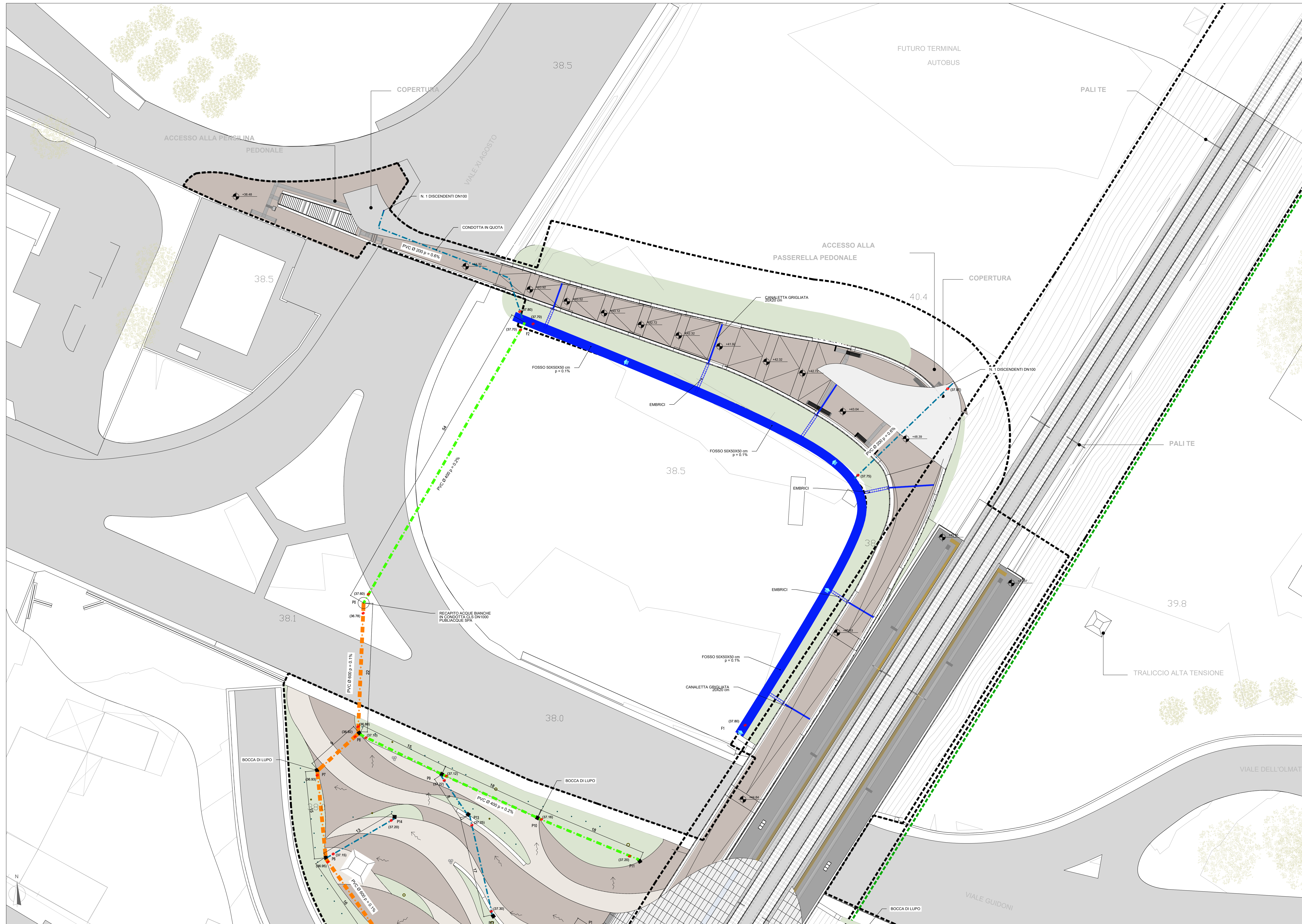
PLANIMETRIA PASSERELLA 1 : 200
