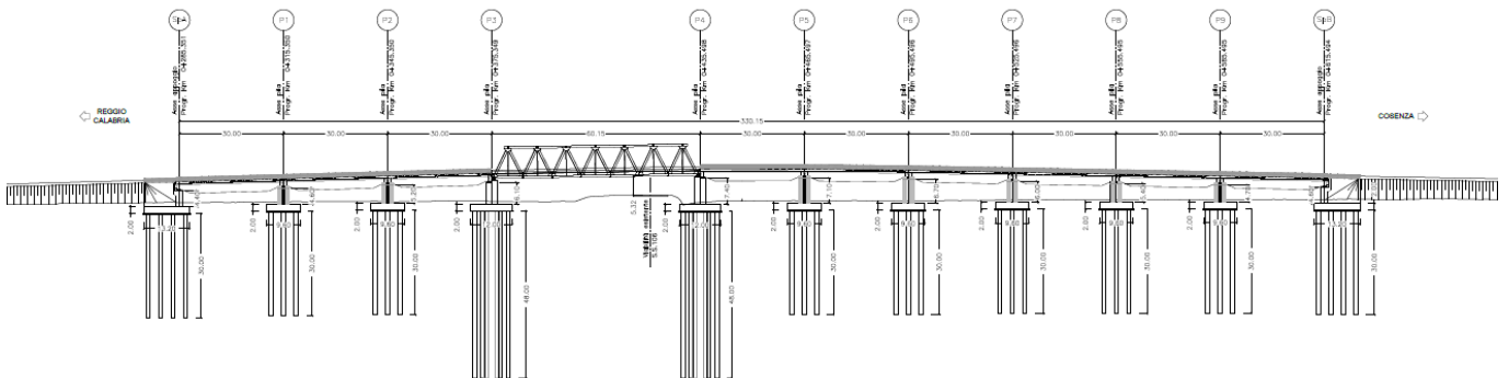
Figura 14 – Prospetto VI01
