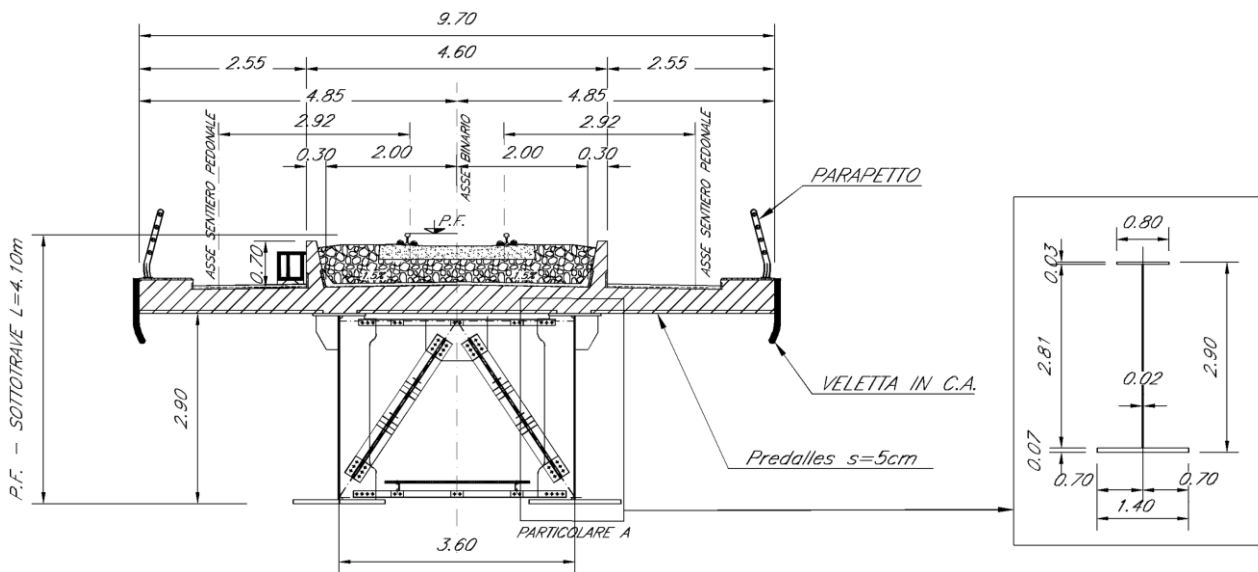
Figura 15. Sezione trasversale impalcato per campate da 30 m
