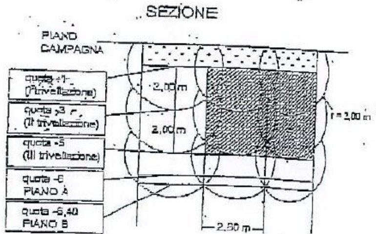
Figura 28 Schemi generali di bonifica ordigni esplosivi profonda
