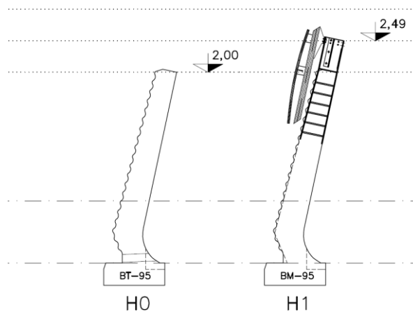
Fig. 93 – Tipologico BA “HS”
