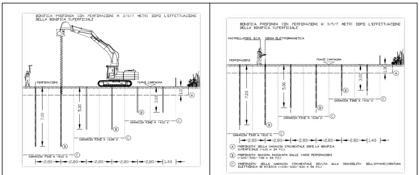
Figura 27 Schemi generali di bonifica ordigni esplosivi profonda
