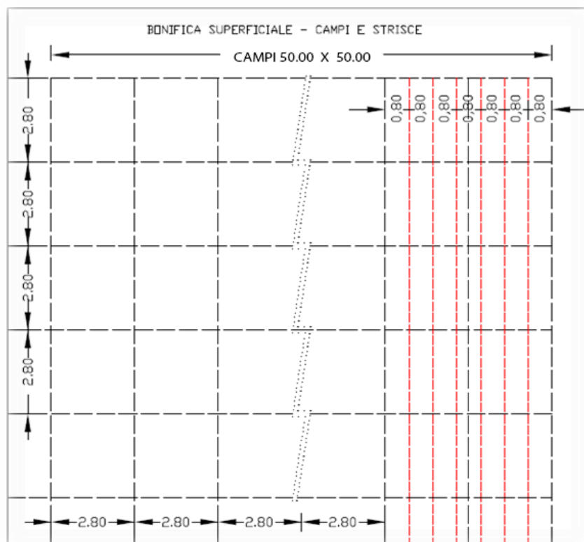
Figura 25 Maglia bonifica superficiale
