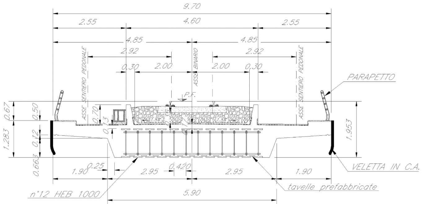
Figura 23. Sezione trasversale impalcato VI02
