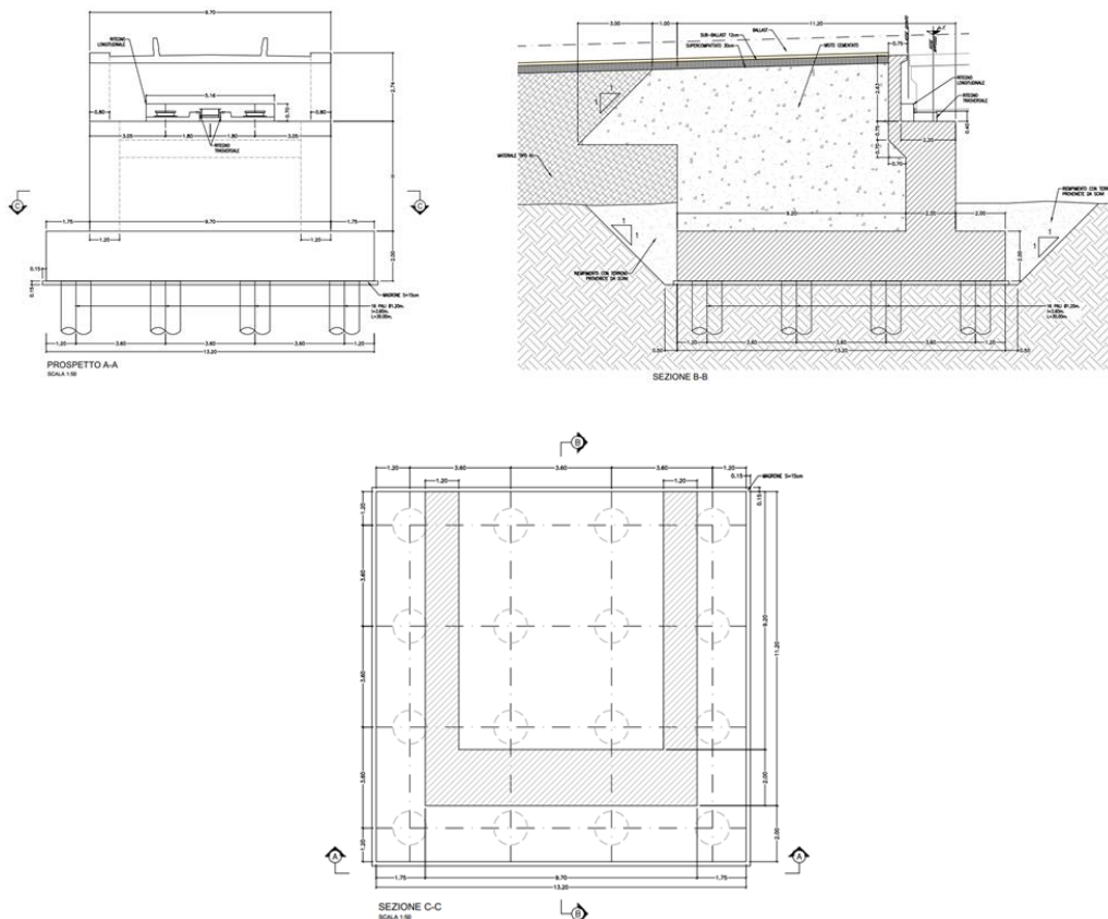
Figura 20 – Prospetto e sezioni spalle [m]
