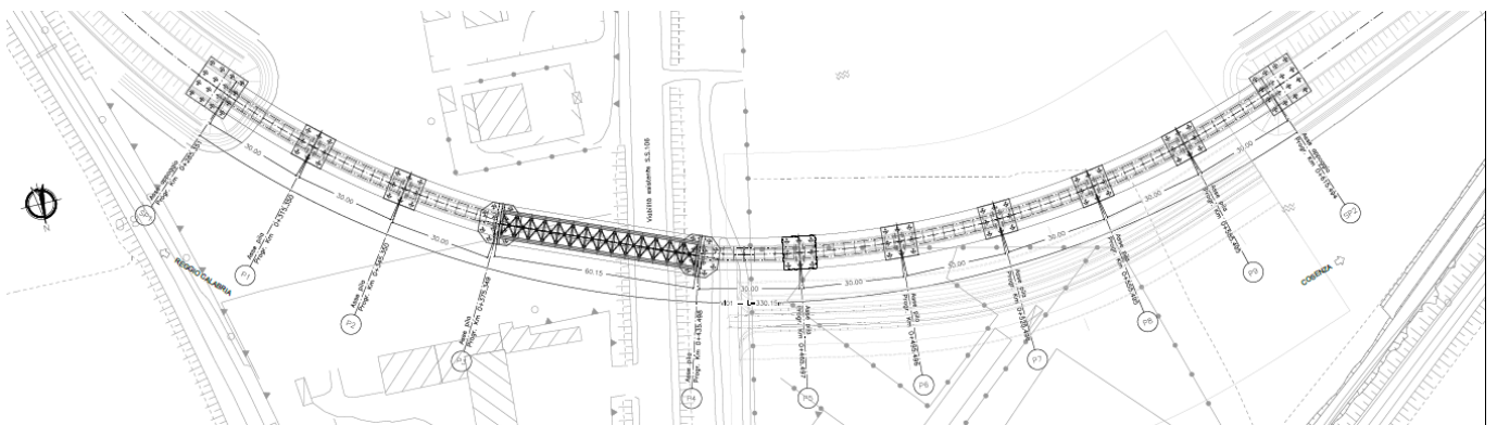
Figura 13 – Vista planimetrica VI01
