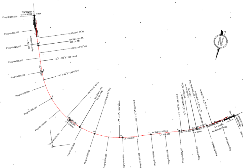
Figura 5 – Planimetria di tracciamento
