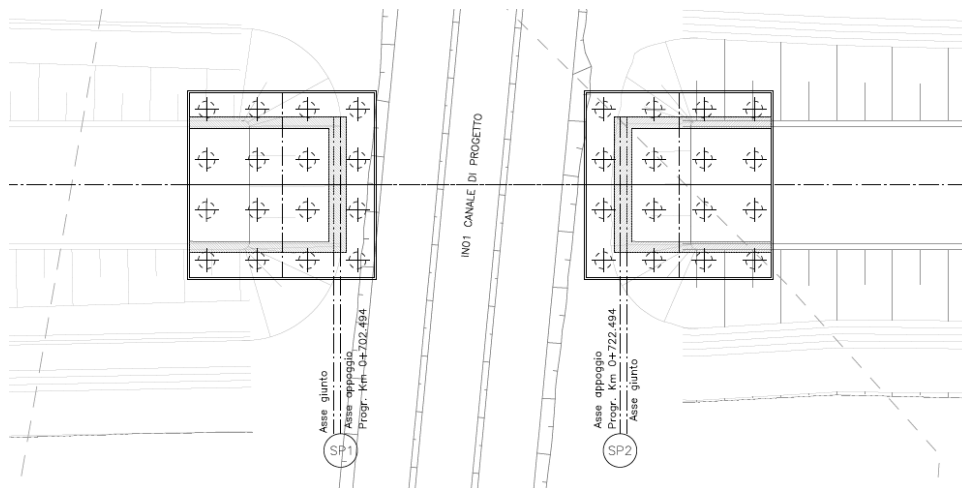
Figura 21 – Vista planimetrica VI02
