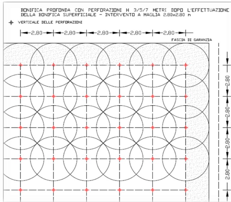
Figura 26 Schema planimetrico maglia perforazioni bonifica profonda
