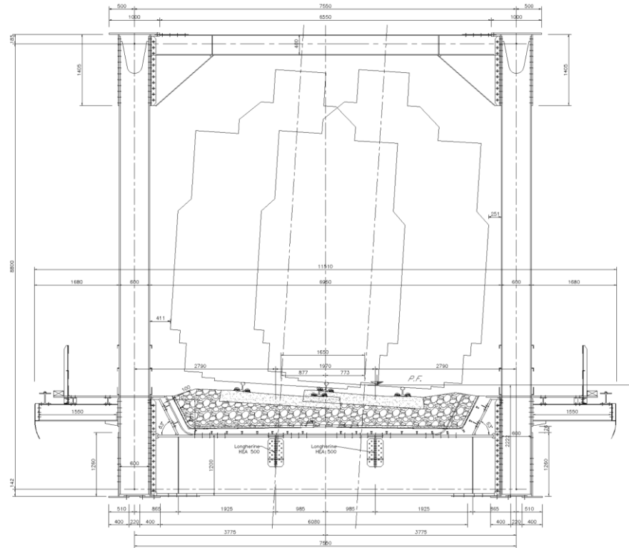
Figura 16 – Sezione trasversale impalcato per campata da 60 m
