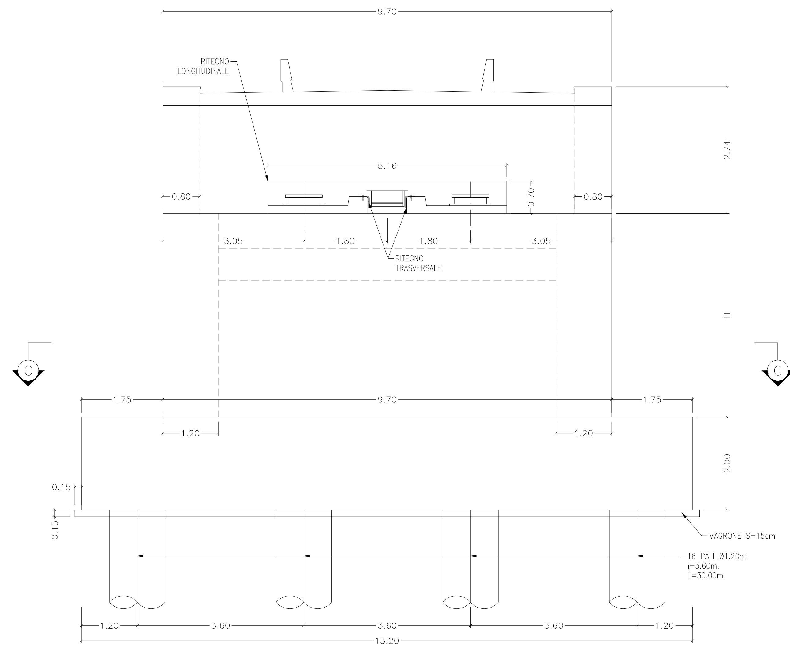
PROSPETTO A-A SCALA 1:50
