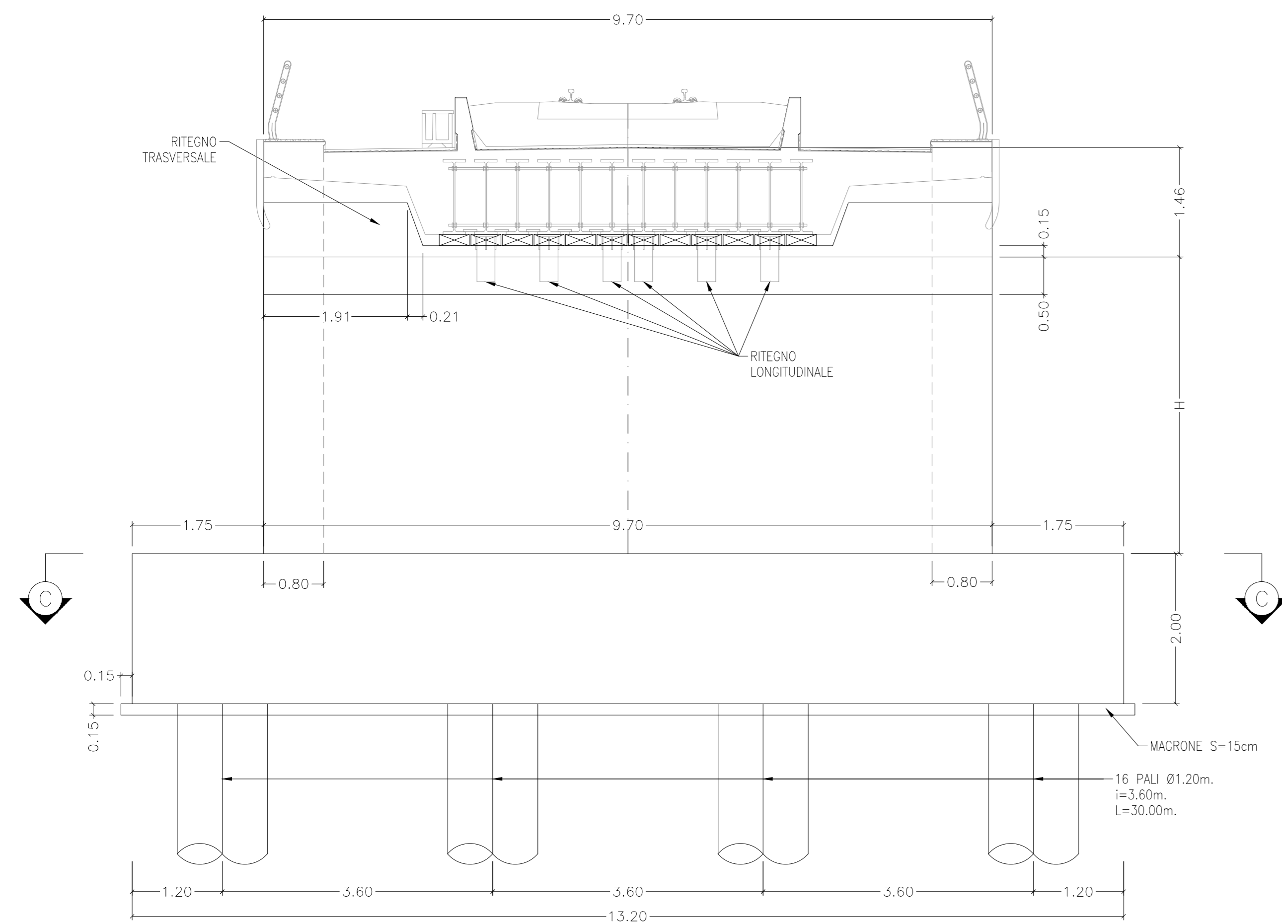
PROSPETTO A-A SCALA 1:50
