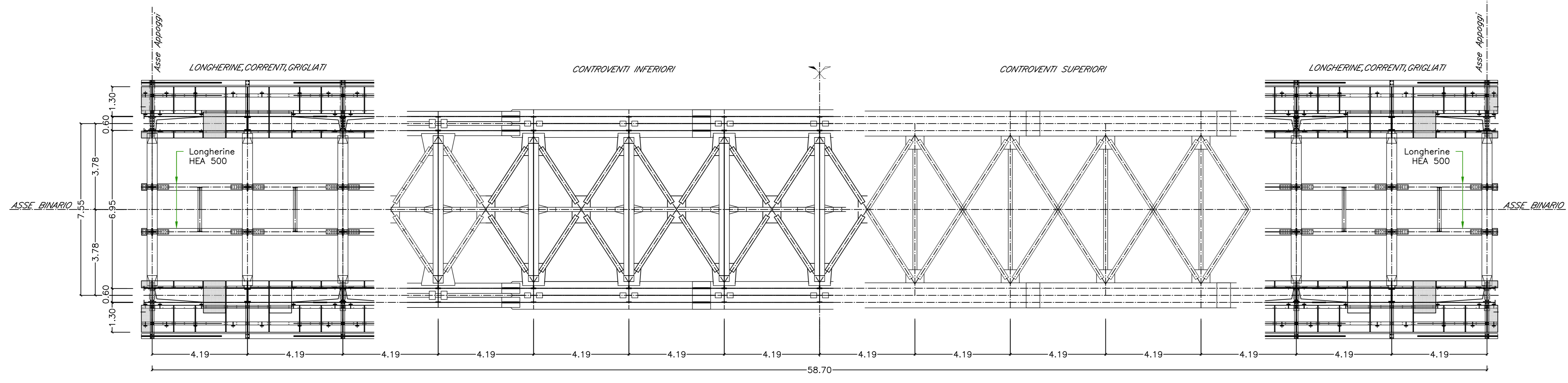
PIANTA L=60m SINGOLO BINARIO SCALA 1:100
