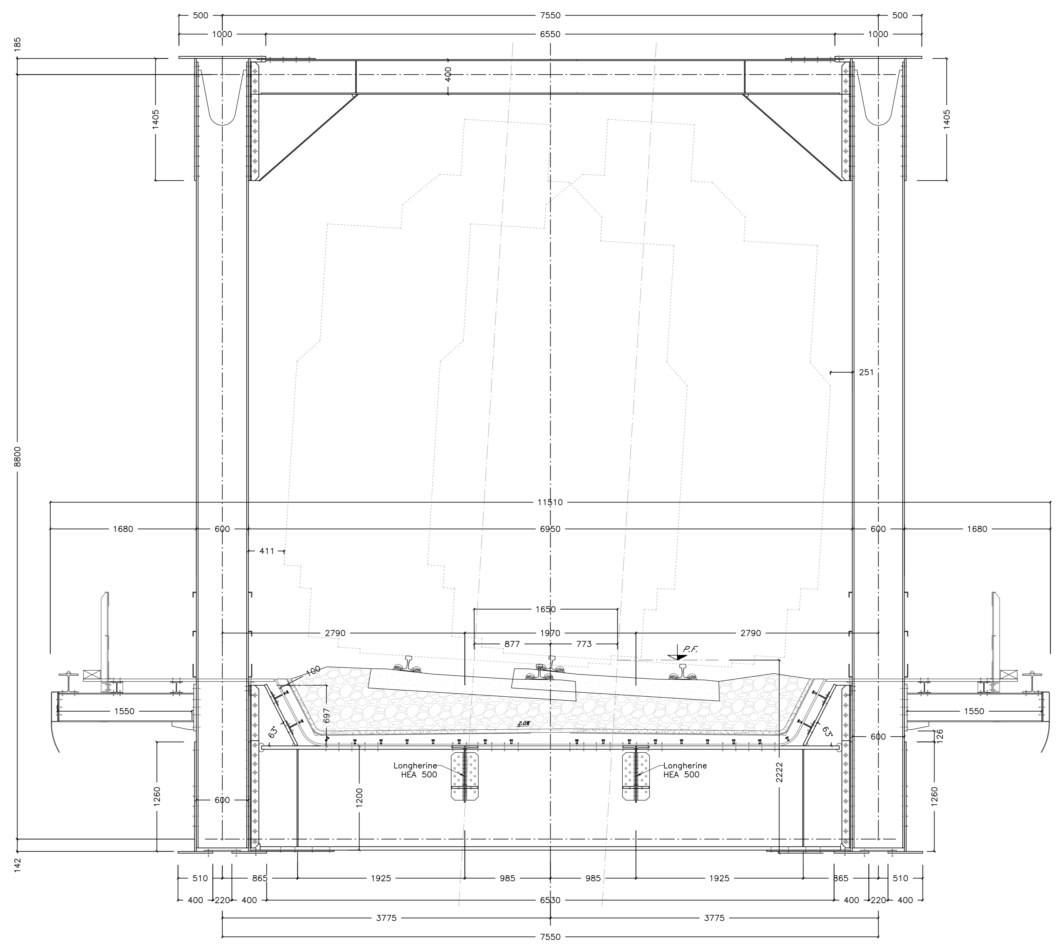
SEZIONE TRASVERSALE L=60m SINGOLO BINARIO SCALA 1:25
