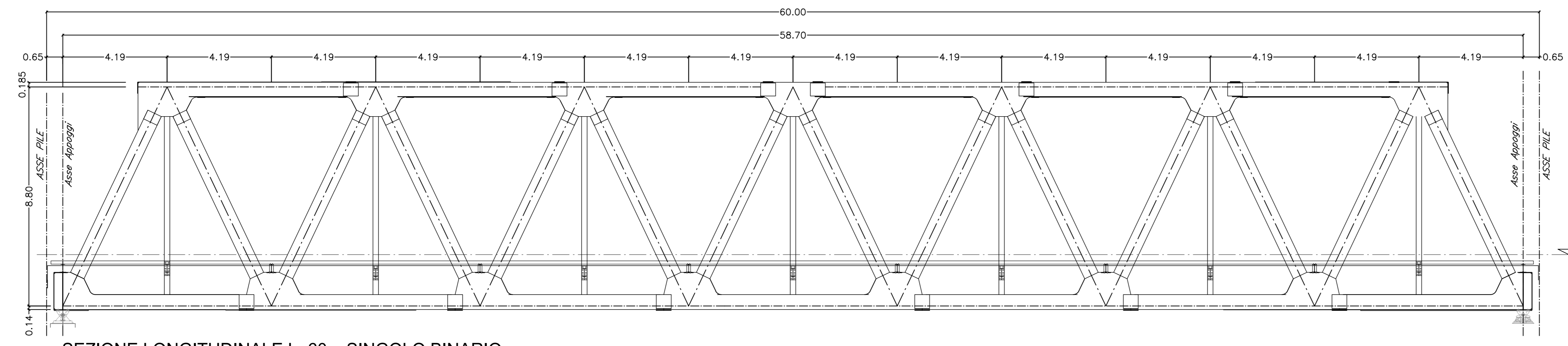
SEZIONE LONGITUDINALE L=60m SINGOLO BINARIO SCALA 1:100
