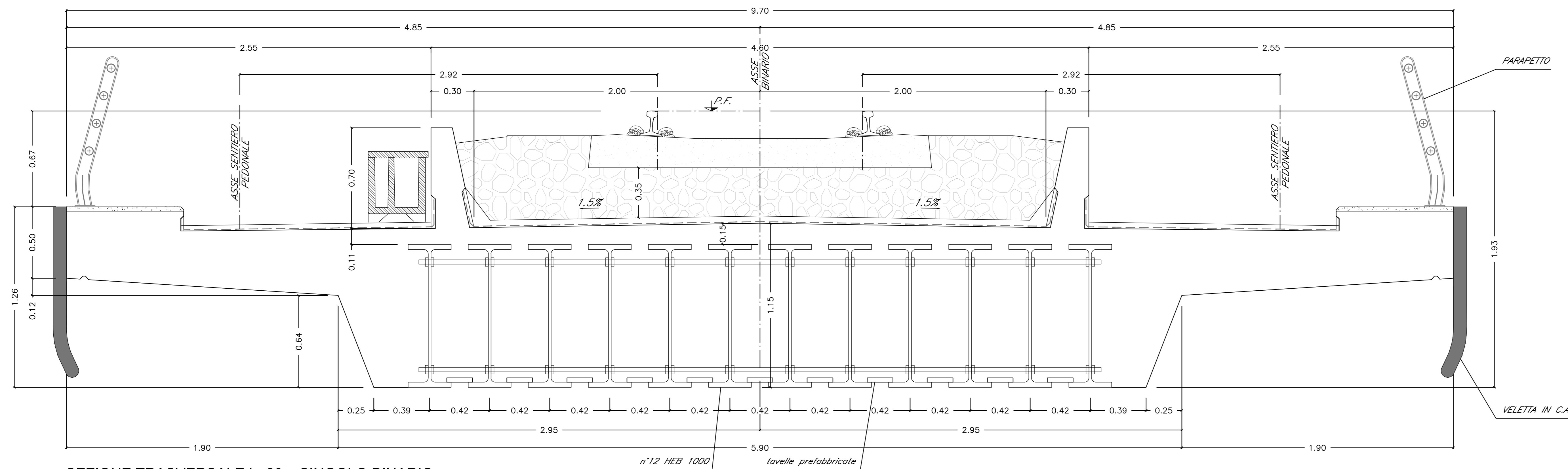
SEZIONE TRASVERSALE L=20m SINGOLO BINARIO SCALA 1:15
