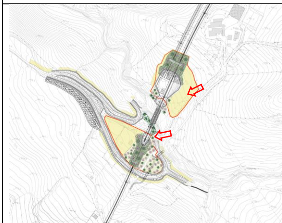
IA02 – Viadotto VI01 e imbocco galleria GN01 Lato Catania e imbocco galleria GN02 Lato Palermo
