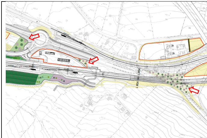
IA01 – Stazione Nuova Enna
