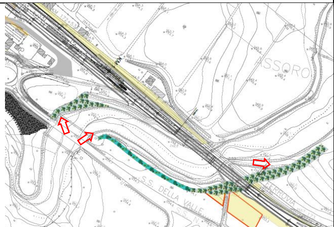
IA06 – Imbocco stazione Dittaino Lato Catania
