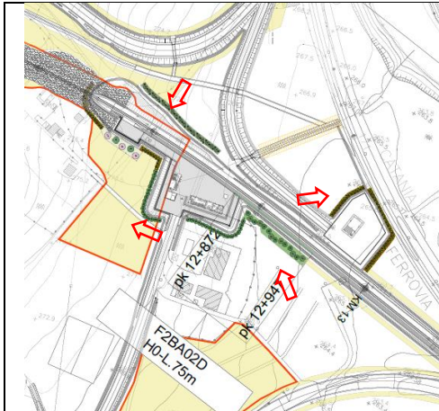
IA05 – Imbocco galleria GN03 Lato Catania
