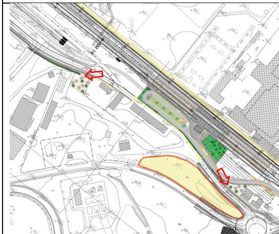
IA06 – Stazione Dittaino
