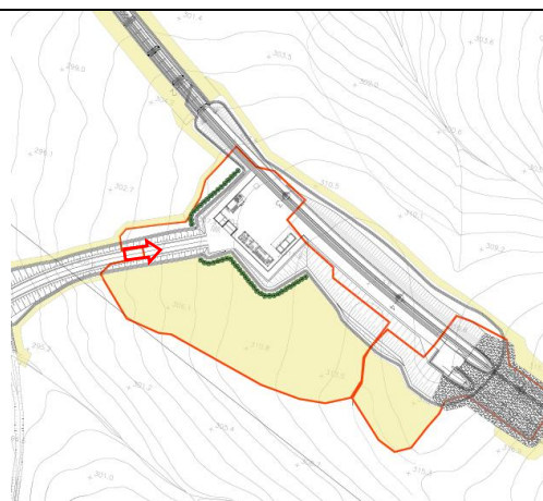
IA04 – Imbocco galleria GN03 Lato Palermo
