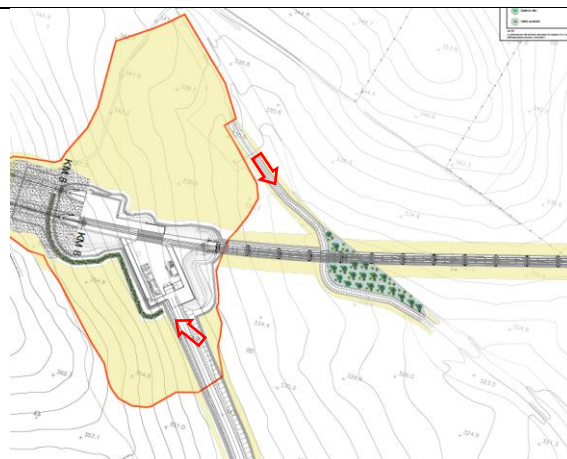
IA03 – Imbocco galleria GN02 Lato Catania
