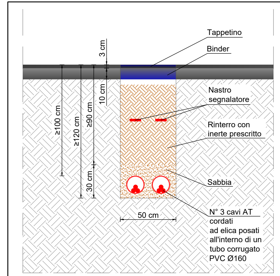
Sezione tipo attraversamento canale
