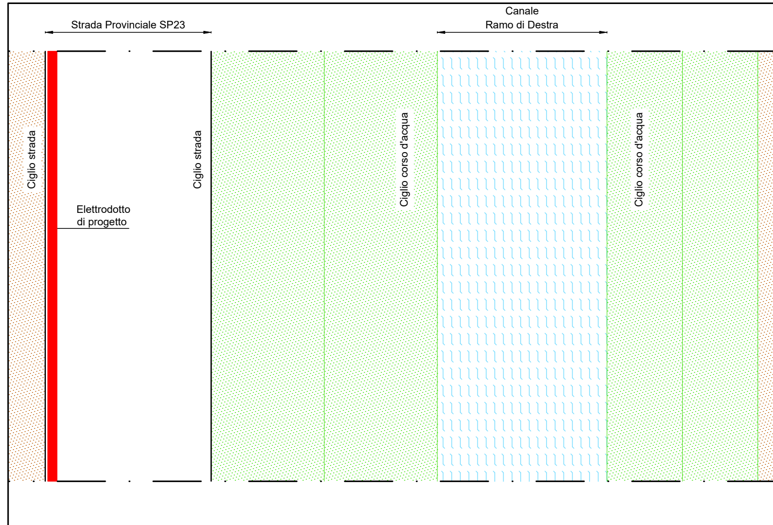
Fiancheggiamento canale Ramo di Destra lungo la Strada Provinciale SP23 Scala 1:100
