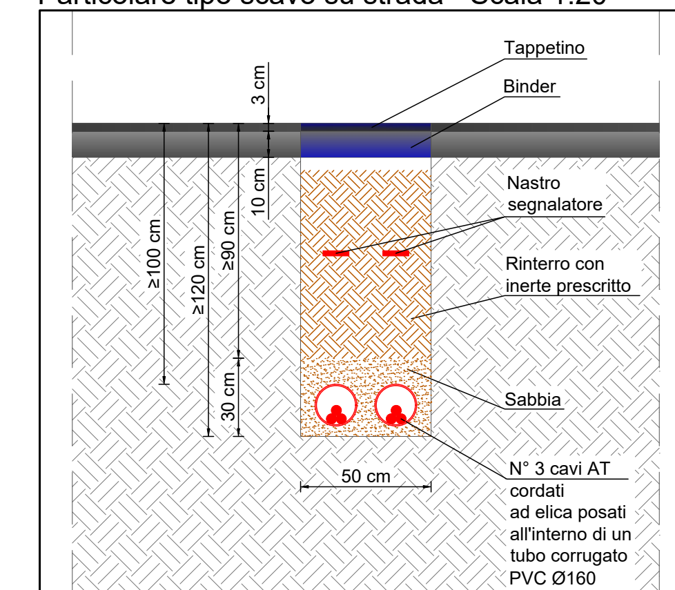
Particolare tipo scavo su strada - Scala 1:20
