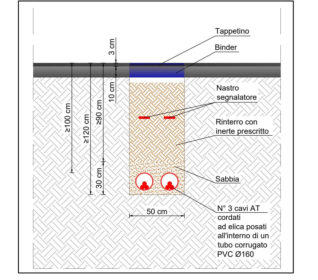
Particolare tipo scavo su strada Scala 1:20
