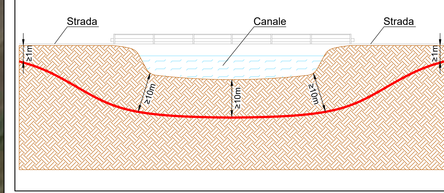
Sezione tipo attraversamento canale mediante TOC (NO DIG)
