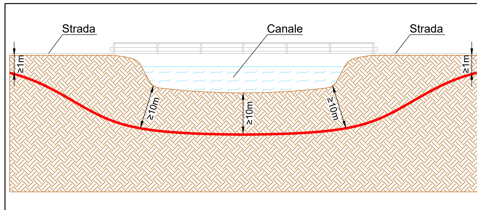
Sezione tipo attraversamento canale
