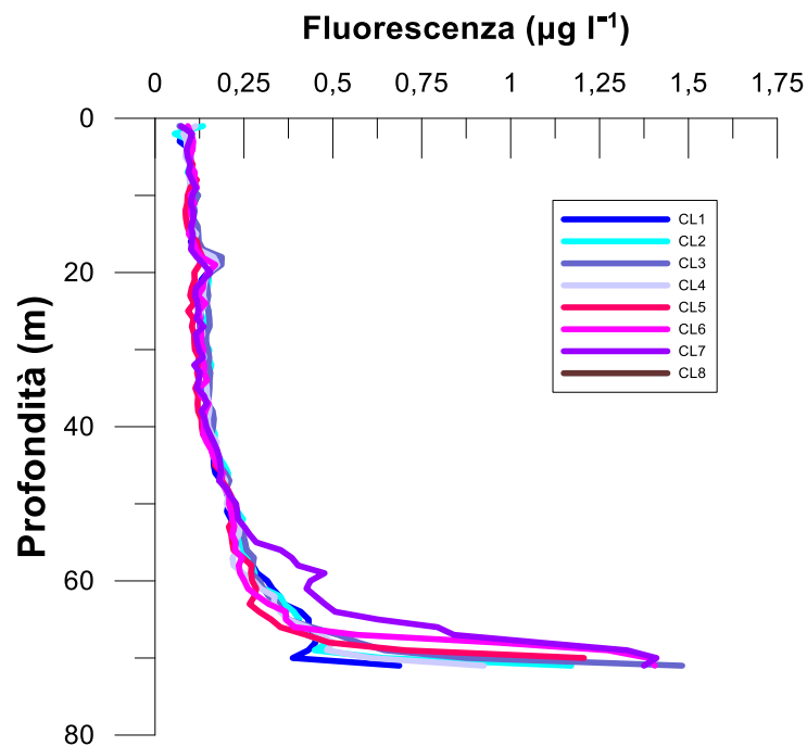
Fig. 3.9 - Profili di fluorescenza ( \mu\text{g L}^{-1} ). Campagna di Luglio 2022 .
