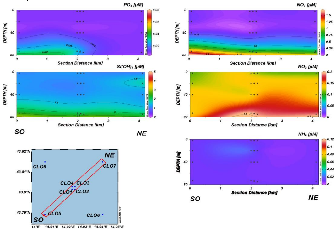
Fig. 3.24b - Sezioni SO-NE delle stazioni CL5, CL1, CL2, CL4, CL3 e CL7 rappresentanti le concentrazioni di fosfati ( PO_4 ), silicati ( Si(OH)_4 ), nitrati ( NO_3 ), nitriti ( NO_2 ) e ammonio ( NH_4 ) in \mu M . Dicembre 2022.
