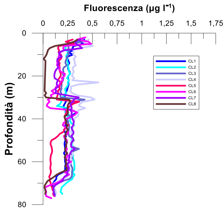
Fig. 3.15 - Profili di fluorescenza ( \mu\text{g L}^{-1} ). Campagna di Dicembre 2022 .
