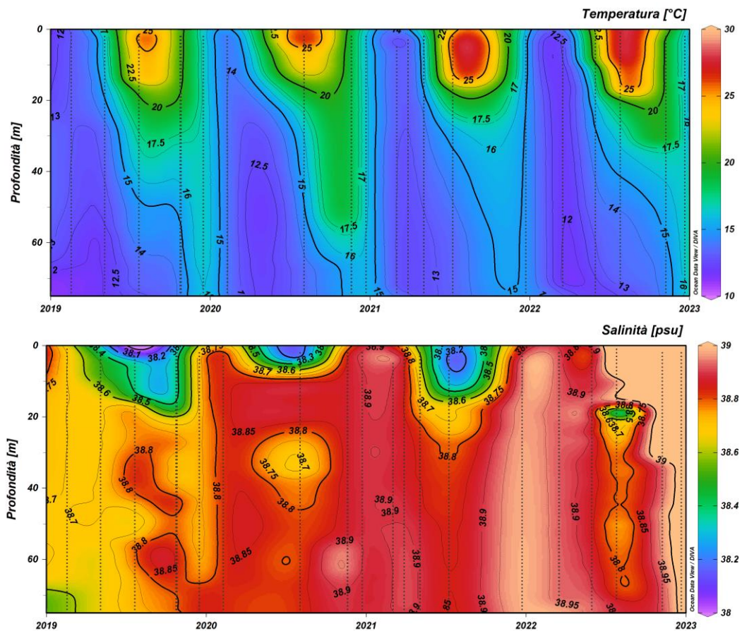
Fig. 3.36 - Andamento annuale della temperatura (°C) e della salinità (psu) per la piattaforma Clara NW (da febbraio 2019 a dicembre 2022).
