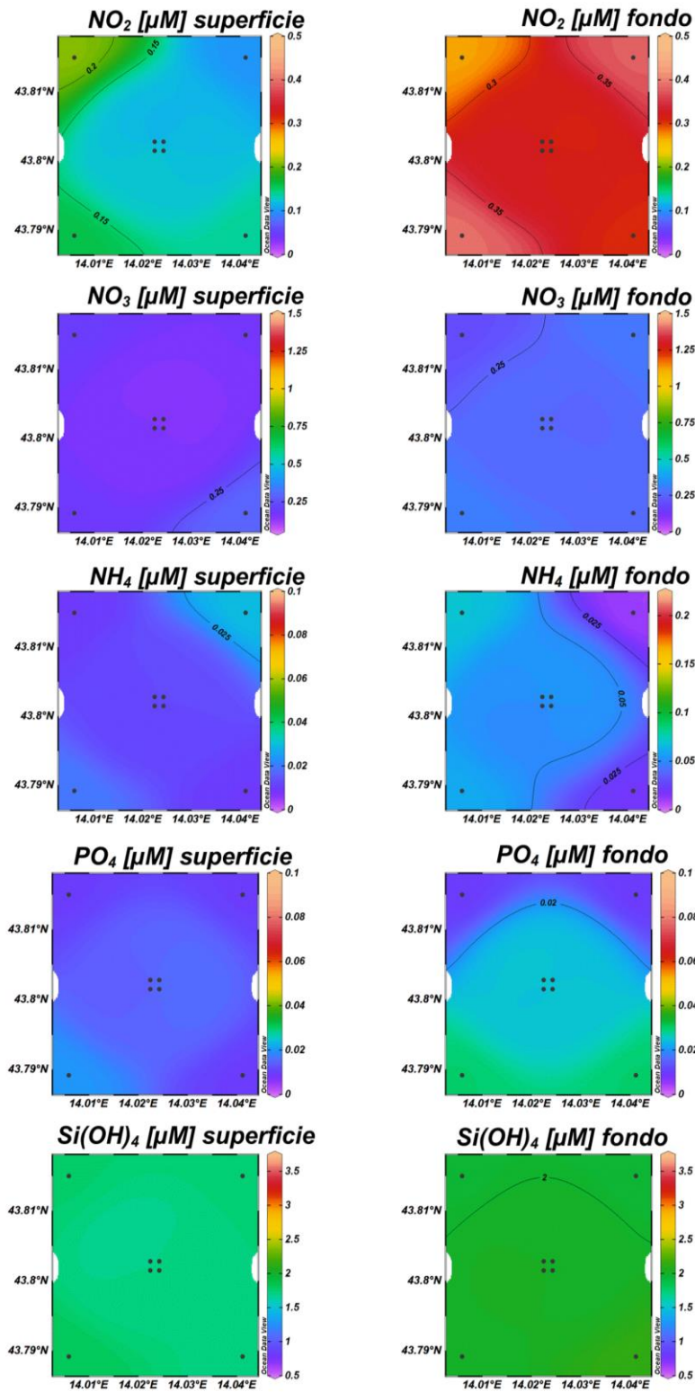
Fig. 3.17 - Mappe areali in superficie e al fondo rappresentanti le concentrazioni di fosfati (PO 4 ), silicati (Si(OH) 4 ), nitrati (NO 3 ), nitriti (NO 2 ) e ammonio (NH 4 ) espresse in \mu M. Marzo 2022.
