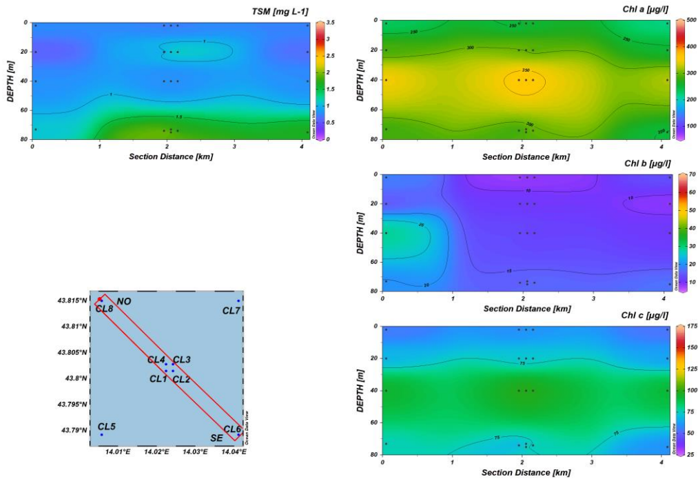
Fig. 3.26a - Sezioni NO-SE delle stazioni CL8, CL4, CL1, CL3, CL2 e CL6 rappresentanti le concentrazioni di particolato sospeso (TSM) espresso in \text{mg L}^{-1} , clorofilla a (Chl a), clorofilla b (Chl b), clorofilla c (Chl c), espresse in \text{ng L}^{-1} . Marzo 2022.
