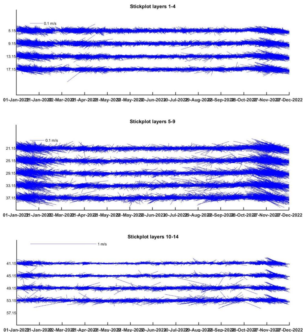
Fig. 3.44 - Stickplot delle correnti (medie giornaliere) lungo la colonna d'acqua ottenuti con il correntometro ADCP nel periodo gennaio - dicembre 2022.
