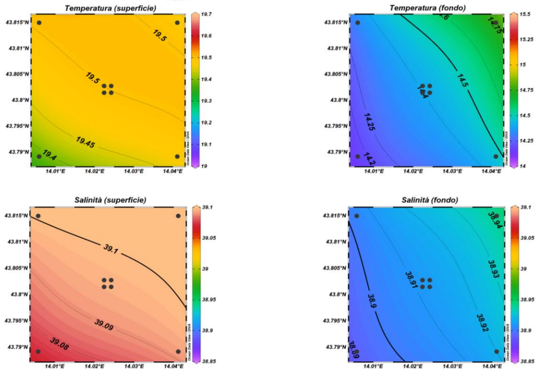
Fig. 3.11 - Mappe areali rappresentanti la temperatura (°C) e la salinità (psu) in superficie e al fondo. Campagna di Novembre 2022 . Grafico realizzato mediante il software Ocean Data View – ODV (© 2016 Reiner Schlitzer).
