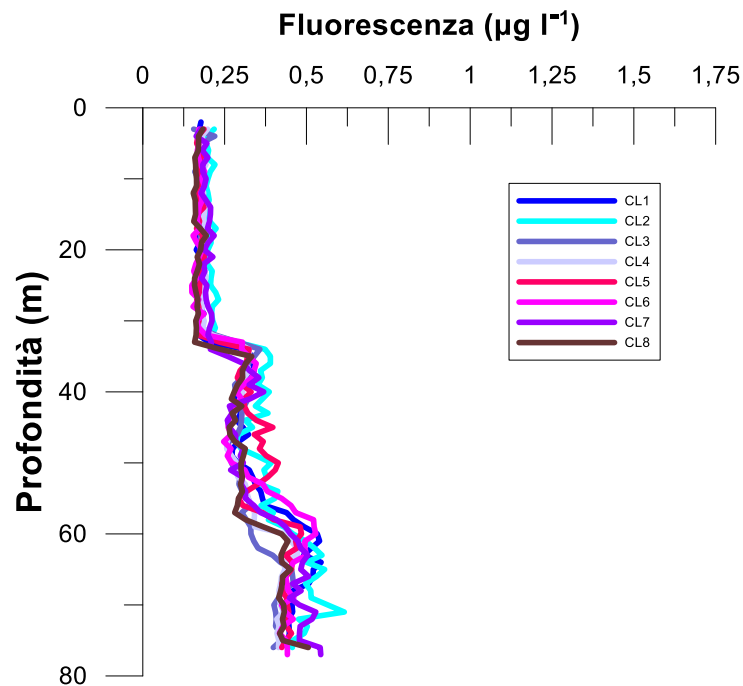
Fig. 3.12 - Profili di fluorescenza ( \mu\text{g L}^{-1} ). Campagna di Novembre 2022 .
