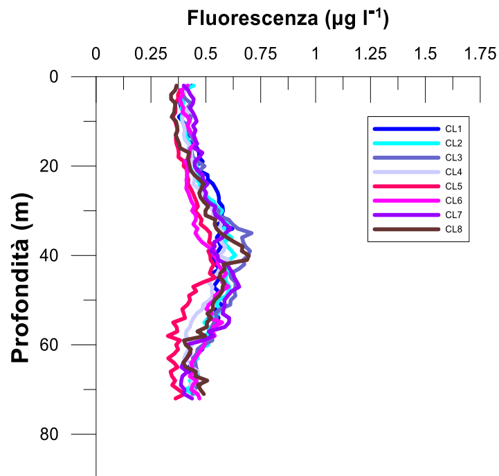
Fig. 3.3 - Profili di fluorescenza ( \mu\text{g L}^{-1} ). Marzo 2022 .
