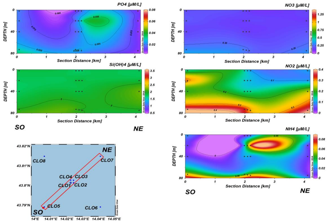
Fig. 3.16b - Sezioni SO-NE delle stazioni CL5, CL1, CL2, CL4, CL3 e CL7 rappresentanti le concentrazioni di fosfati ( \text{PO}_4 ), silicati ( \text{Si(OH)}_4 ), nitrati ( \text{NO}_3 ), nitriti ( \text{NO}_2 ) e ammonio ( \text{NH}_4 ) espresse in \mu\text{M} . Marzo 2022.
