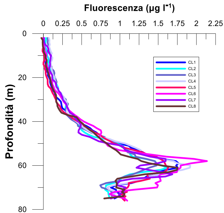
Fig. 3.6 - Profili di fluorescenza ( \mu\text{g L}^{-1} ). Maggio 2022.
