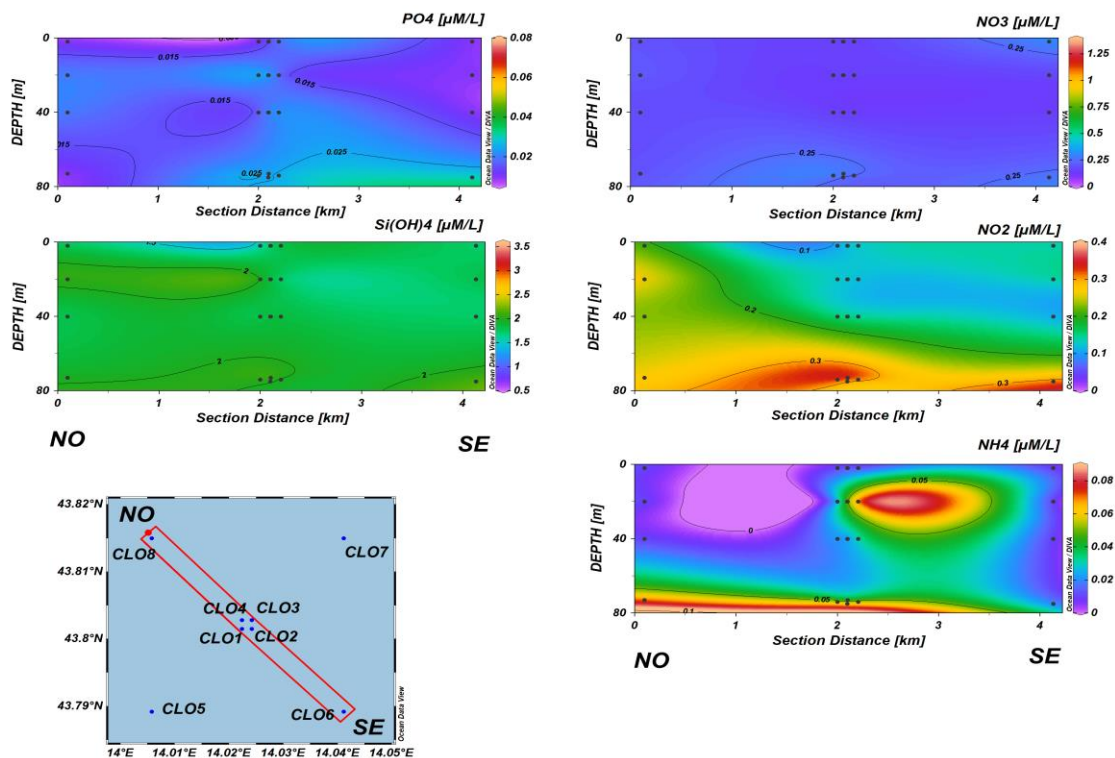
Fig. 3.16a - Sezioni NO-SE delle stazioni CL8, CL4, CL1, CL3, CL2 e CL6 rappresentanti le concentrazioni di fosfati ( \text{PO}_4 ), silicati ( \text{Si}(\text{OH})_4 ), nitrati ( \text{NO}_3 ), nitriti ( \text{NO}_2 ) e ammonio ( \text{NH}_4 ) espresse in \mu\text{M} . Marzo 2022.
