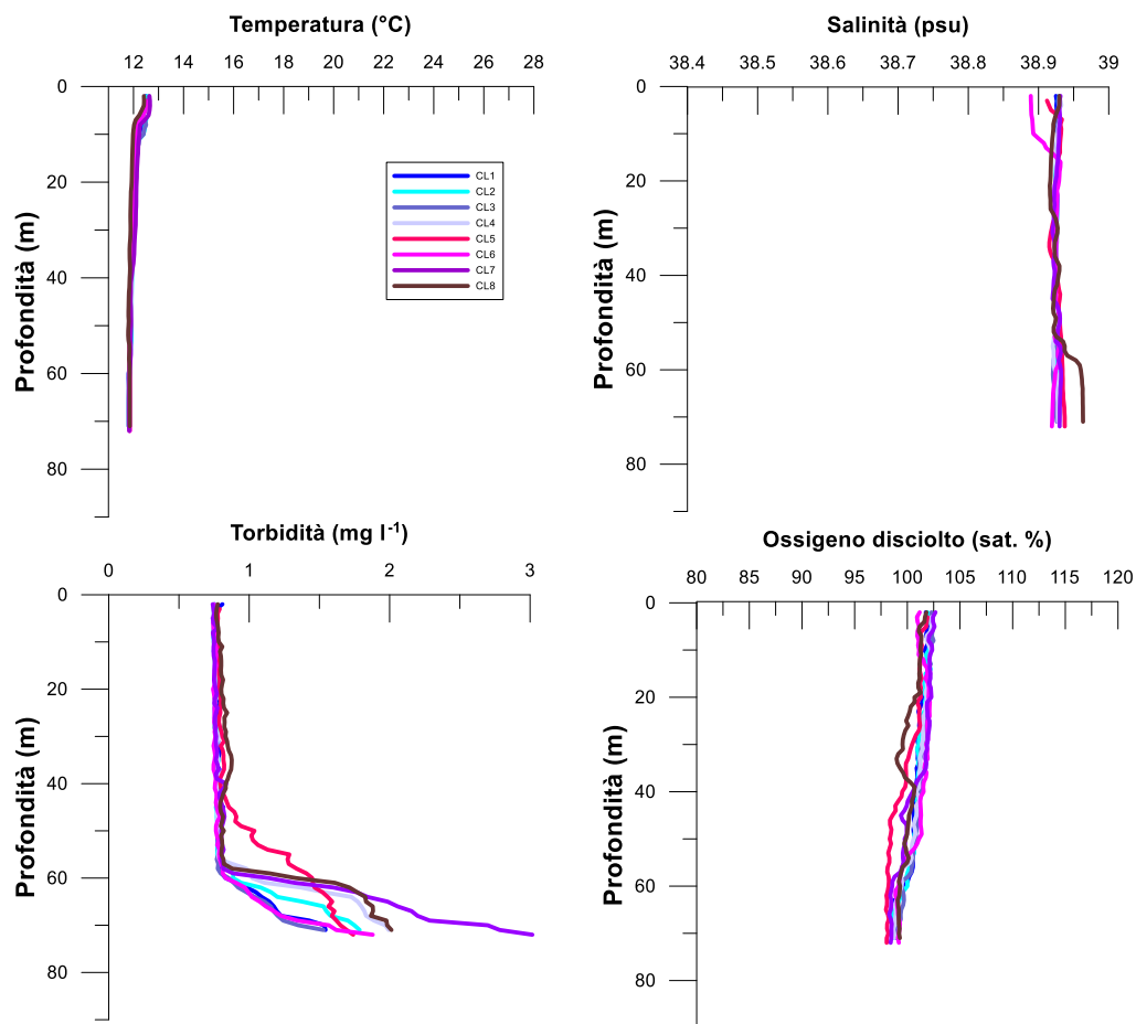
Fig. 3.1 - Profili di temperatura ( ^\circ\text{C} ), salinità (psu), torbidità ( \text{mg L}^{-1} ) e ossigeno disciolto in % di saturazione (sat %). Marzo 2022.
