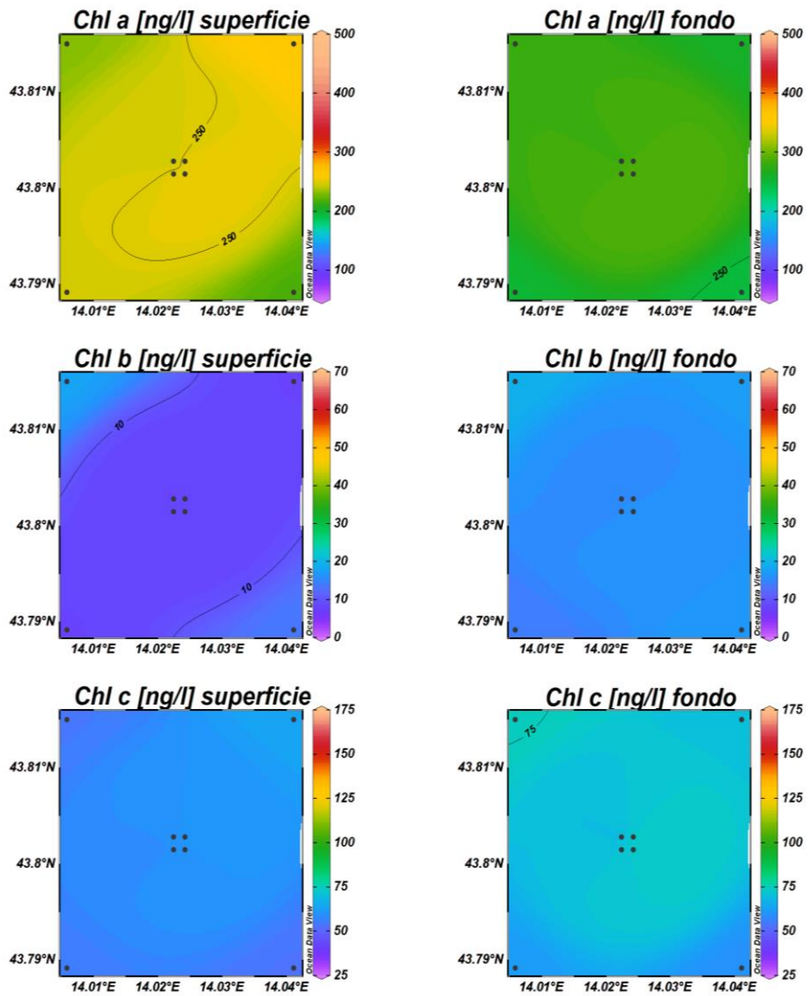
Fig. 3.27 - Mappe areali in superficie e al fondo rappresentanti le concentrazioni di clorofilla a (Chl a ), clorofilla b (Chl b ) e clorofilla c (Chl c ) espresse in ng L -1 . Marzo 2022.
