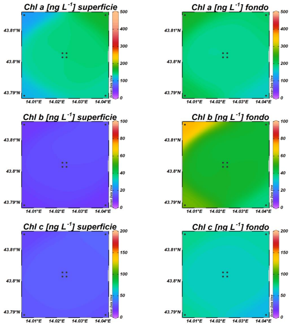
Fig. 3.33 - Mappe areali in superficie e al fondo rappresentanti le concentrazioni di clorofilla a (Chl a ), clorofilla b (Chl b ), clorofilla c (Chl c ), espresse in \text{ng L}^{-1} . Novembre 2022.
