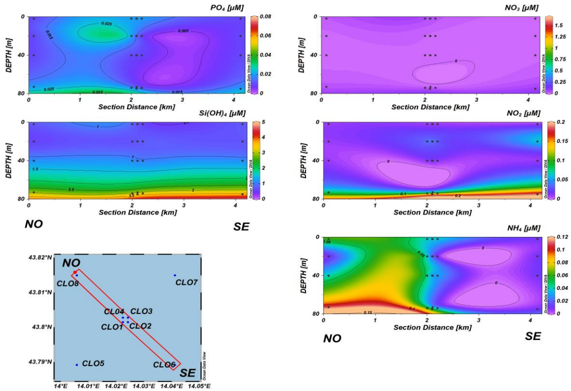
Fig. 3.20a - Sezioni NO-SE delle stazioni CL8, CL4, CL1, CL3, CL2 e CL6 rappresentanti le concentrazioni di fosfati ( PO_4 ), silicati ( Si(OH)_4 ), nitrati ( NO_3 ), nitriti ( NO_2 ) e ammonio ( NH_4 ) espresse in \mu M . Luglio 2022.
