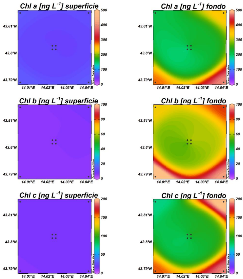
Fig. 3.31 - Mappe areali in superficie e al fondo rappresentanti le concentrazioni di clorofilla a (Chl a ), clorofilla b (Chl b ), clorofilla c (Chl c ), espresse in \text{ng L}^{-1} . Luglio 2022.
