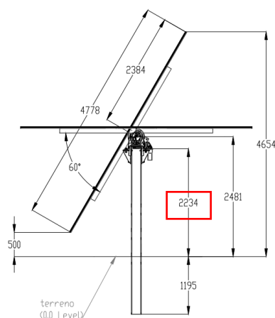
Sezione struttura tracker
