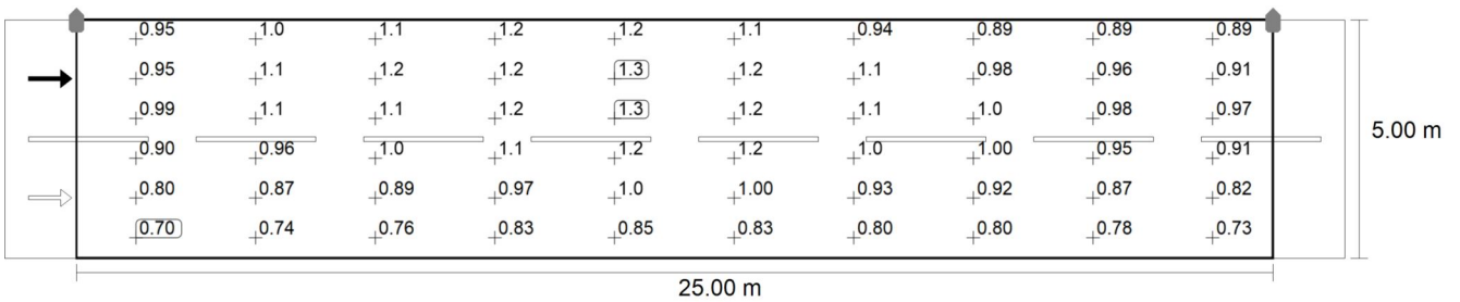
Osservatore 2: Luminanza per nuova installazione [cd/m²] (Raster dei valori)
