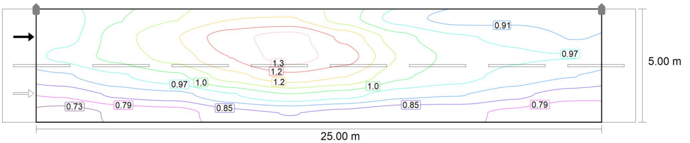
Osservatore 2: Luminanza per nuova installazione [cd/m²] (Curve isolux)
