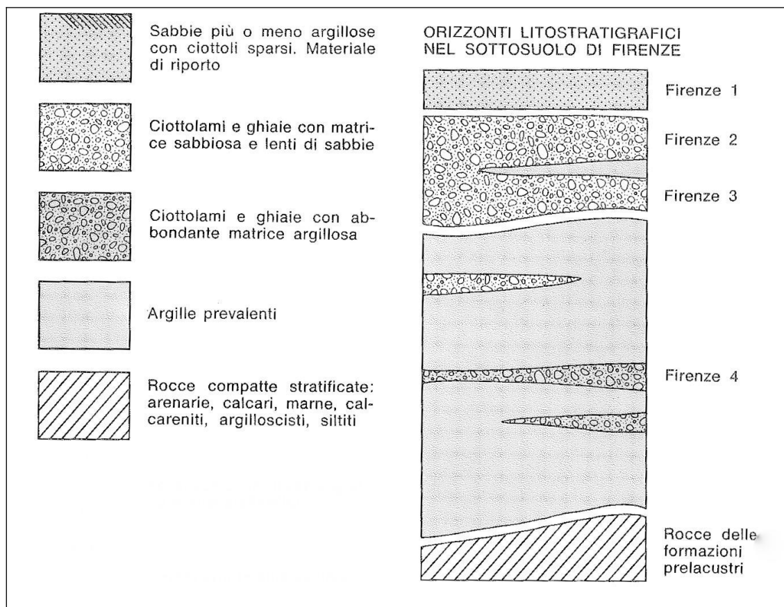
Figura 1 - Orizzonti stratigrafici presenti nel sottosuolo dell'area di Firenze (estratto da Capecchi et al. , 1976b).
