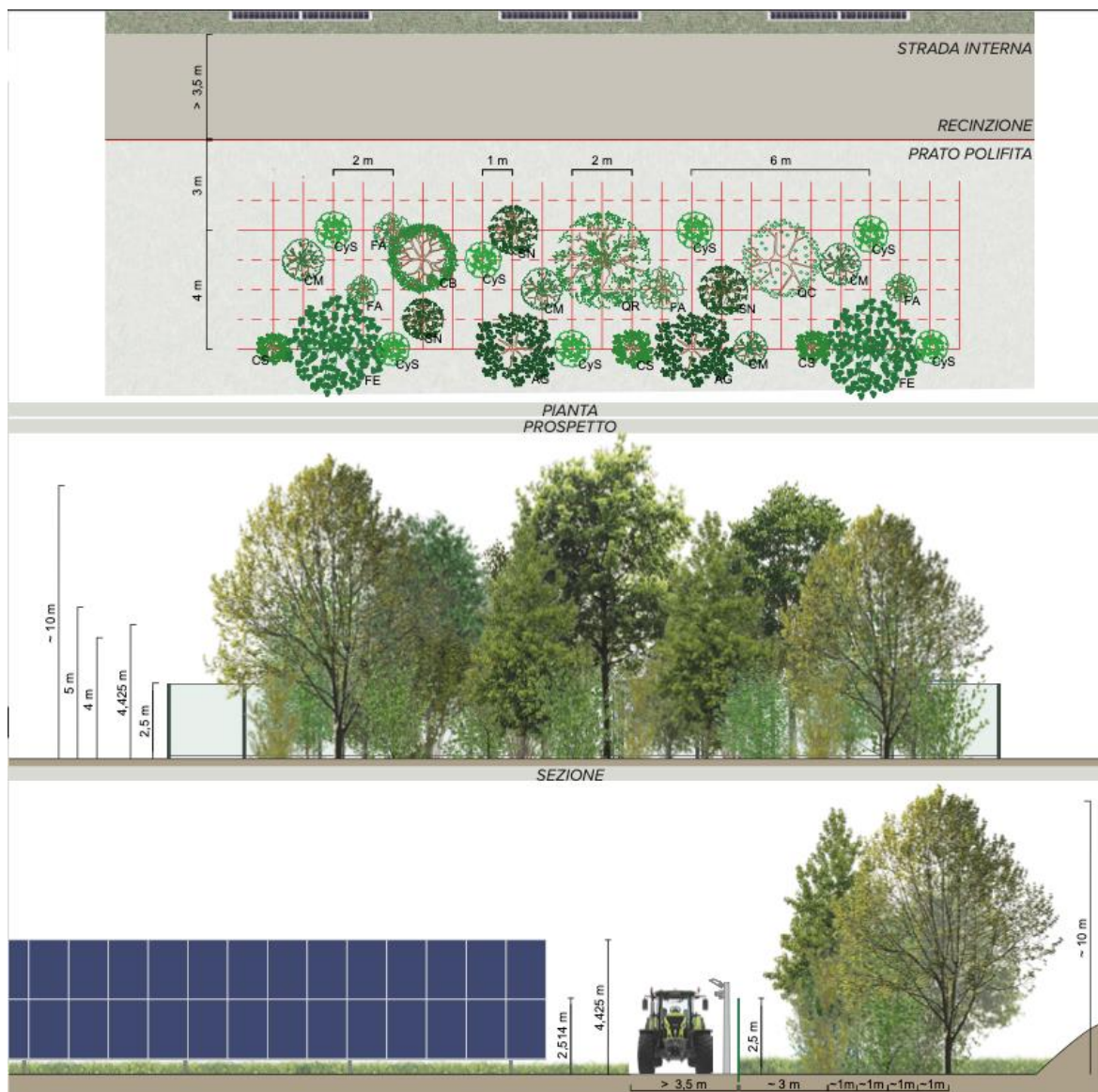
Figura 20 Sesto di impianto, prospetto e sezione delle fasce vegetate "Tipo 1". Immagine estratta dall'elaborato M_7.2_MAS_OMA_1_Particolari sest di impianto opere di mitigazione e compensazione ambientale.
