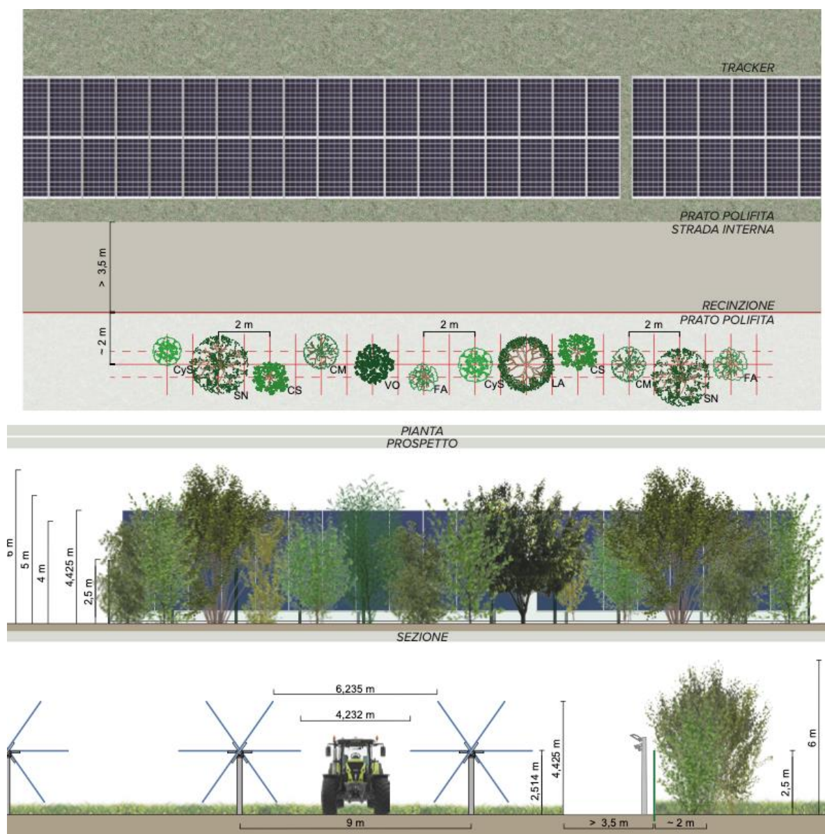
Figura 22 Sesto di impianto, prospetto e sezione delle fasce vegetate “Tipo 3”. Immagine estratta dall’elaborato M_7.2_MAS_OMA_1_Particolari sestì di impianto opere di mitigazione e compensazione ambientale.
