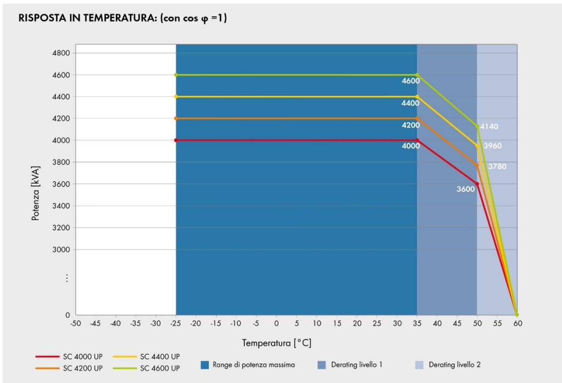
Figura 9: Prestazioni dell'inverter
