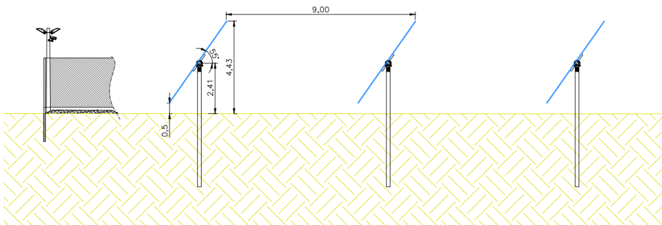
Figura 4: Sezione Tracker (Dimensioni in metri)
