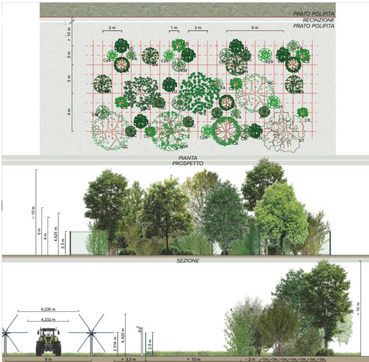
Figura 23 Sesto di impianto, prospetto e sezione delle fasce vegetate "Tipo 4". Immagine estratta dall'elaborato M_7.2_MAS_OMA_1_Particolari sestì di impianto opere di mitigazione e compensazione ambientale.
