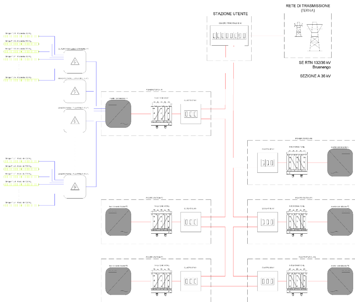
Figura 6: Schema a blocchi
