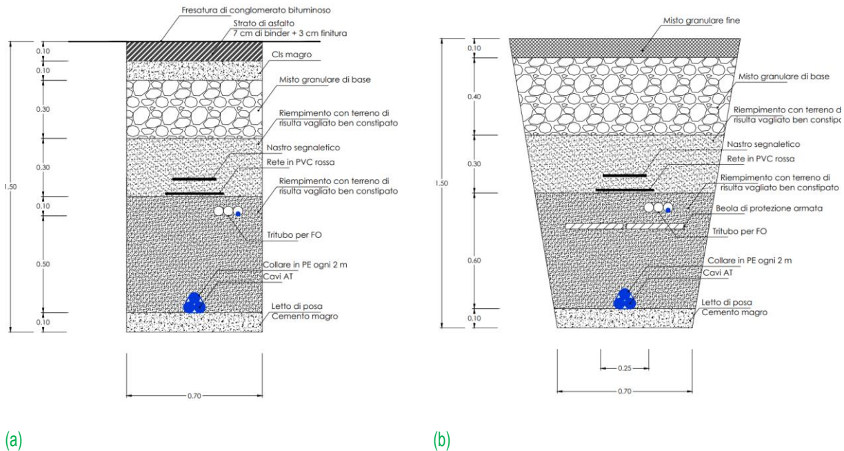
Figura 13: Modalità di posa sotto strada asfaltata (a) e su terreno agricolo (b)
