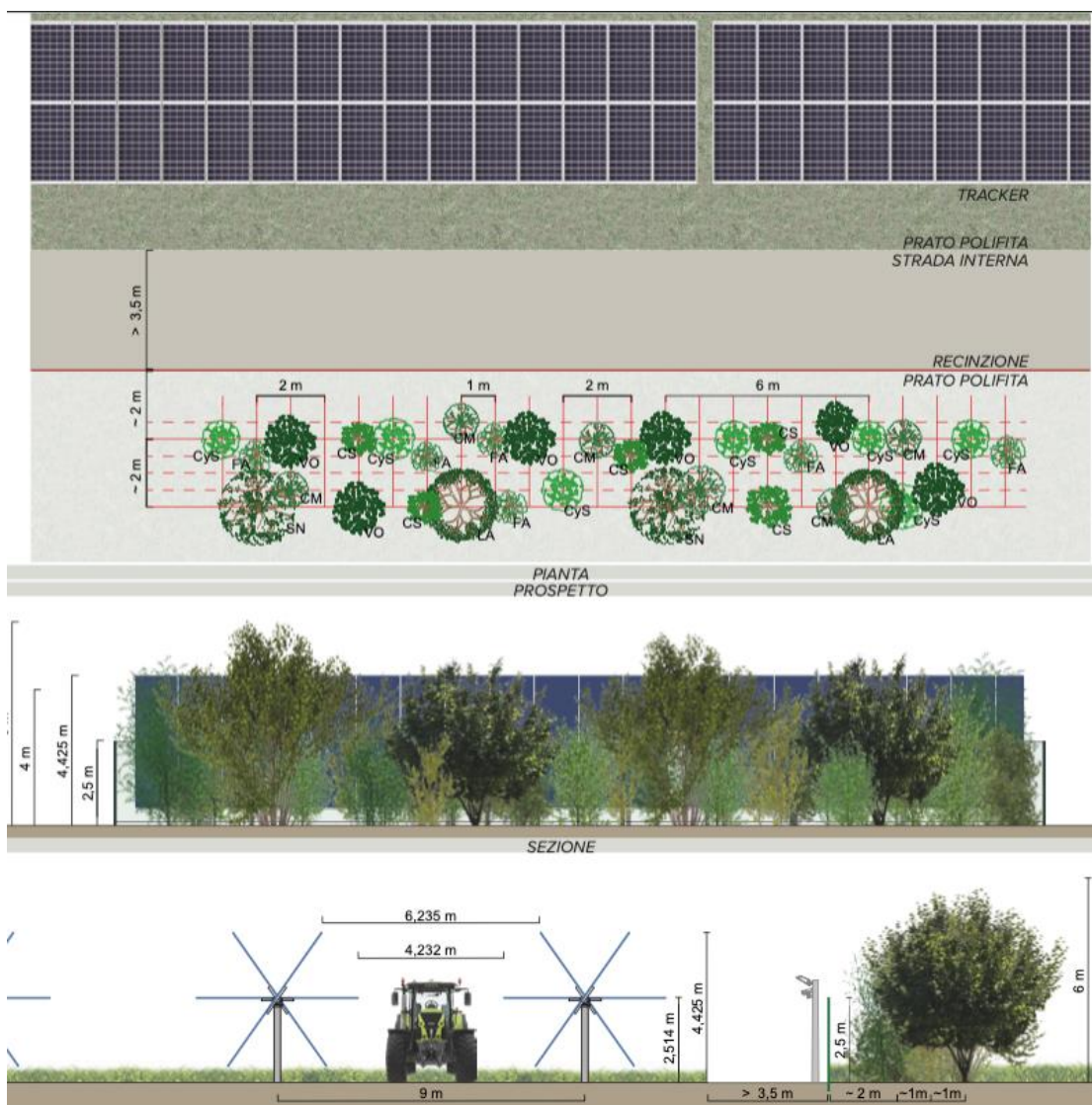
Figura 21 Sesto di impianto, prospetto e sezione delle fasce vegetate "Tipo 2". Immagine estratta dall'elaborato M_7.2_MAS_OMA_1_Particolari sestì di impianto opere di mitigazione e compensazione ambientale.
