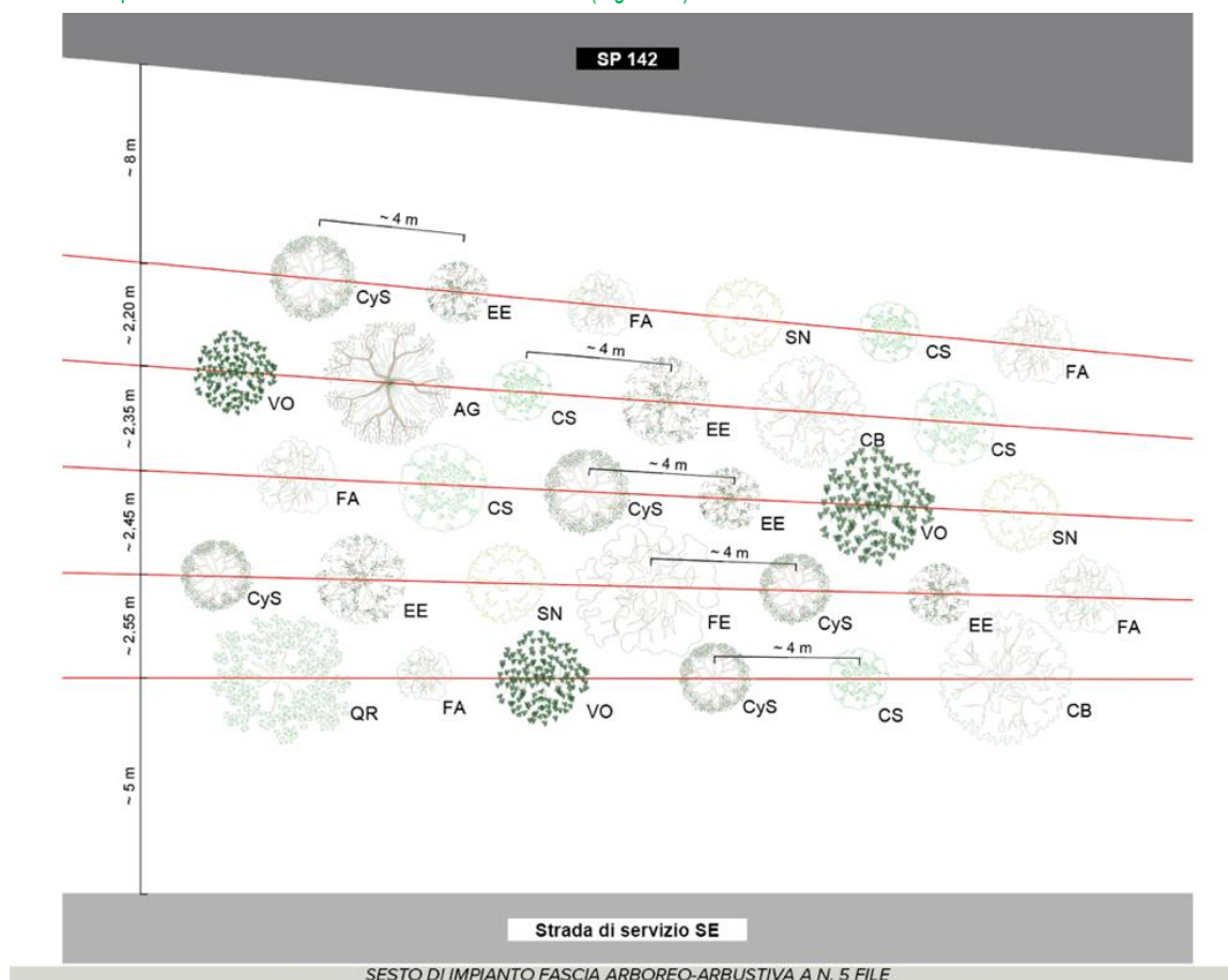
Figura 31 Estratto del sesto di impianto a n. 5 file.
