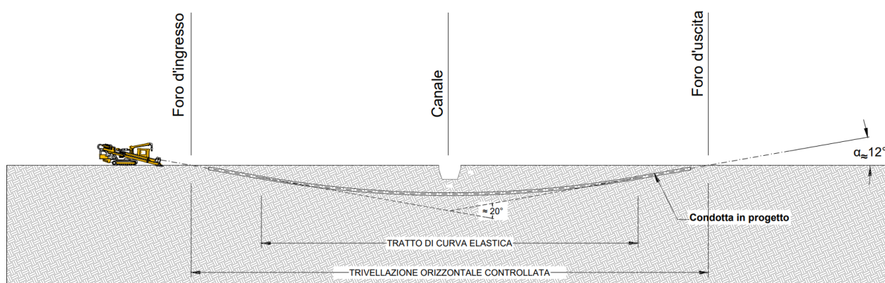
Figura 14: Esempio di Trivellazione Orizzontale Controllata
