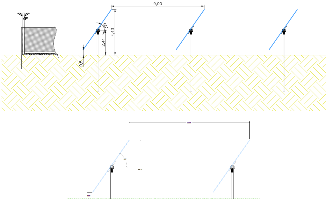
Figura 8. Sezione Tracker (Dimensioni in metri)
