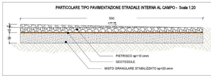
Figura. 36 - Particolare tipo pavimentazione delle viabilità di servizio interne
