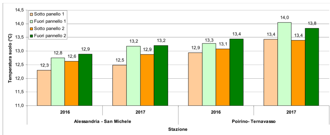
Figura 57. Confronto 2016-2017 dei valori medi di temperatura nel suolo
