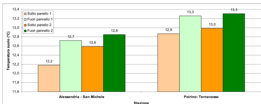
Figura 56. Valori medi di temperatura del suolo nel 2017
