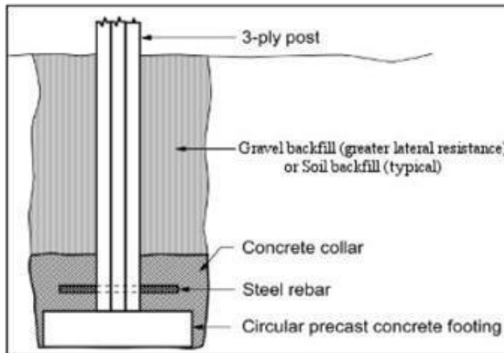
Figura 4. Esempio di fondazione ottenuta mediante perforazione del terreno e successiva creazione del palo di fondazione con getto di cemento
