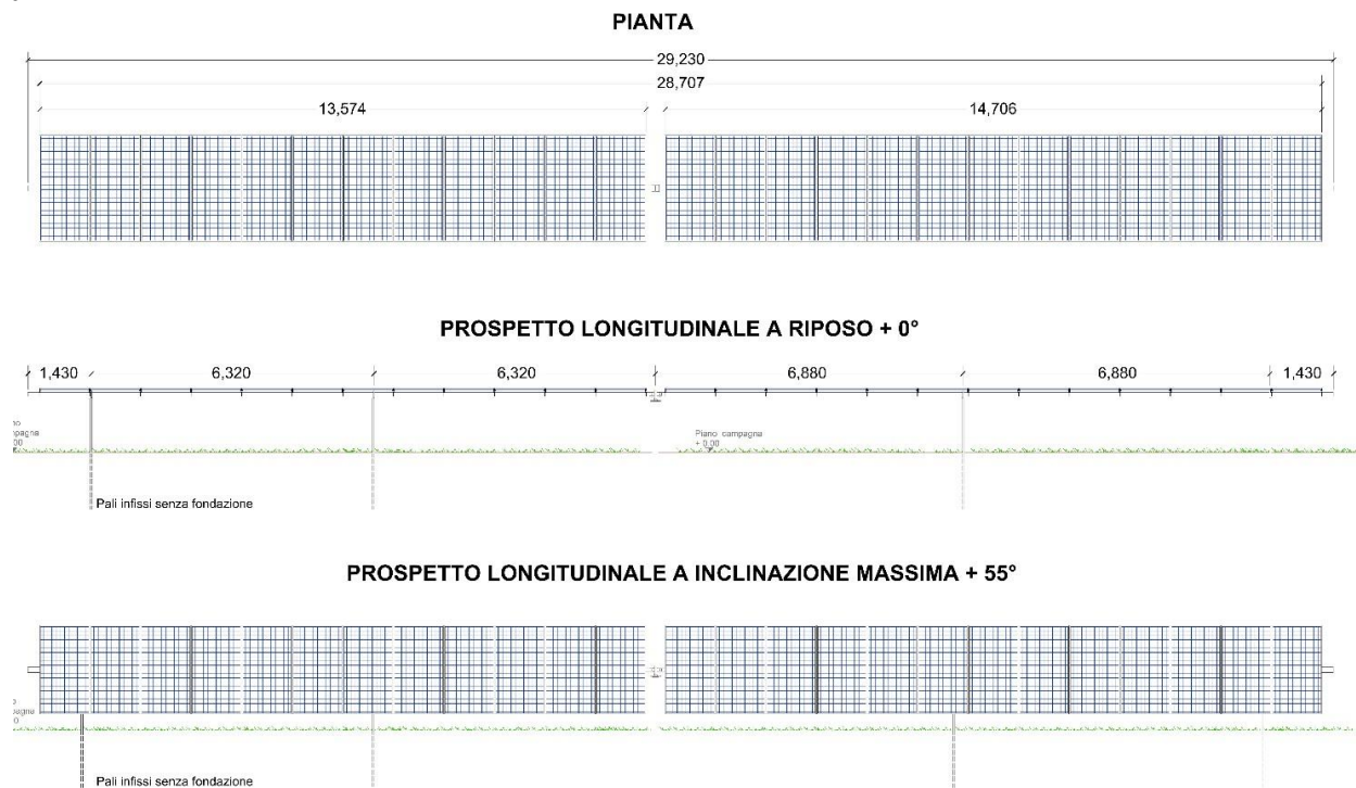
Figura 35 - : Infissione nel terreno delle strutture metalliche di sostegno dei moduli fotovoltaici (vista in sezione).
