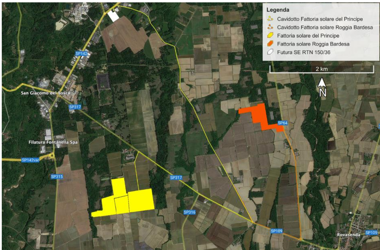
Figura 68. Aree di cantiere e opere di rete per i progetti fattoria solare del Principe e fattoria solare Roggia Bardesa
