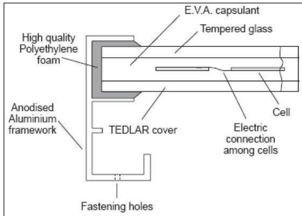
Figura 58. Sezione del modulo fotovoltaico tipo
