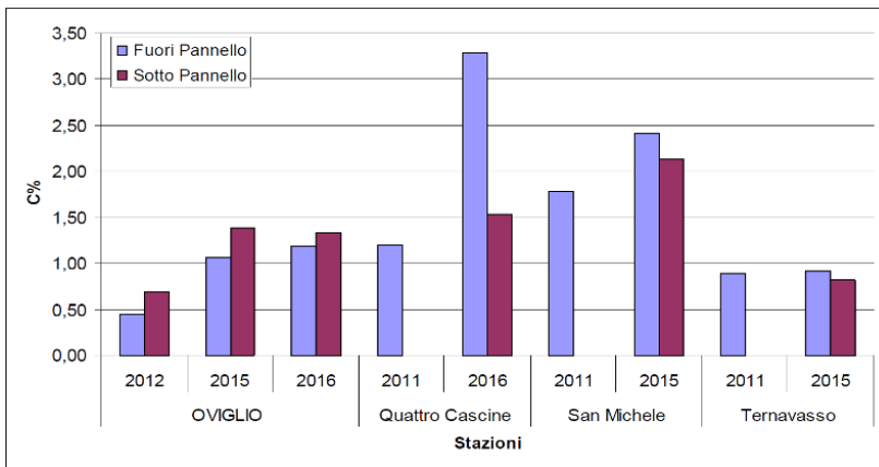
Figura 52. Risultanze dei monitoraggi condotti da IPLA (IPLA, 2017) che attestano, nella maggior parte dei casi, un progressivo incremento della dotazione di Carbonio organico sia sotto copertura, sia nell'interfilare tra le stringhe fotovoltaiche.
