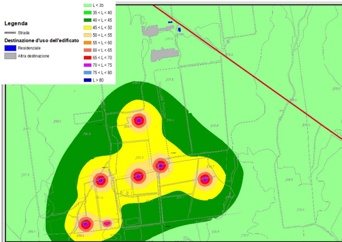
Figura 51. mappa acustica diurna – fase di esercizio (fonte: Studio previsionale Acustico M_12.5_MAS).
