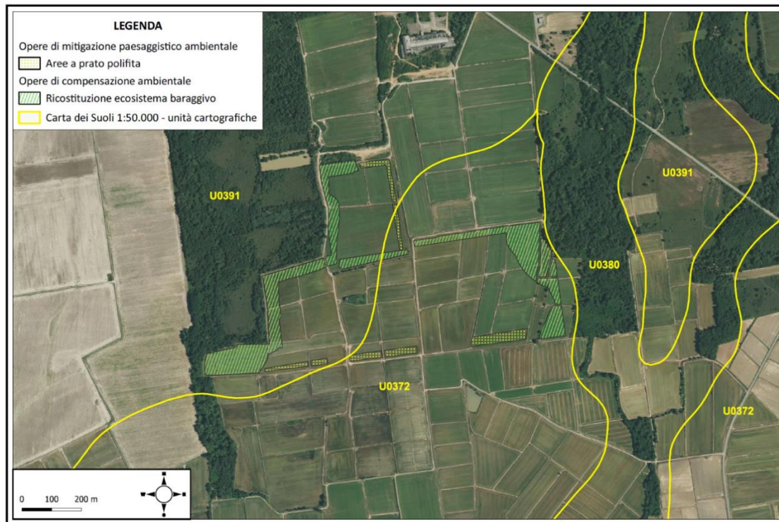
Figura 73. Carta dei suoli a scala 1:50.000 della Regione Piemonte
