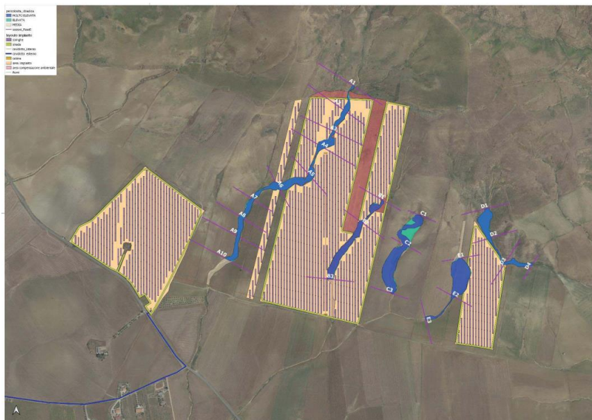
Figura 41: Planimetria delle aree allagabili
