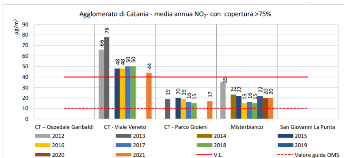
Figura 7: Media annua NO 2 - Agglomerato di Catania (Fonte: Arpa Sicilia)
