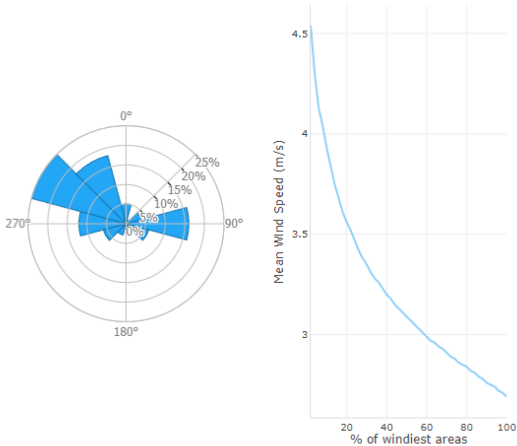
Figura 36: Wind Speed Rose a 10 m relativa all'area di impianto. La velocità del vento a 10 m risulta pari a 3.93 m/s
