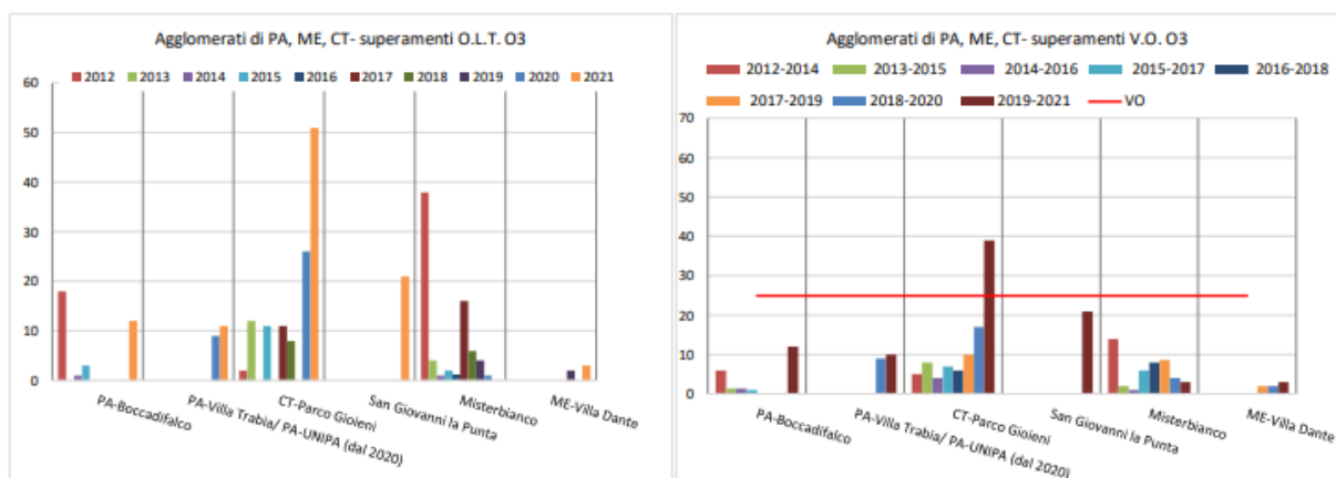
Figura 15:Trend del numero di superamenti OLT e VO agglomerati di PA,ME,CT
