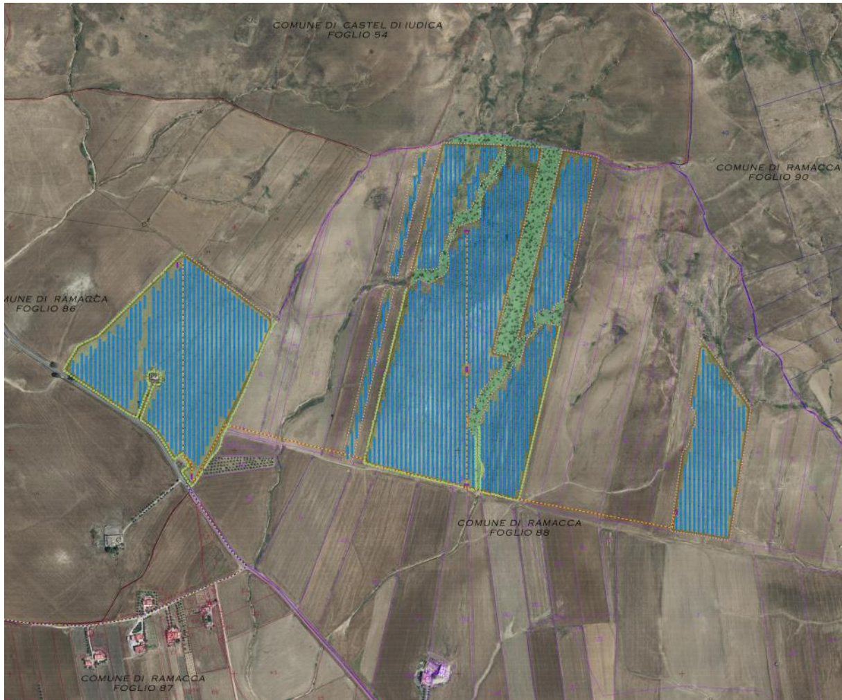
Figura 50: Layout definitivo e aree di mitigazione e/o compensazione
