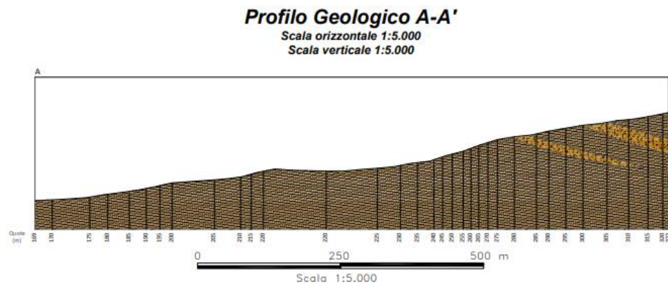
Figura 42: Stralcio Profilo Geologico
