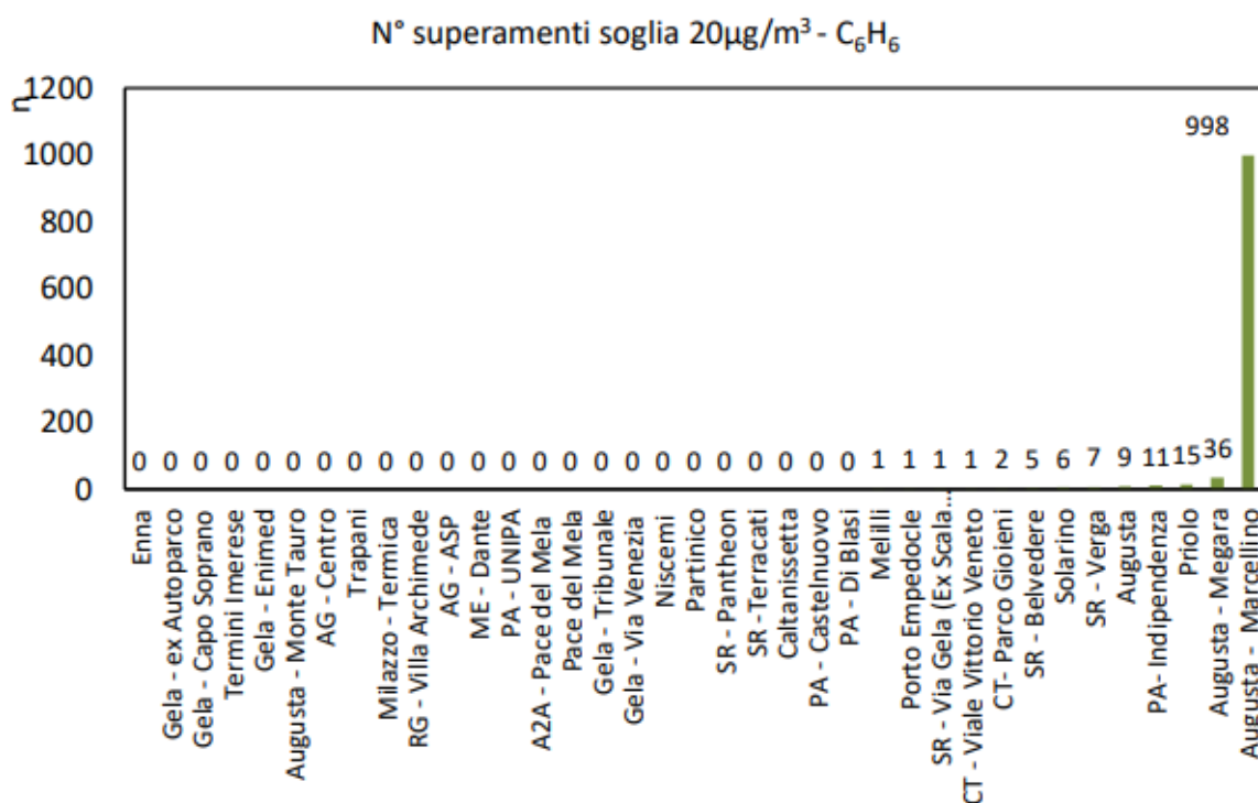
Figura 21: Trend dei numeri di superamenti della soglia di 20 µg/m 3 - Anno 2021
