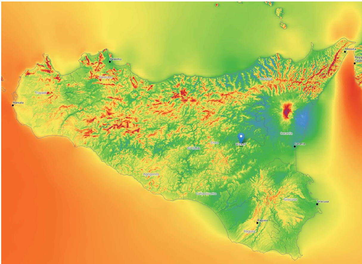
Figura 35: Velocità media del vento in tempo reale a 50 metri pari a 4.75 m/s (Fonte: Global Wind Atlas)
