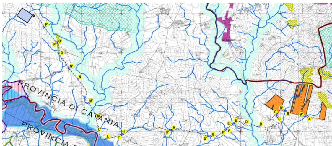
Figura 31: interferenze del parco di Ramacca (CT), da realizzare in località "Masseria Magazzinazzo", con le infrastrutture presenti - stralcio dell'elaborato grafico "Planimetria con individuazione delle interferenze"
