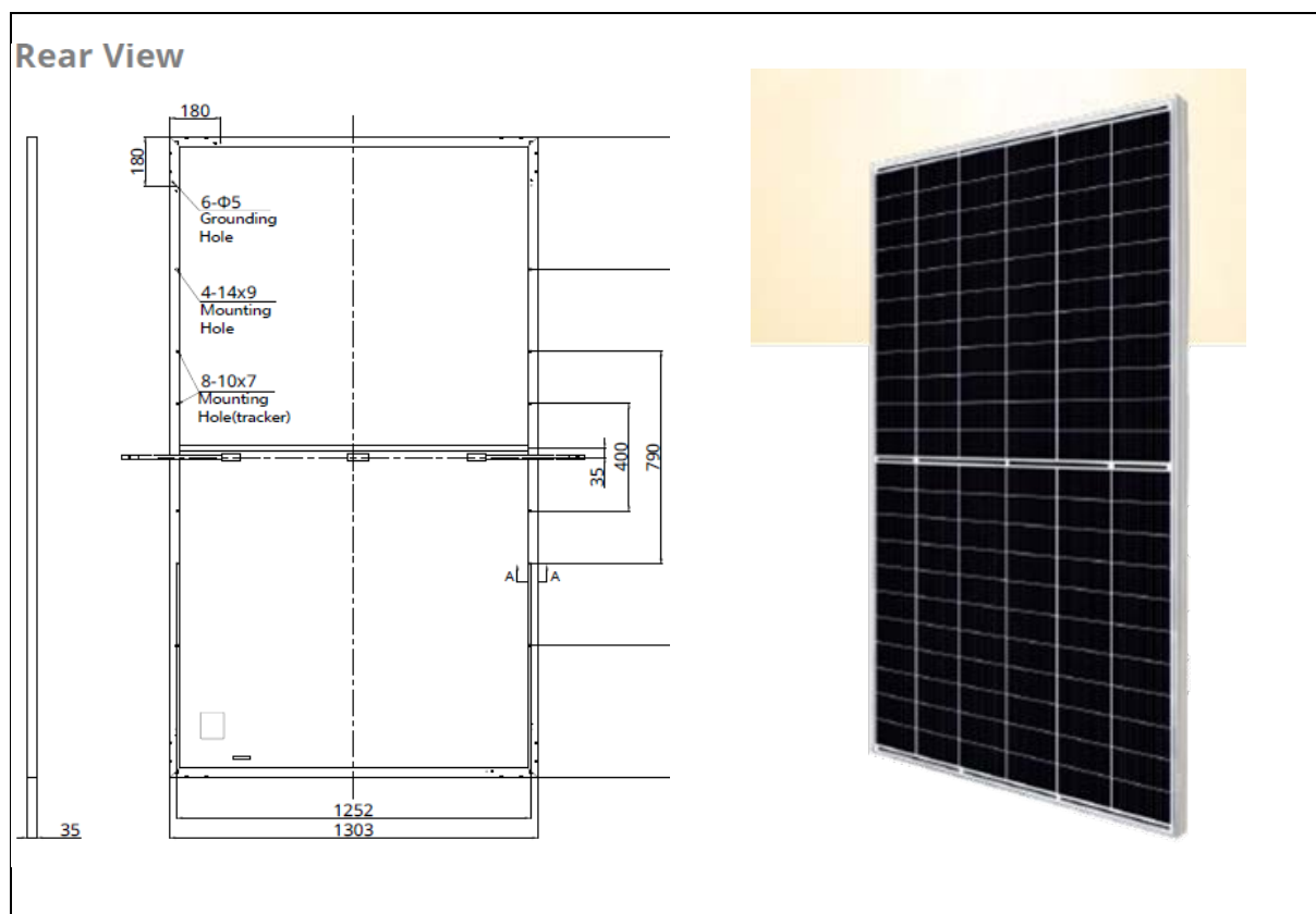
Figura 34: pannello FV fino a 665 Wp con dimensioni 2384 x 1303 x 35 mm
