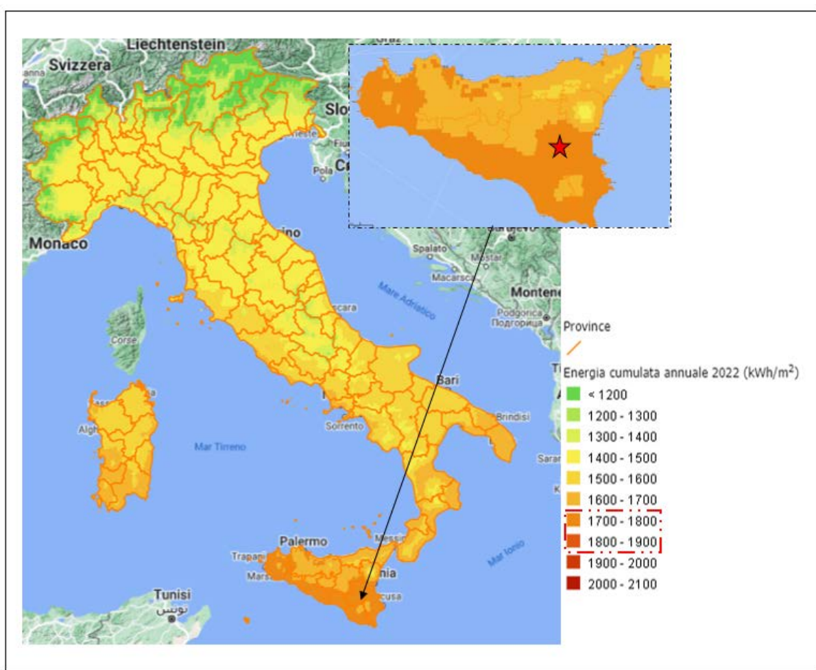
Figura 8: Regime insolazione anno 2022 - Fonte: RSE ( https://sunrise.rse-web.it/ )
