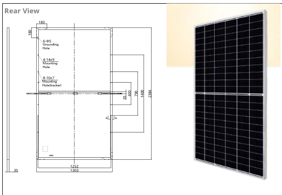
Figura 2: pannello FV fino a 665 Wp con dimensioni 2384 x 1303 x 35 mm
