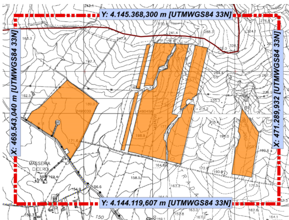
Figura 9: Inquadramento generale dell'area di realizzazione dell'impianto fotovoltaico da 25 MW in agro nel comune di Ramacca (CT) in località "Masseria Magazzinazzo"
