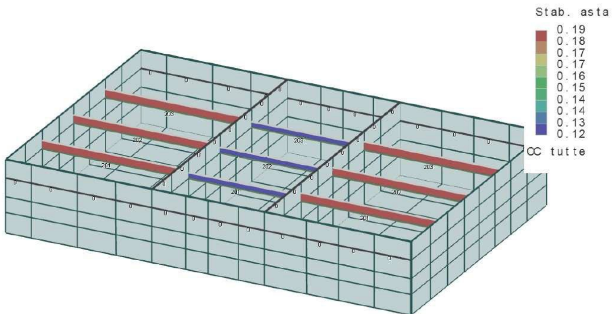
Figura 1 - Tasso di sfruttamento a pressoflessione
