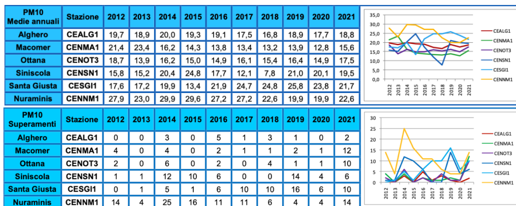
Fig. 19-20: Medie annuali di biossido di PM10 e superamento dei valori ( \mu\text{g}/\text{m}^3 ).
