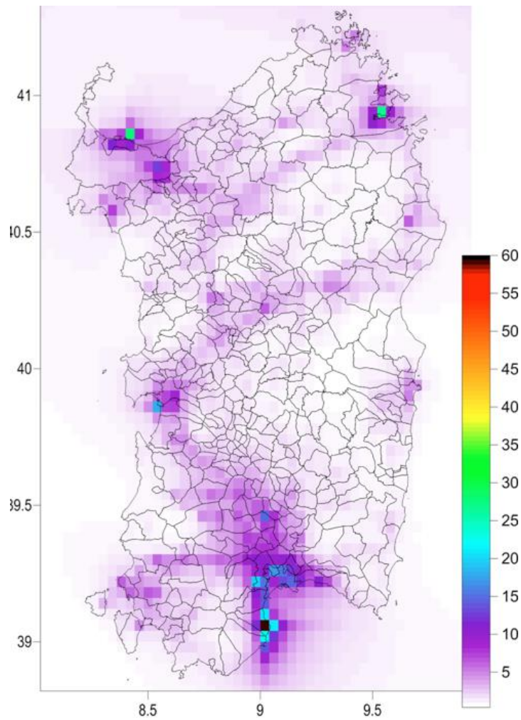
Fig. 11: Media annuale stimata delle concentrazioni di NO 2 sul territorio regionale (modello CHIMERE).
