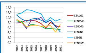
Fig. 18: Medie annuali di biossido di azoto ( \mu\text{g}/\text{m}^3 ).
