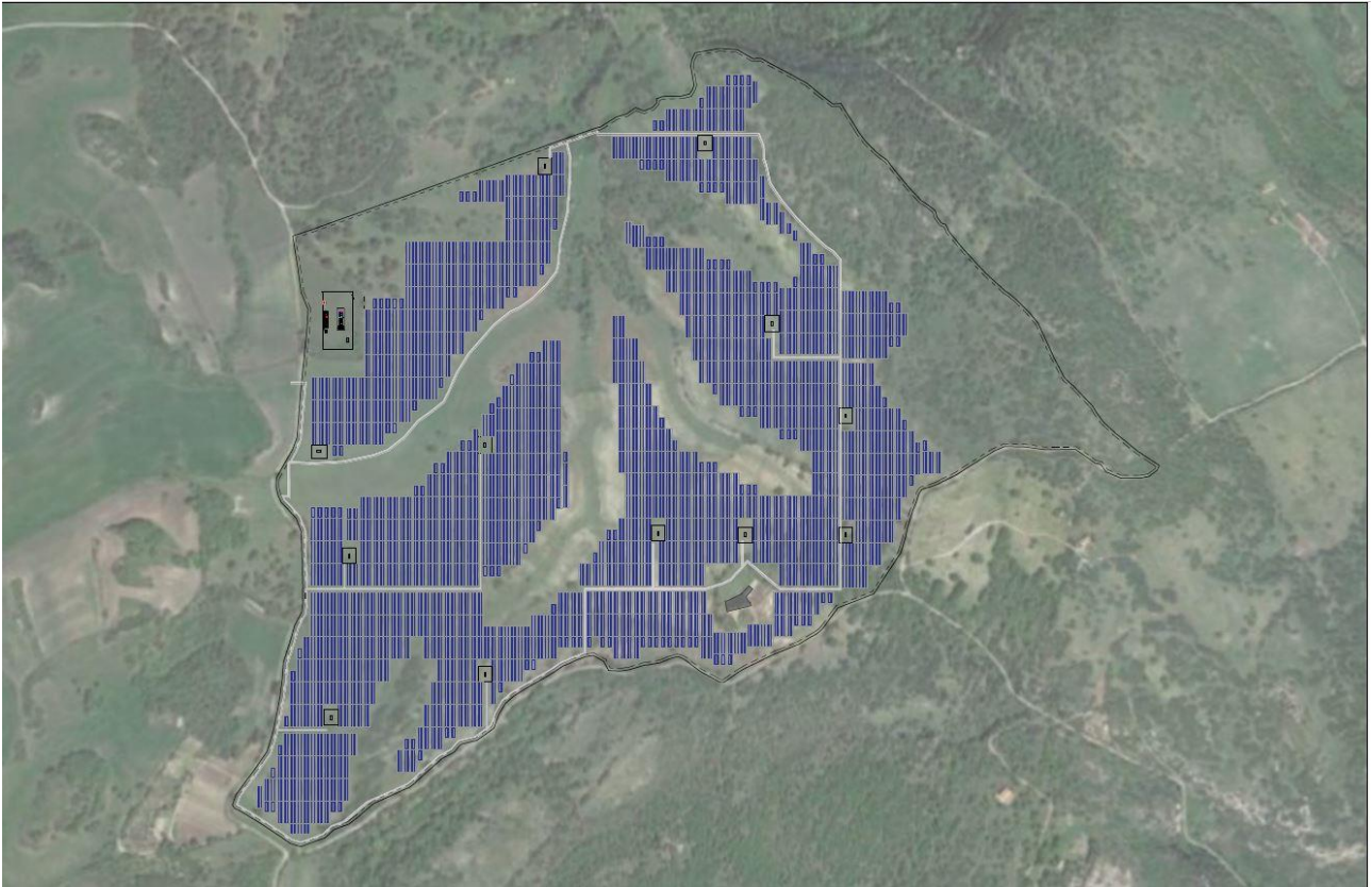
Fig. 1: Layout su ortofoto.
