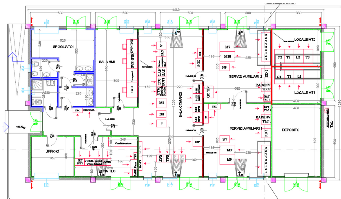
Figura 7 – planimetria edificio comandi
