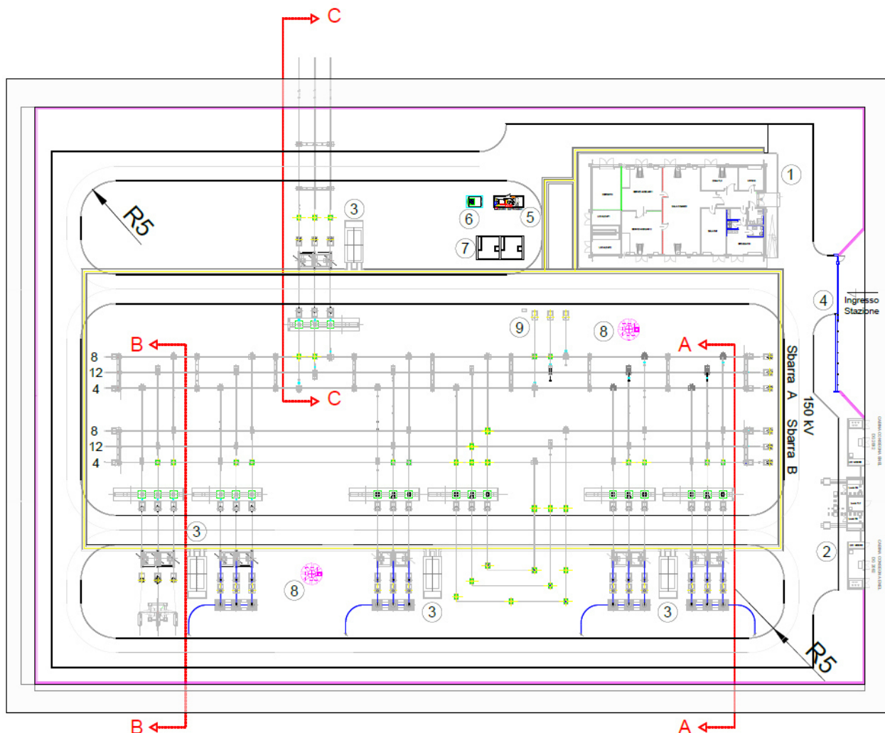
Figura 6 – planimetria elettromeccanica
