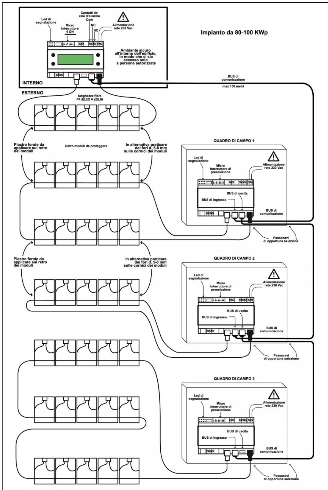
Figura 9 – Sistema di antifurto dei moduli FV
