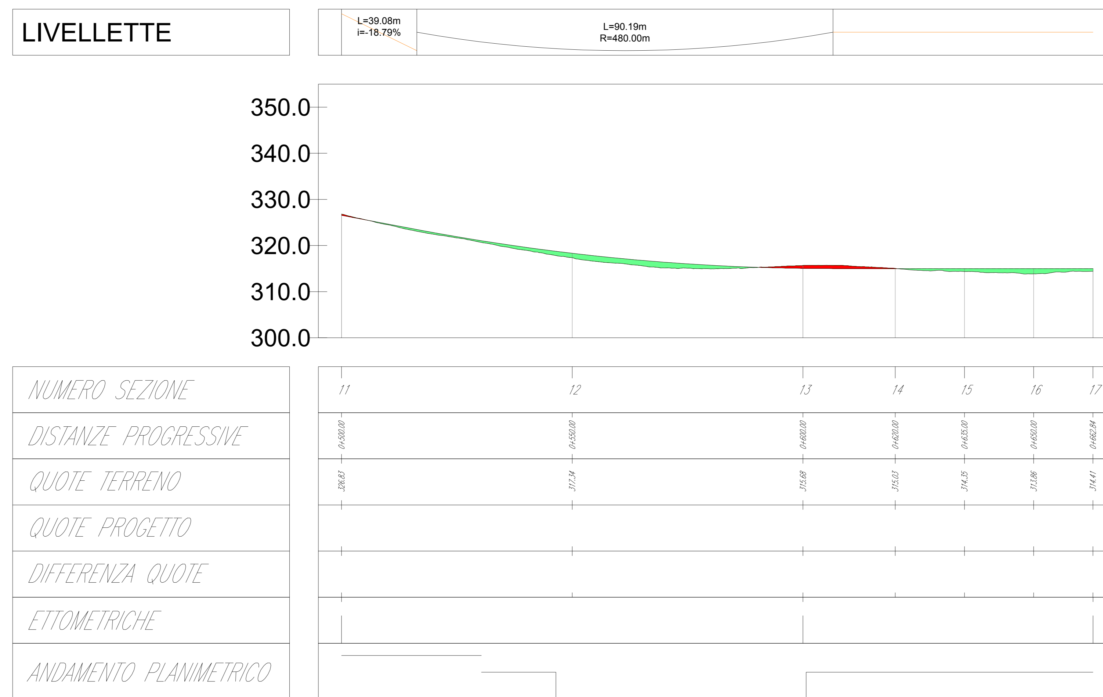
Profilo: PROFILO LONGITUDINALE STRADA SF7 (2) Q.Rif. : 300.00
