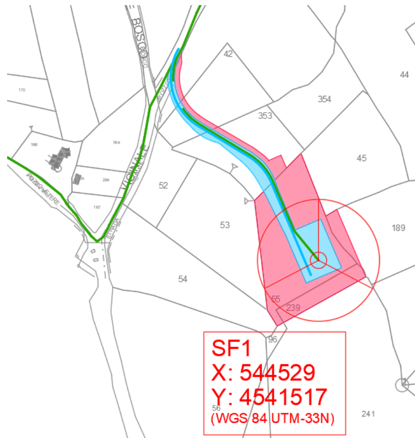
Figura 5 – Dettaglio strade di accesso-aree provvisorie e definitive
