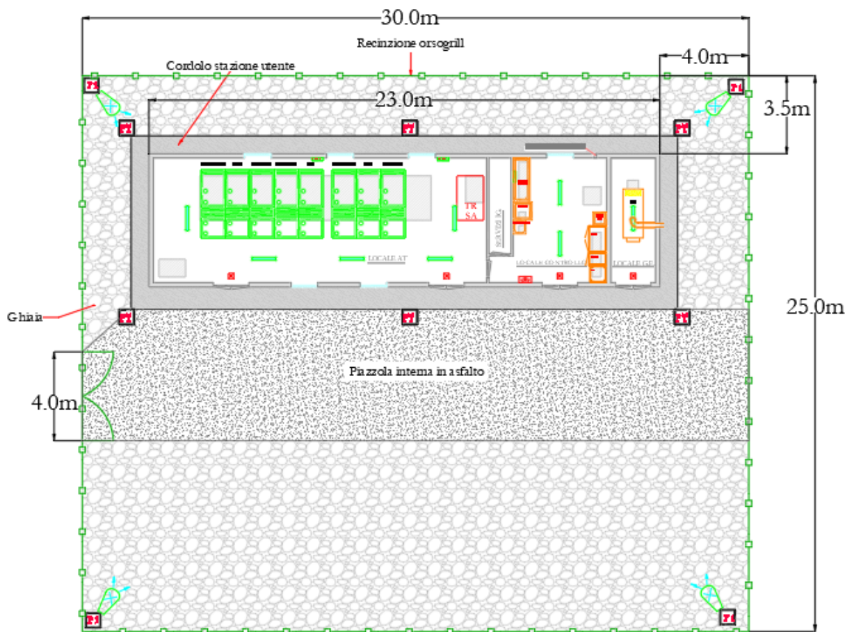
Figura 13 – Planimetria della Stazione Utente
