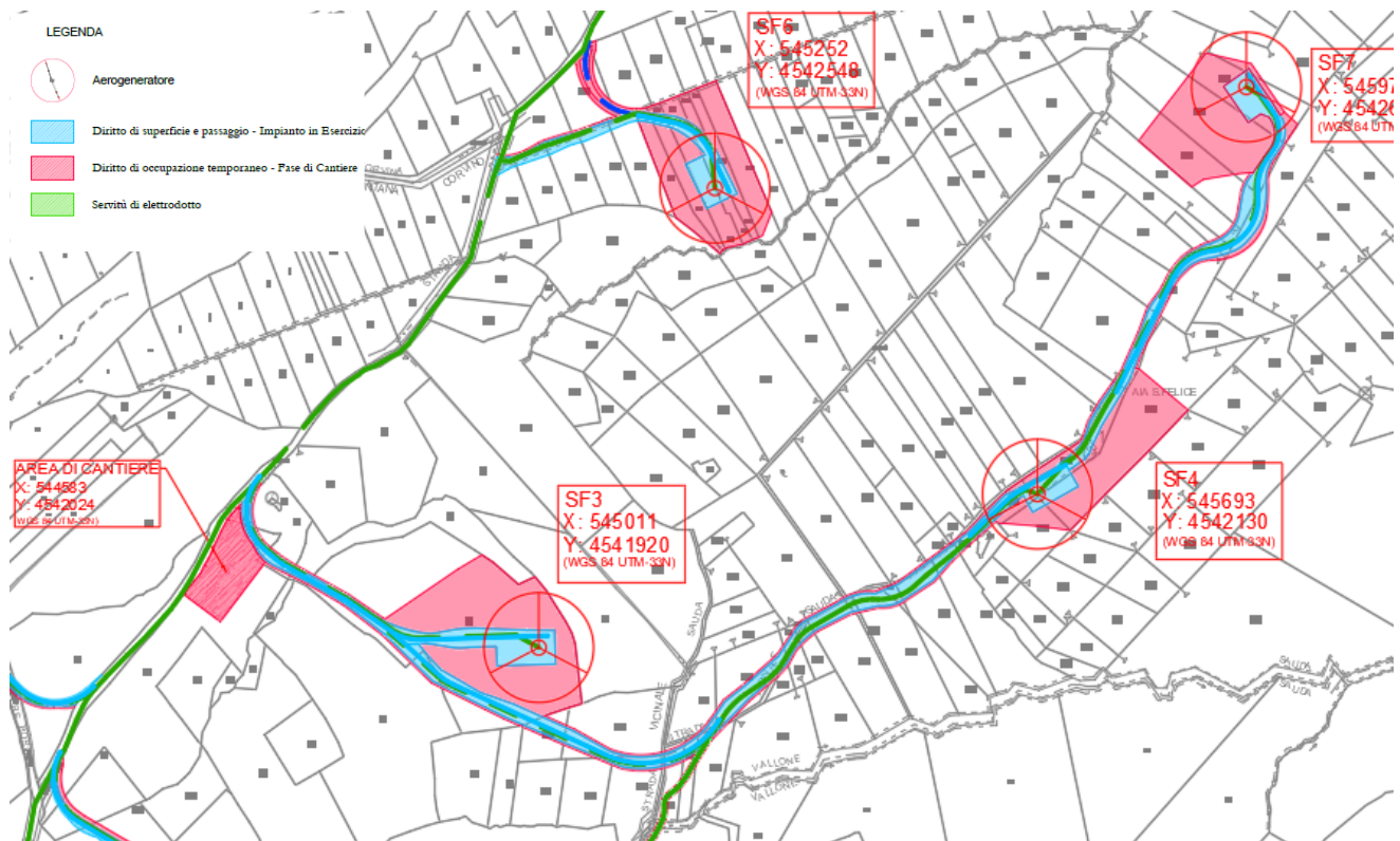
Figura 3 - Rappresentazione grafica generale aree di occupazione e servitù (1/2)
