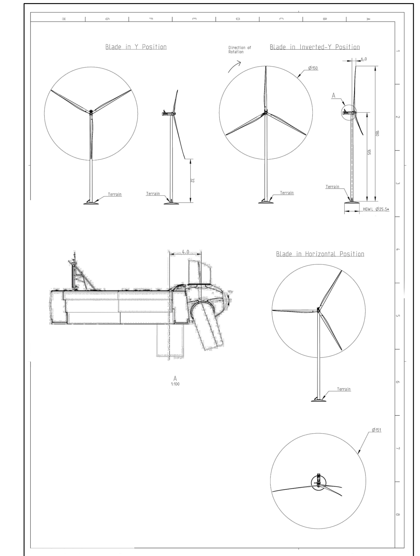
Disegni tecnici aerogeneratore
