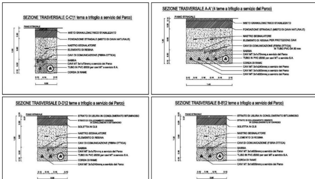
Figura 7. Differenti tipologie di posa del cavidotto
