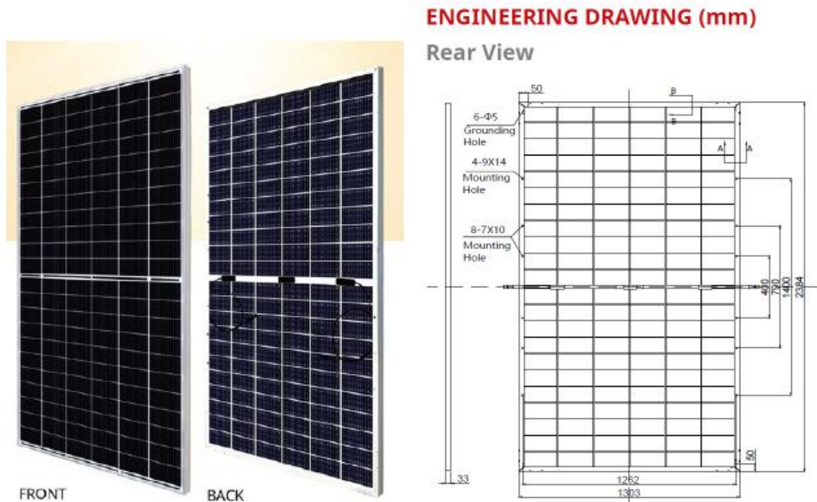
Figura 3. Pannello FV fino a 665 Wp con dimensioni 2384 x 1303 x 35 mm esempio
