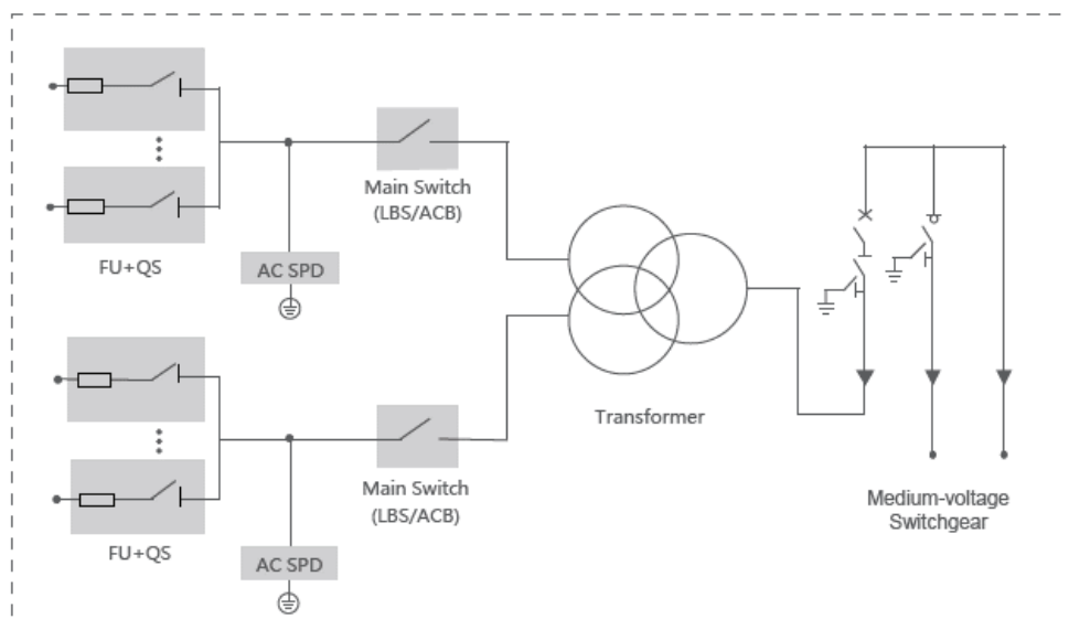
Figura 6. Schema di un possibile collegamento del trasformatore e delle relative protezioni
