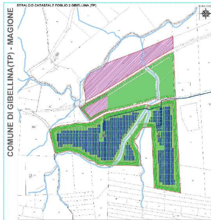
Figura 5 B – Layout dell’impianto ricadente in Contrada Magione con cavidotto
