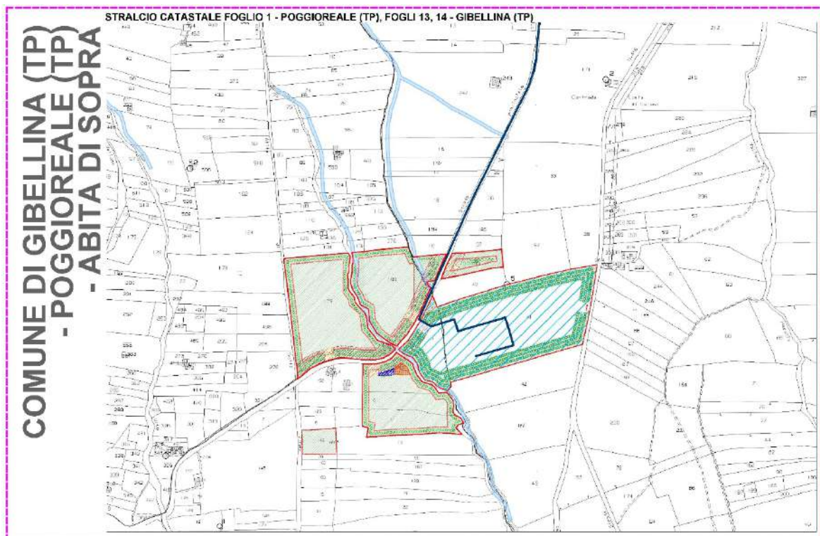
Figura 4 D – Layout dell'area di produzione di idrogeno ricadente in Contrada Abita di Sopra , nei territori di Gibellina (TP) e Poggioreale (TP) e cavidotto di connessione
