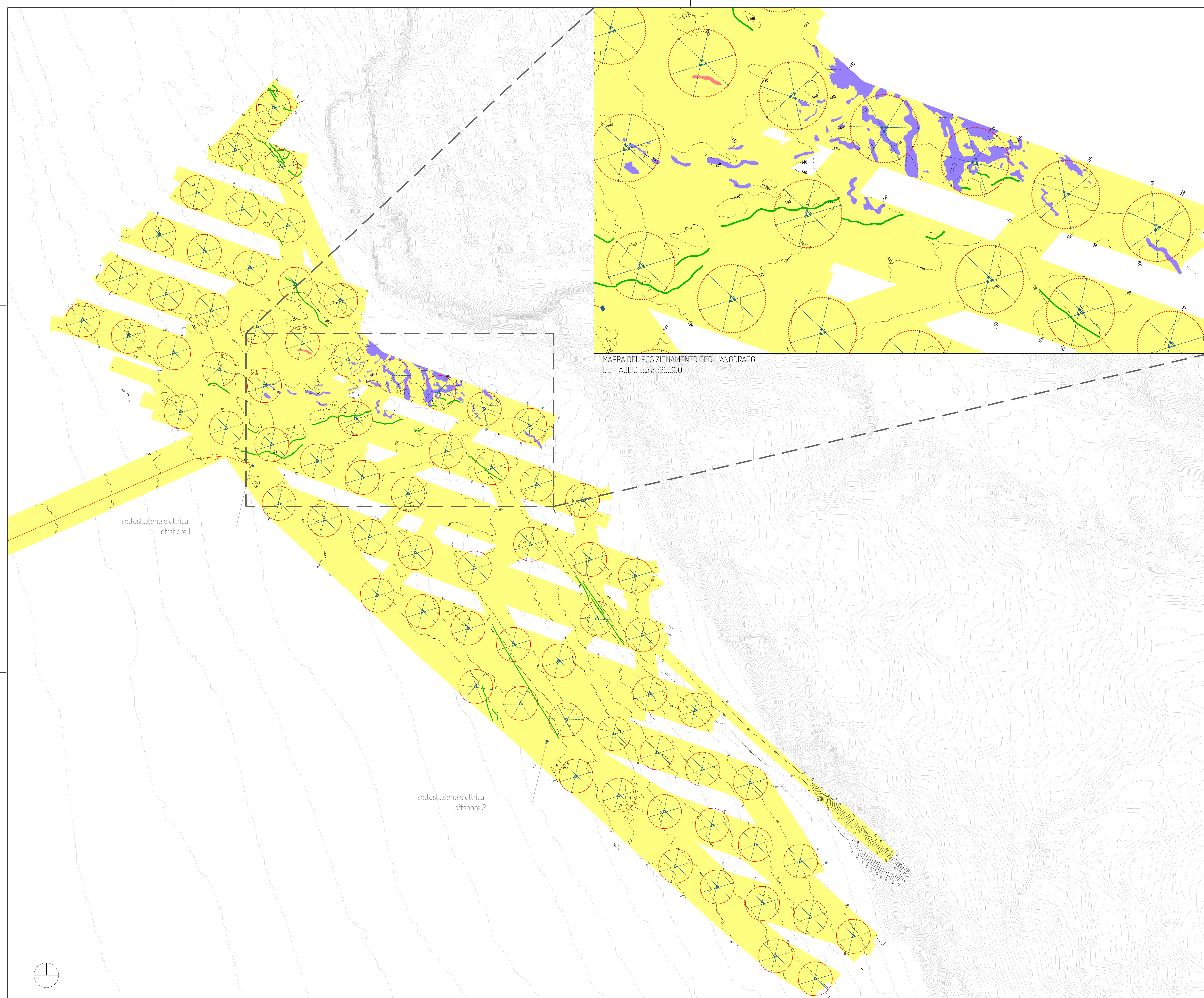
Range di posizionamento degli ancoraggi 500-550 metri dalla fondazione flottante semisommersibile
