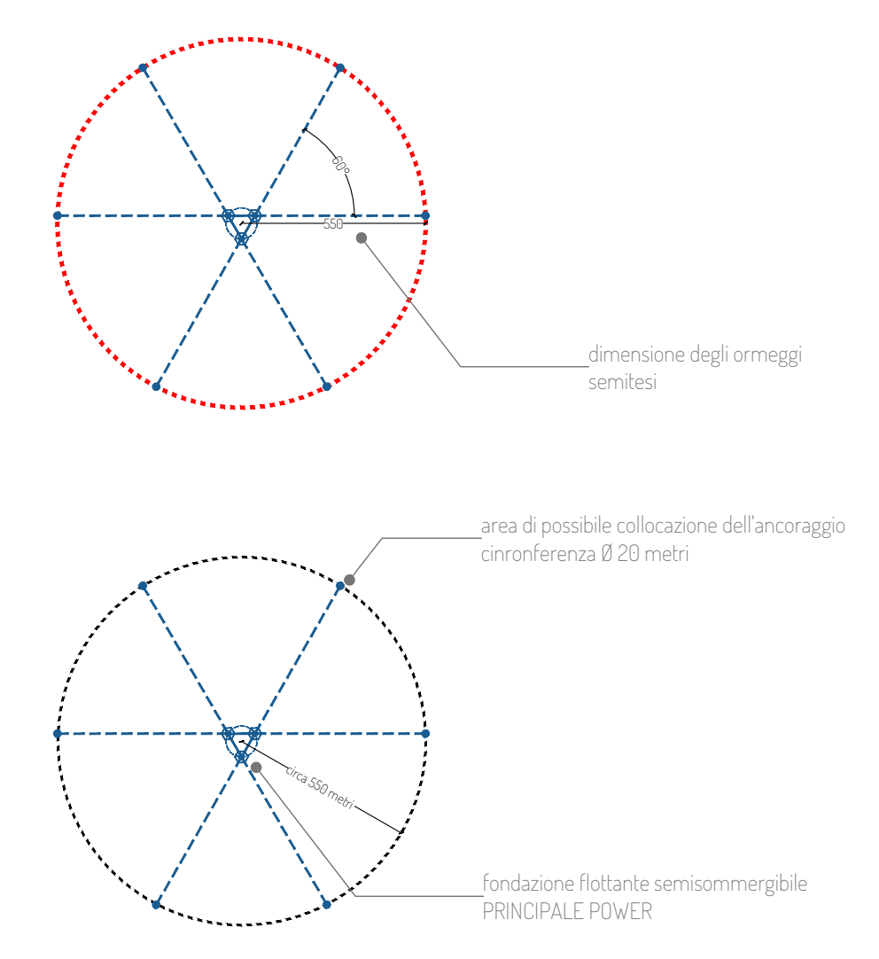
Range di posizionamento degli ancoraggi 500-550 metri dalla fondazione flottante semisommersibile
