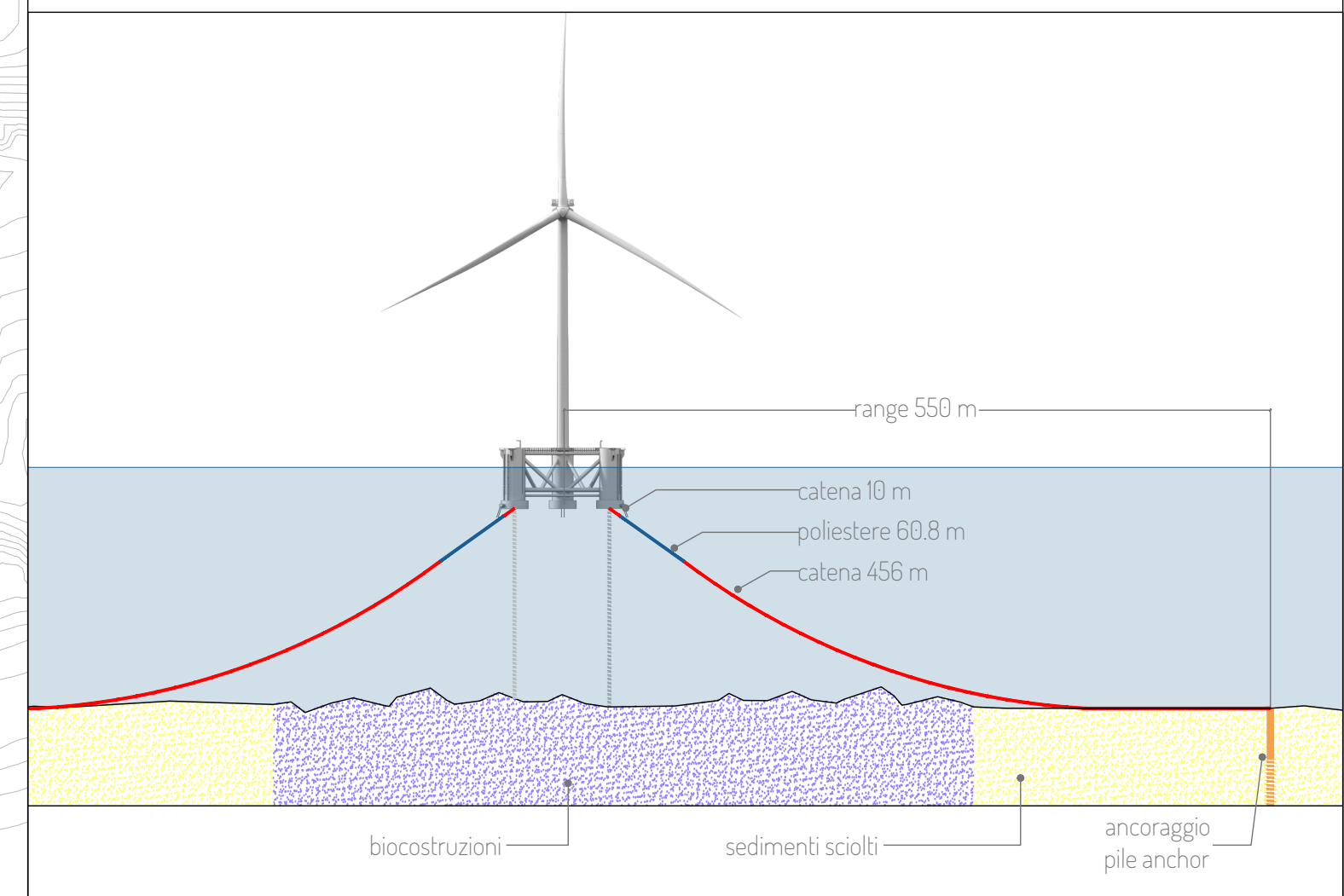
Tipico degli ormeggi semitesi per la fondazione semisommersibile PRINCIPALE POWER
