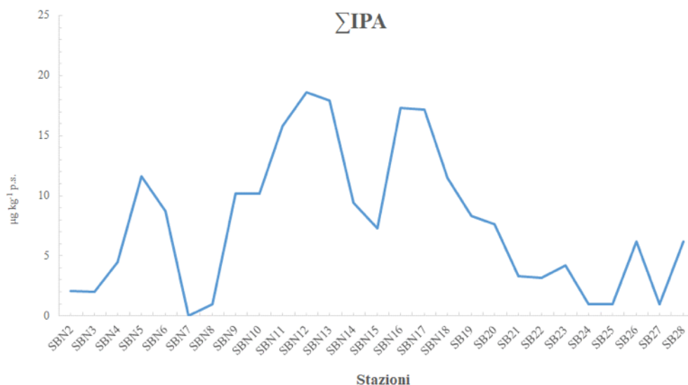
Fig. 4.3.2.3.A – Andamento dei livelli di ΣIPA.
