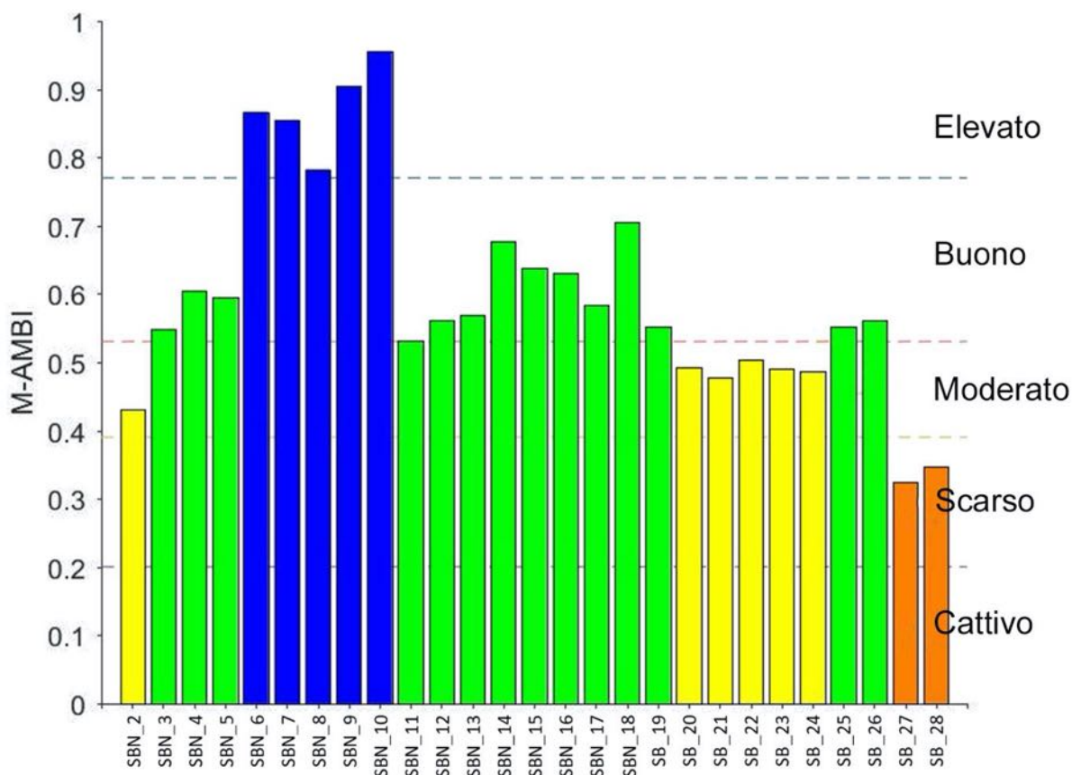
Fig. 5.2.D – Istogramma riportante i valori M-AMBI (che variano da 0 a 1) e la Classificazione di Stato Ecologico calcolati per ciascuna delle stazioni di campionamento effettuate sui fondali interessati dalla futura messa in opera del campo eolico al largo delle città di Bari e Barletta nell’ambito del progetto Barium Bay.
