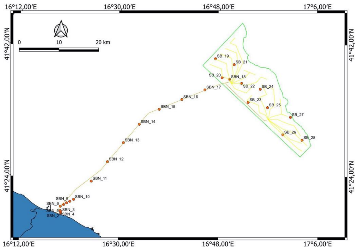
Fig. 5.2.A – Mappa delle stazioni effettuate nell’ambito delle indagini dei fondali interessati dalla messa in opera del futuro parco eolico al largo delle città di Barletta e Bari nell’ambito del progetto Barium Bay.
