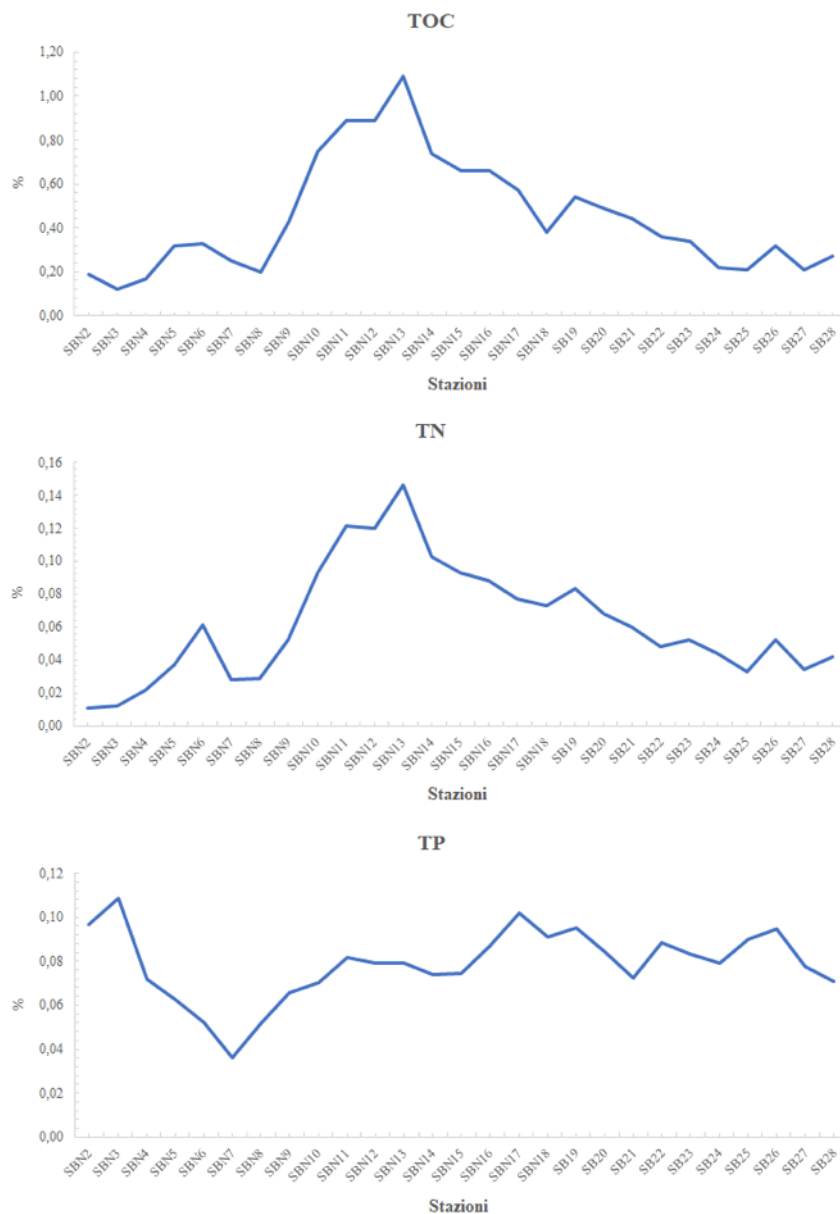
Fig. 4.3.2.1.A – Andamento livelli di TOC, TN e TP.
