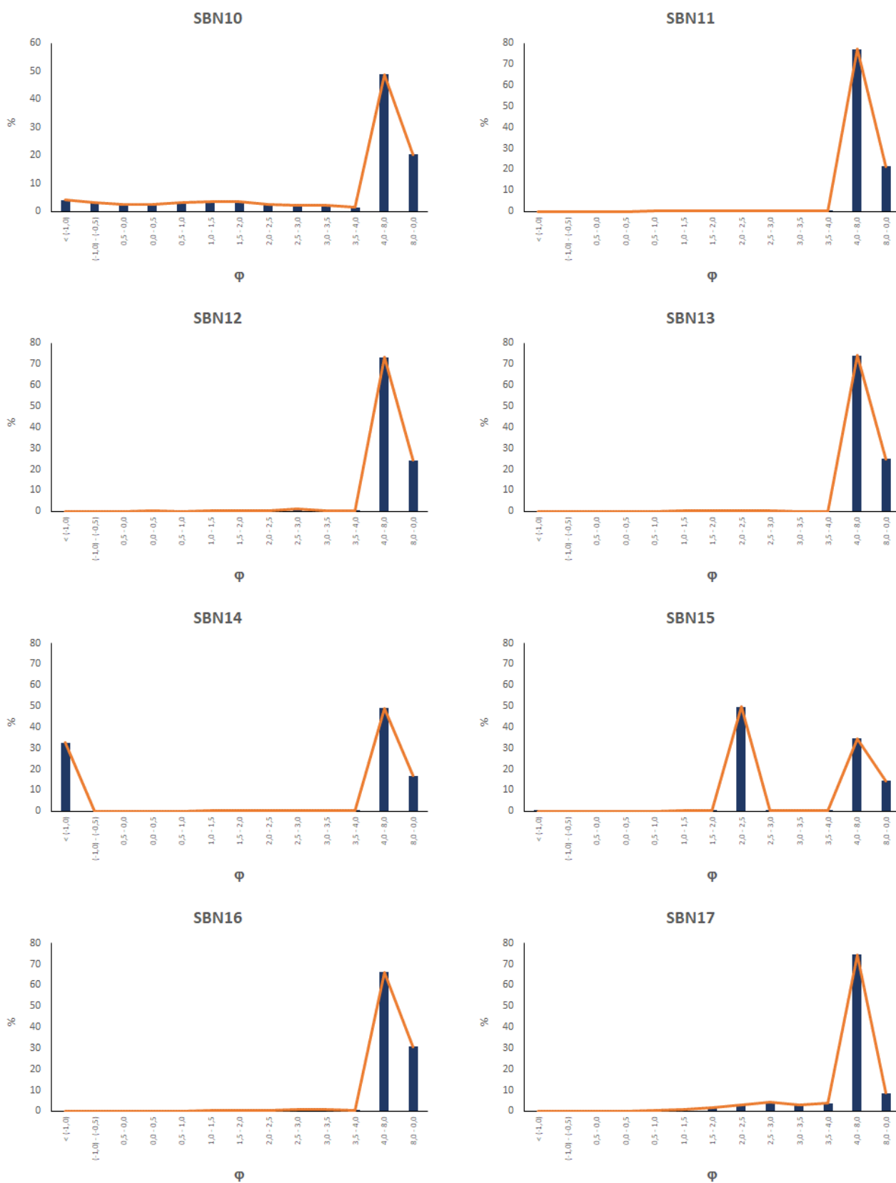
Fig. 4.3.1.B – Distribuzione delle frequenze delle classi granulometriche dei campioni di sedimento delle stazioni da SBN10 a SBN17
