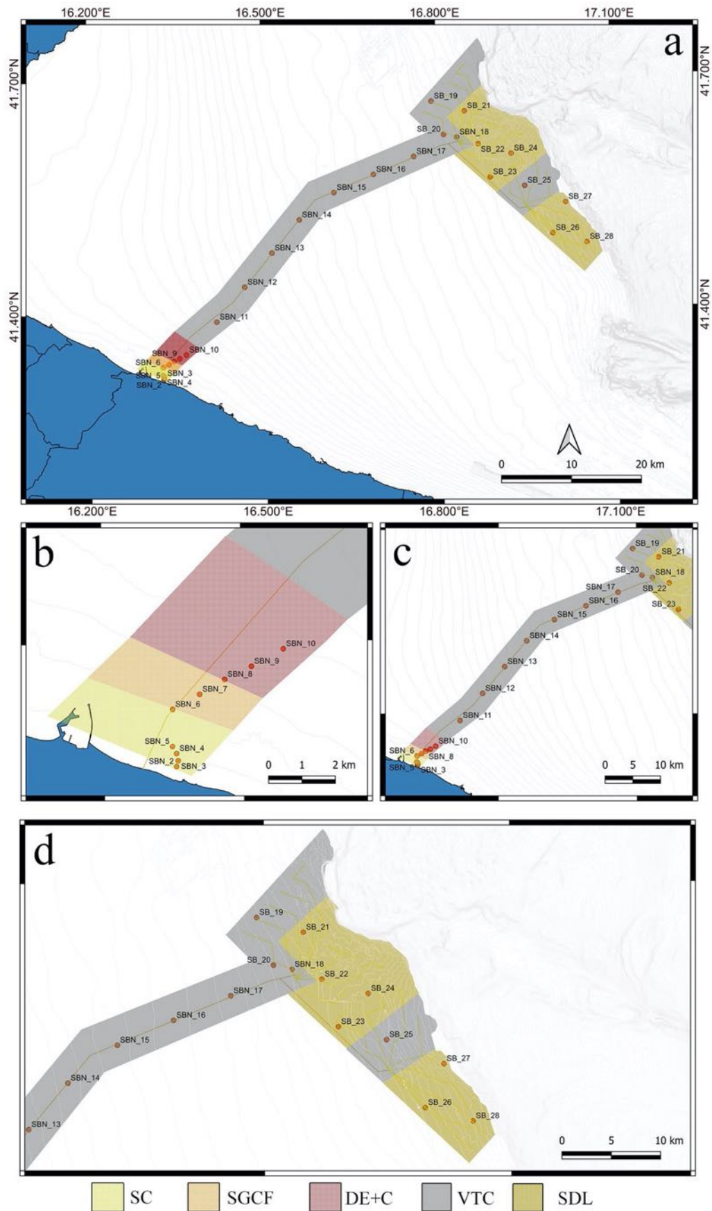
Fig. 6.2.A – Mappa biocenotica dell’area di studio al largo delle città di Barletta e Bari che mostra la distribuzione batimetriche dei diversi tipi di fondale rinvenuti nel corso delle indagini. SC: Sabbie Costiere; SGCF: Sabbie Grossolane con Correnti di Fondo; DE+C: Detritico infangato con nuclei di Coralligeno; VTC: Fanghi Terrigeni Costieri; SDL: Sabbie Detritiche del Largo.
