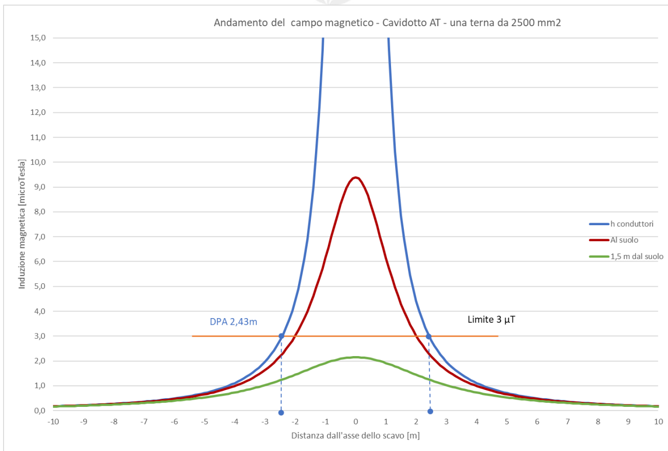
Figura 5 - Andamento del campo magnetico in funzione della distanza dall'asse dei conduttori in forma grafica relativa al cavidotto AT
