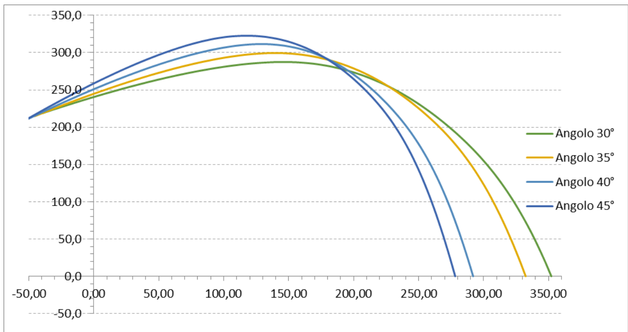
Grafico della traiettoria di un frammento di pala lungo 5 mt
