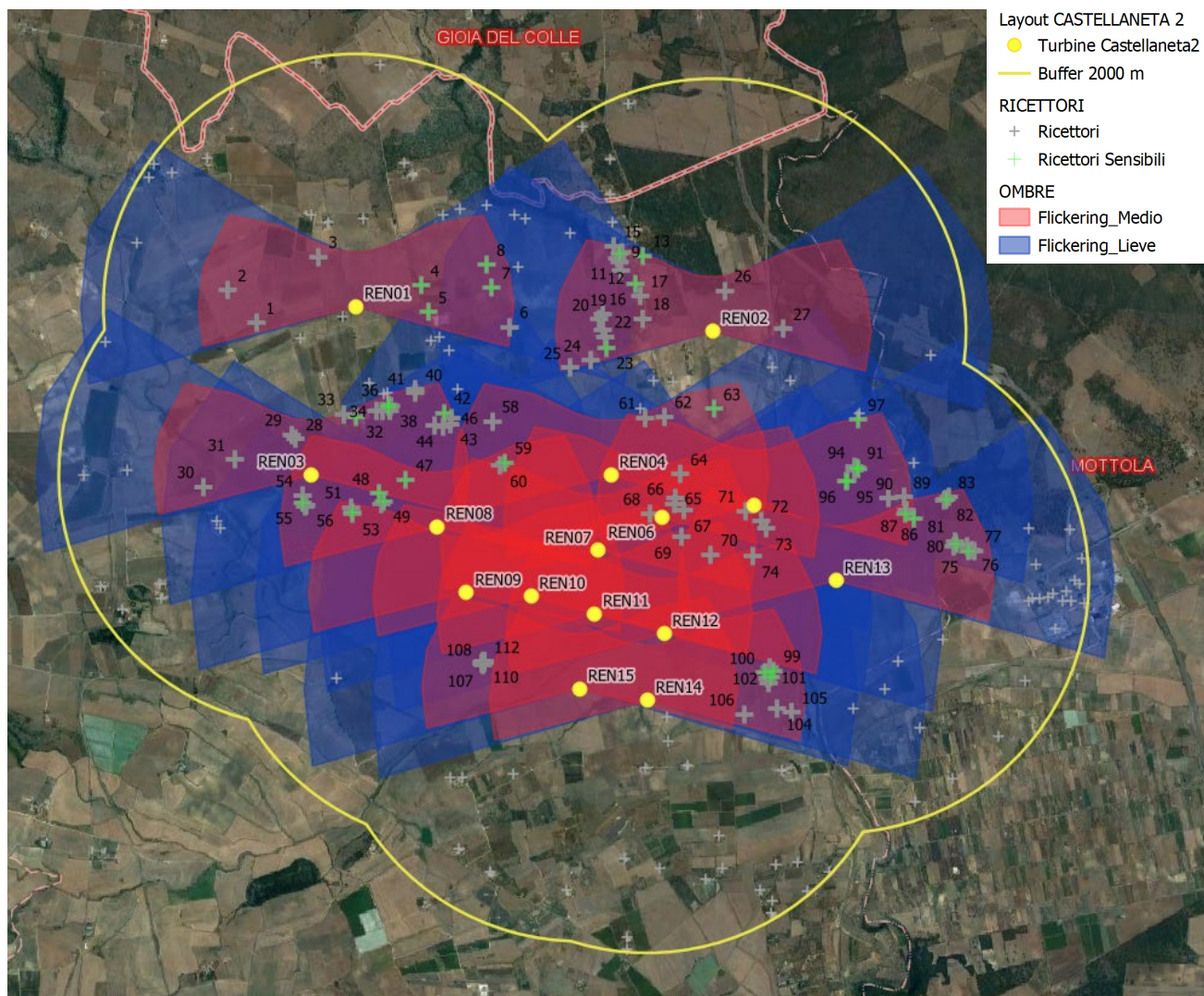
Figura 5-1: Evoluzione dell'ombra nell'area di indagine
