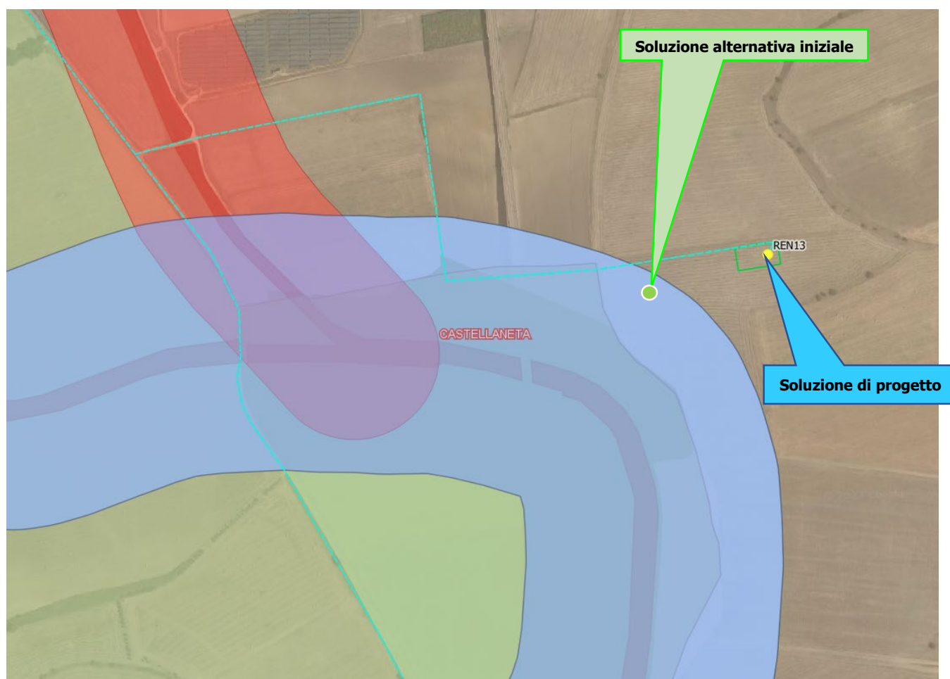
Figura 11-2: Turbina spostata dalla Alternativa 1
