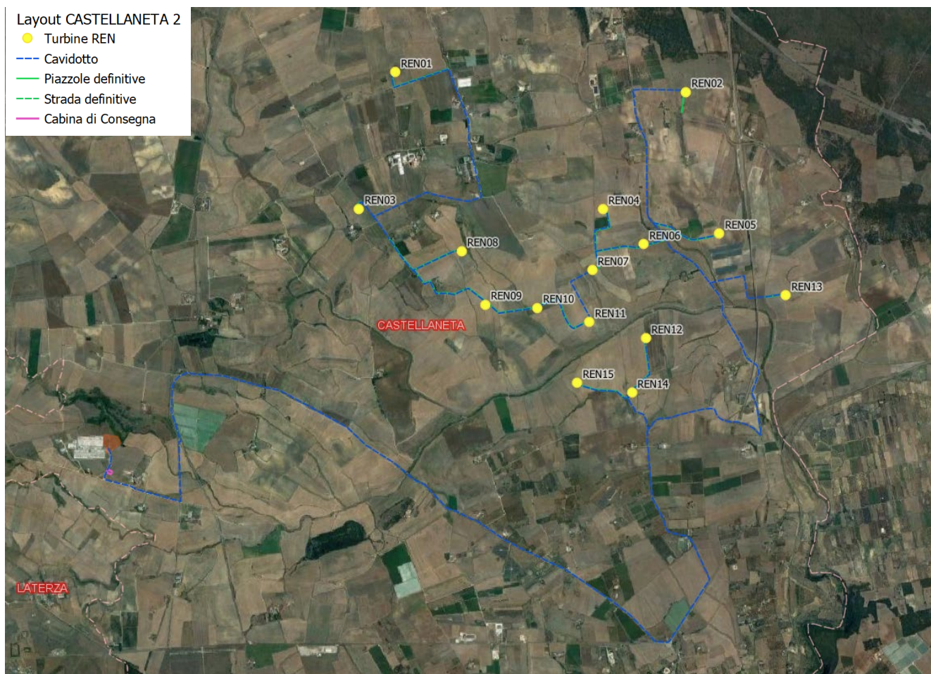
Figura 1-4: Area di intervento: layout di progetto su ortofoto
