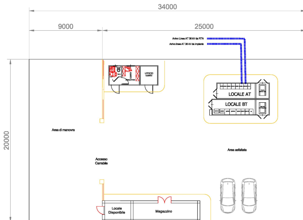
Figura 3-5: Cabina di Consegna utente – schema planimetrico
