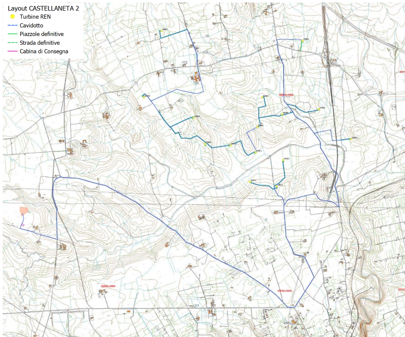
Figura 1-3: Layout del Parco Eolico su base CTR
