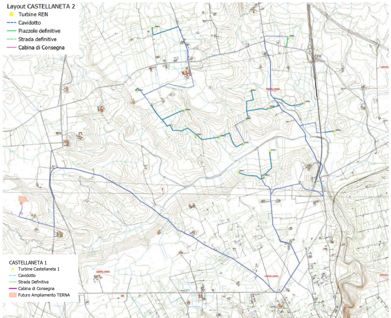
Figura 2-2: Layout del Parco Eolico su base CTR
