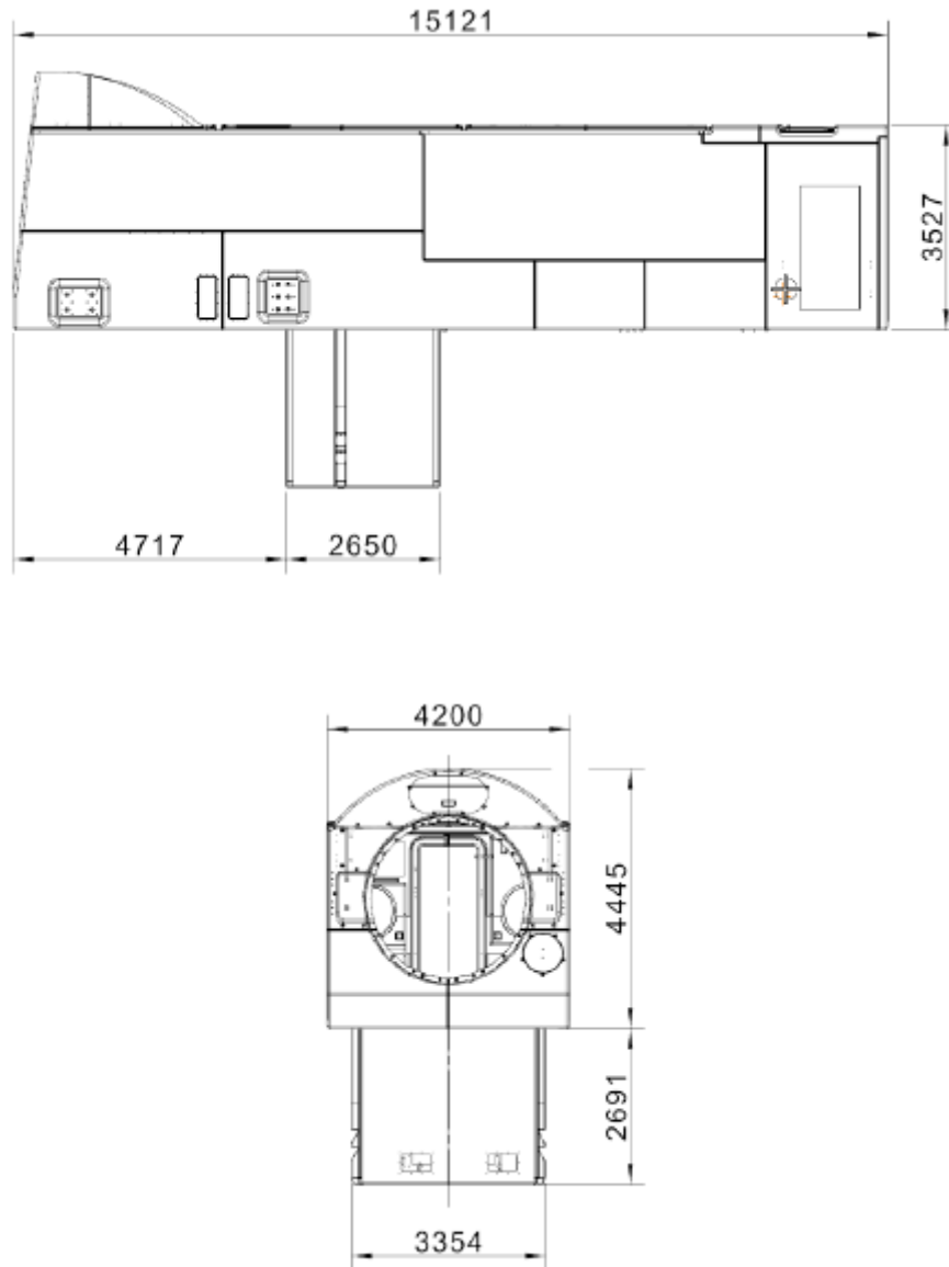
Figura 2-6: Tipico navicella WTG
