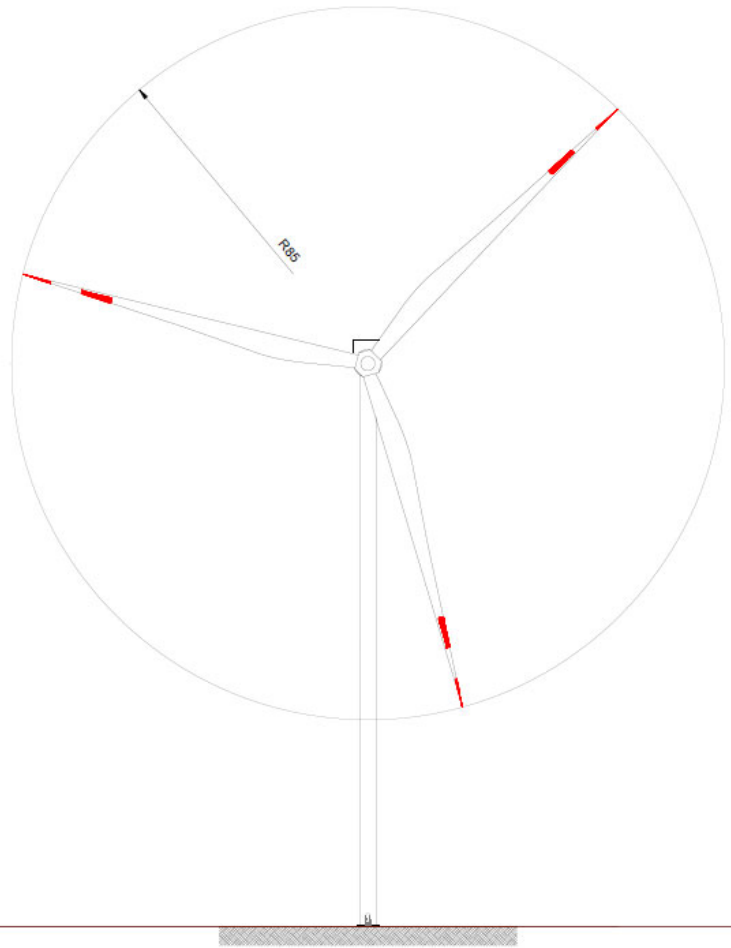
Figura 2-5: Struttura aerogeneratore
