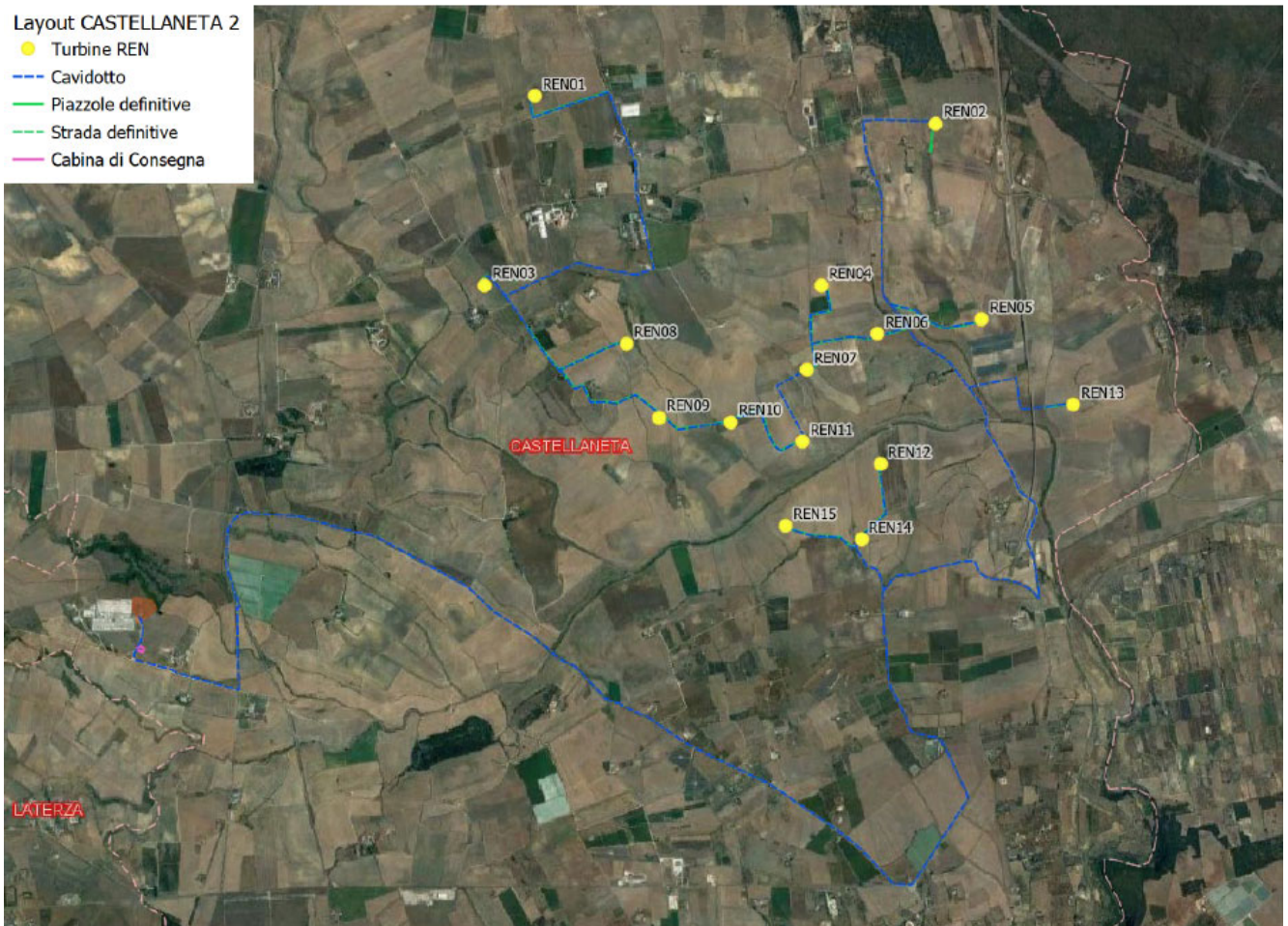
Figura 2-3: Area di intervento: layout di progetto su ortofoto
