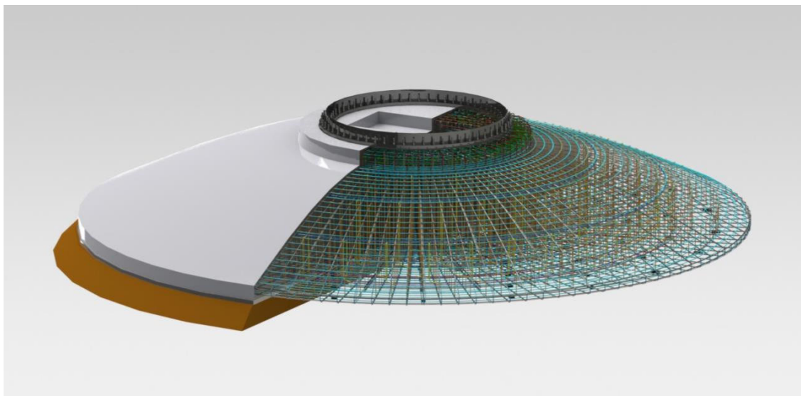
Figura 4: Modello 3d fondazione
