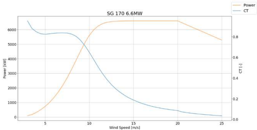
Figura 9. Curva di potenza e di CT(Thrust Coefficient) per l'aerogeneratore SG170 6,6 MW
