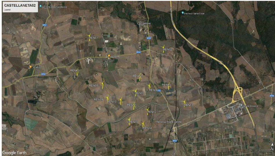
Figura 7. Layout di impianto. Vista in direzione Nord
