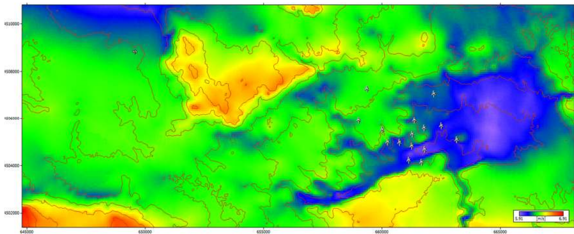
Figura 10. Mappa dell'intensità del vento ad altezza mozzo (115 m)
