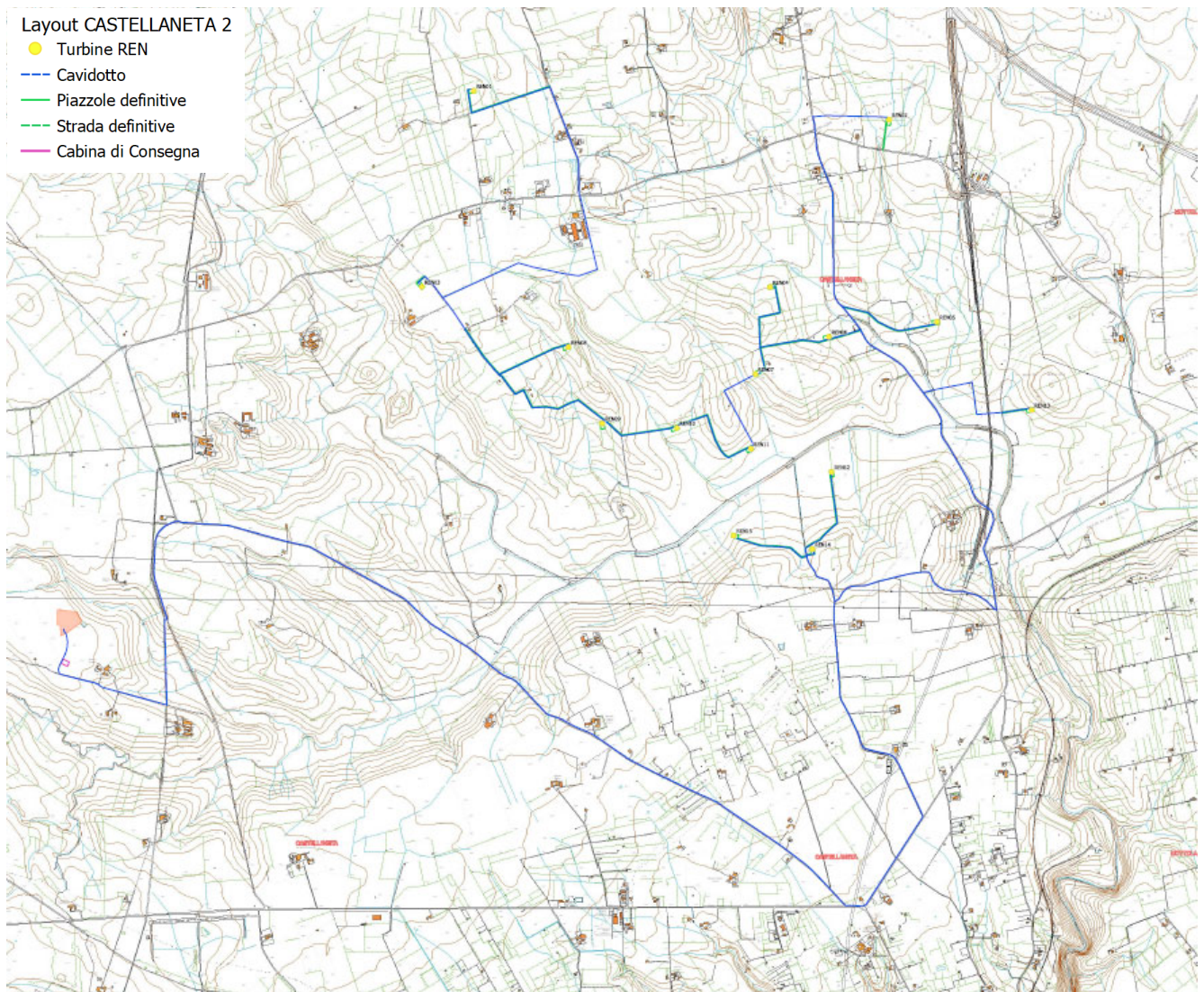
Figura 4-3: Area delle turbine su base CTR
