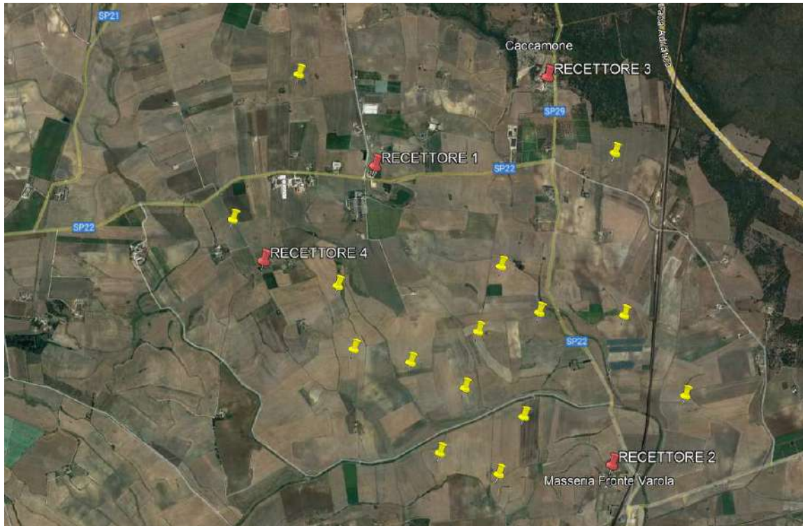
Figura 2: Posizione recettori sensibili
