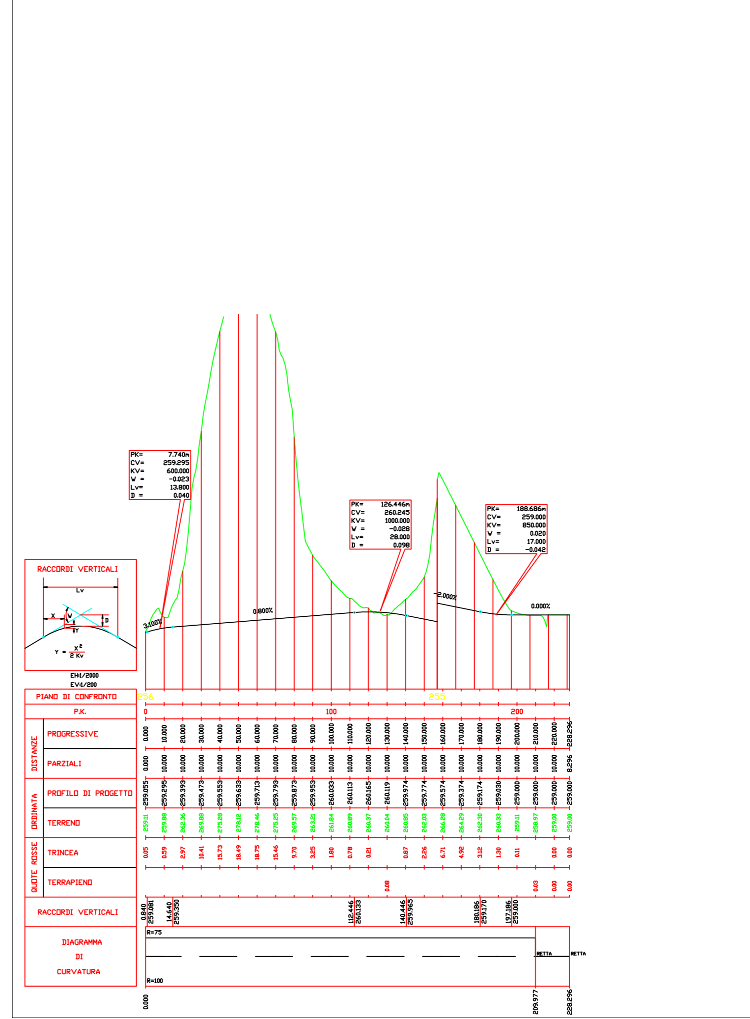
PROFILO FINO AD AEROGENERATORE E7
