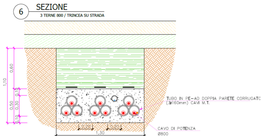
Fig.2 Sezione tipo cavidotto su strada asfaltata
