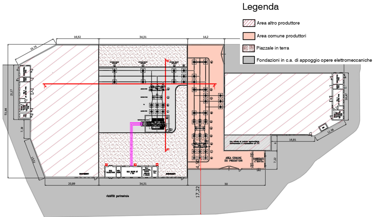
Fig.3 Pianta Stazione elettrica di trasformazione
