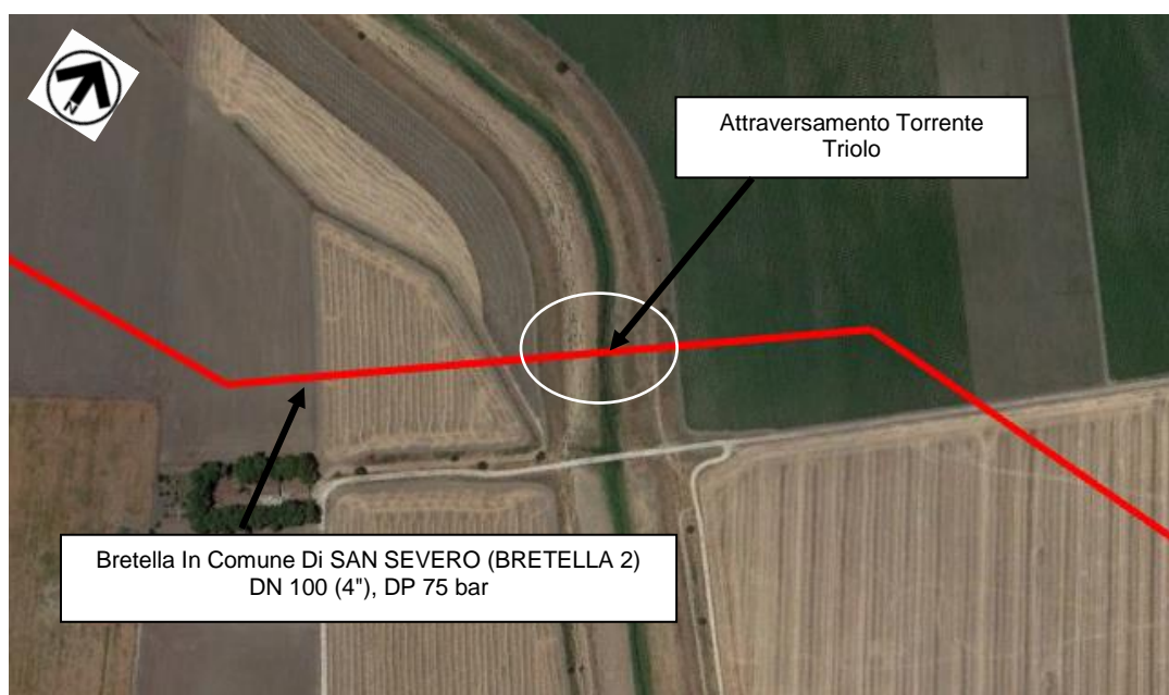
Figura 2.3: Stralcio con foto aerea dell'ubicazione dell'attraversamento del Torrente Triolo con il gasdotto in progetto (in rosso)
