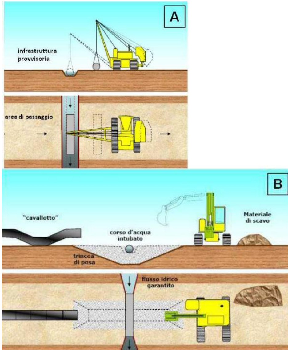
Fig 7.2.1.a. sezione tipo di un by-pass provvisorio del flusso idrico: A. Posa del by-pass per l'incanalamento del corso d'acqua B. Scavo della trincea di posa a cavallo del tratto canalizzato
