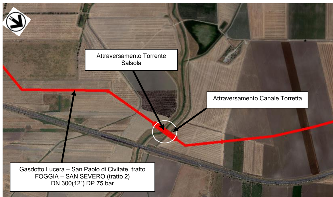
Figura 2.3: Stralcio con foto aerea dell'ubicazione dell'attraversamento del Canale Torretta con il metanodotto in progetto (in rosso)
