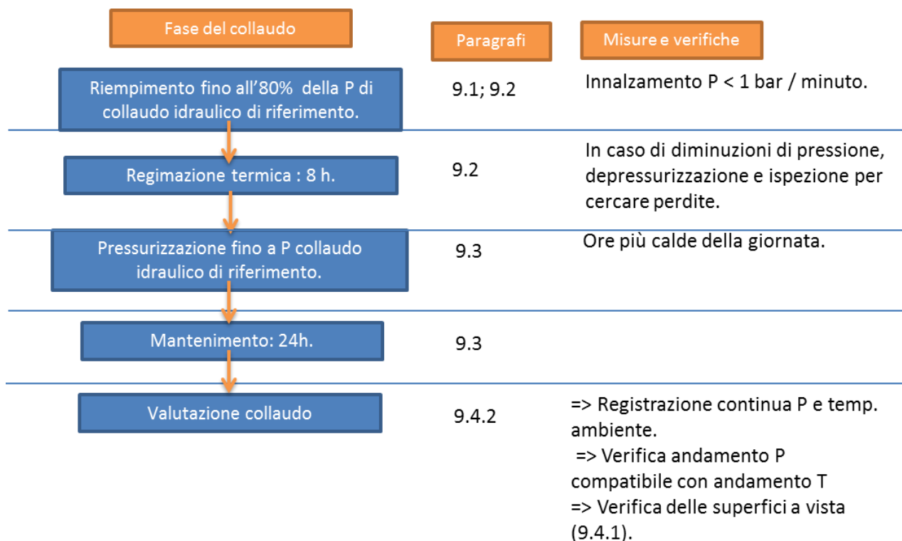
Figura 4 - Schema generale per il collaudo di impianti di grandi dimensioni
