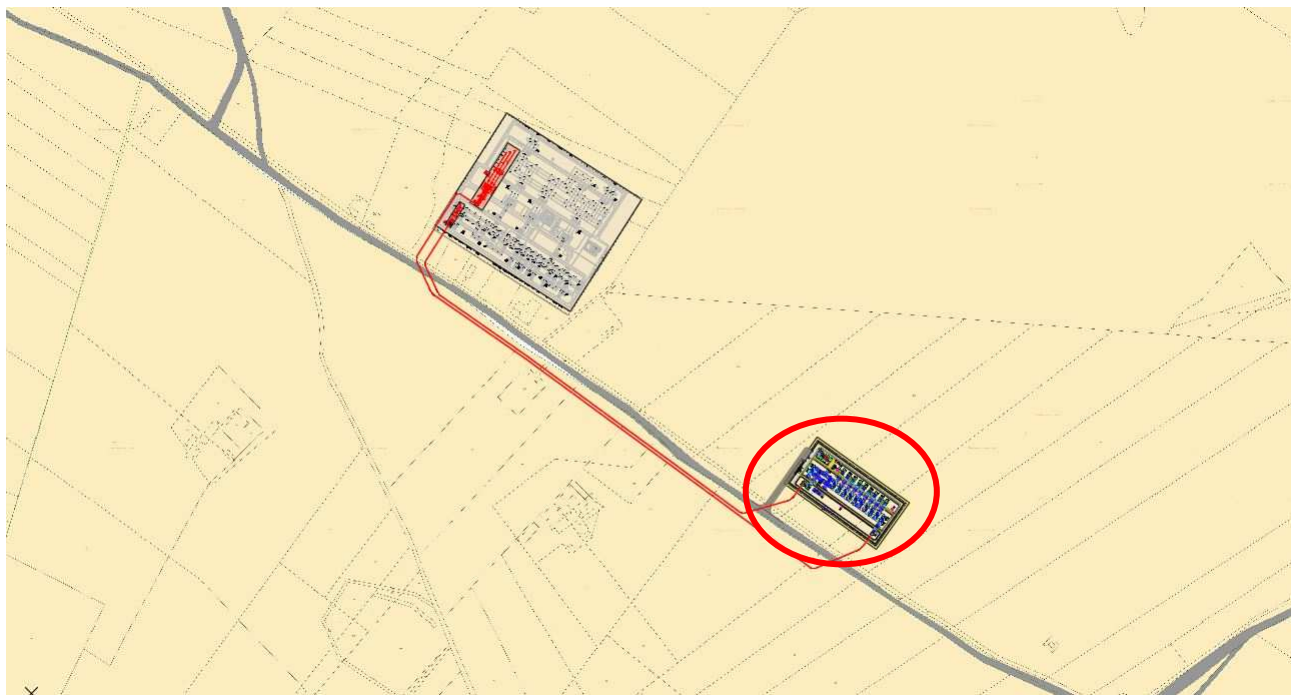
Figura 4 – individuazione dell’area destinata al nuovo satellite della SE RTN di Genzano (PZ) su catastale
