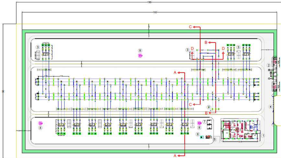
Figura 10 – planimetria elettromeccanica
