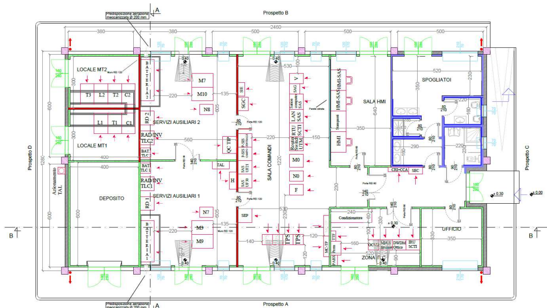
Figura 11 – planimetria edificio comandi
