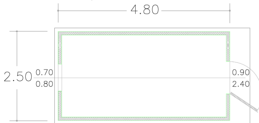
Figura 13 – planimetria chioschi
