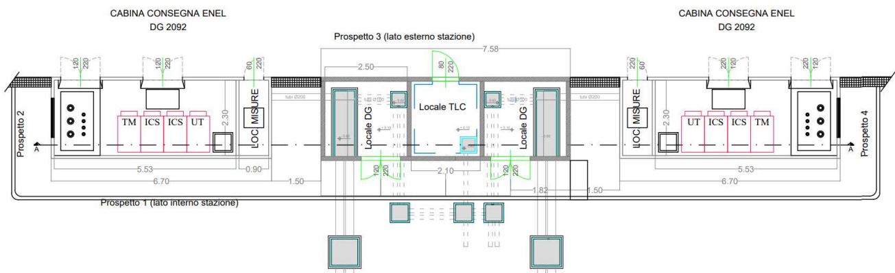
Figura 12 – planimetria edifici consegna MT e TLC
