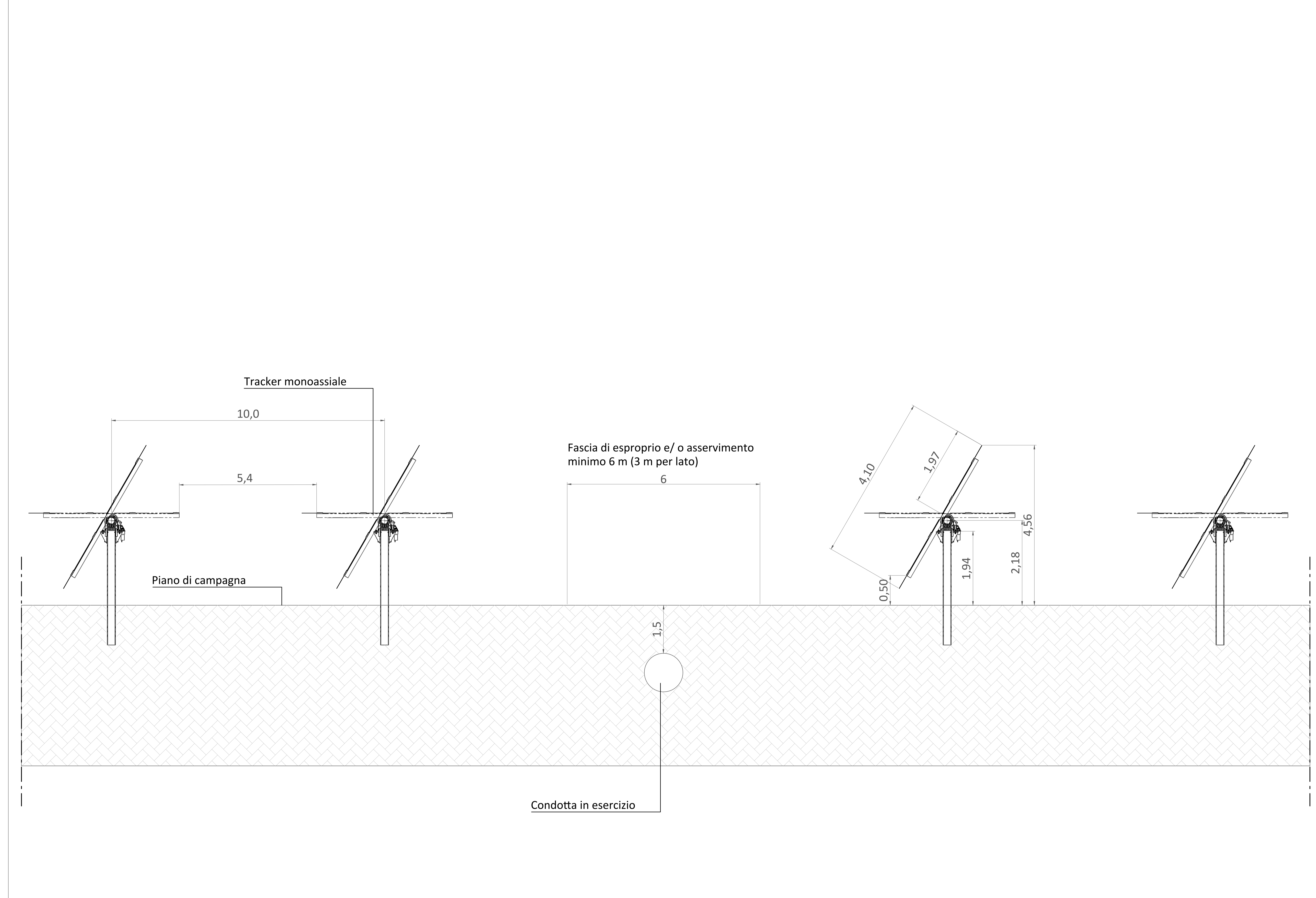
SEZIONE A-A - Scala 1:50
