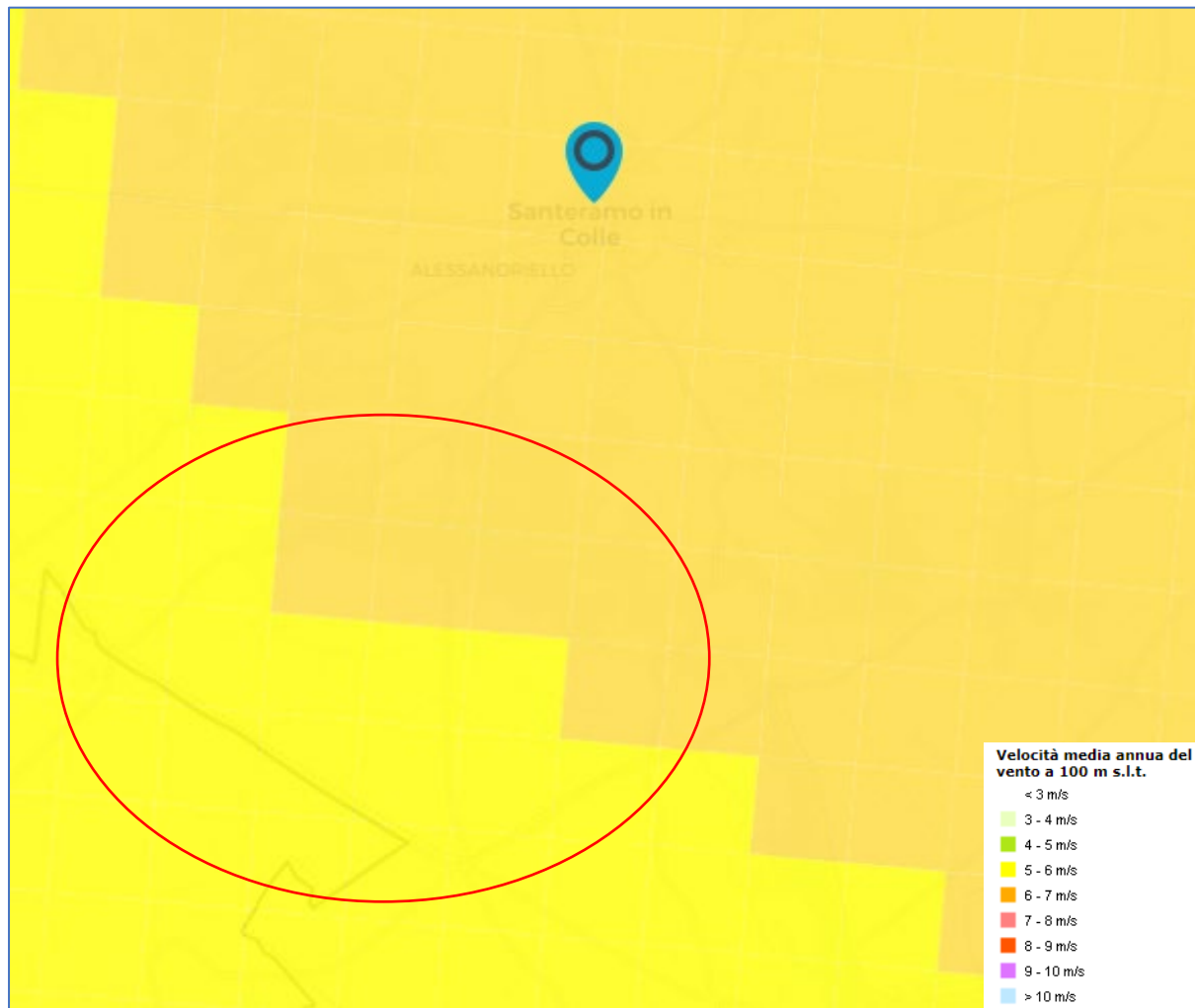
Figura 3 - velocità del vento a 100 m s.l.t.
