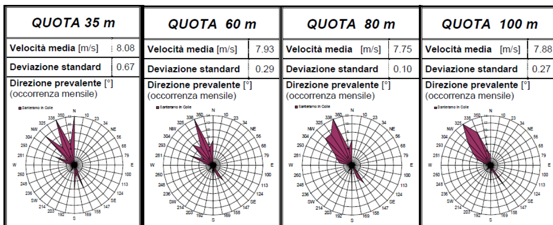
Figura 2 - Velocità media annua del vento fino a 100 m s.l.m.m - fonte Atlante Eolico
