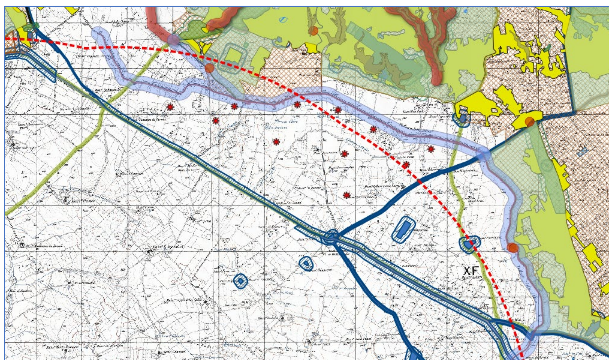
Figura 3 - Ipotesi Layout a 11 aerogeneratori - analisi vincolistica
