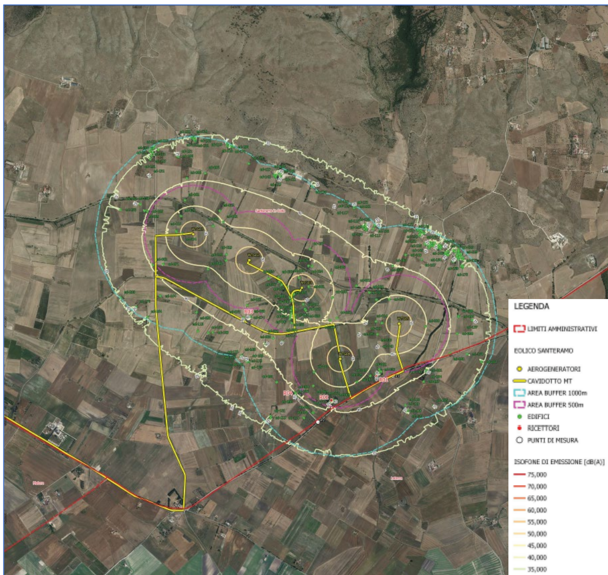
Figura 4 - Inquadramento dei recettori considerati nella stima previsionale di emissione delle turbine di progetto (WTG) proposta nella versione ortofotografica satellitare estratta da Google Earth.
